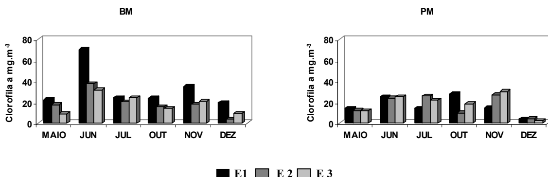
Figura 17. Variação sazonal da biomassa fitoplactônica - clorofila a ( \text{mg.m}^{-3} ) no estuário do rio Formoso, Pernambuco, durante a baixa-mar e a preamar no período chuvoso (maio, jun., jul/02) e de estiagem (out., nov. e dez/02). E = Estação; BM = Baixa-mar; PM = Preamar.
