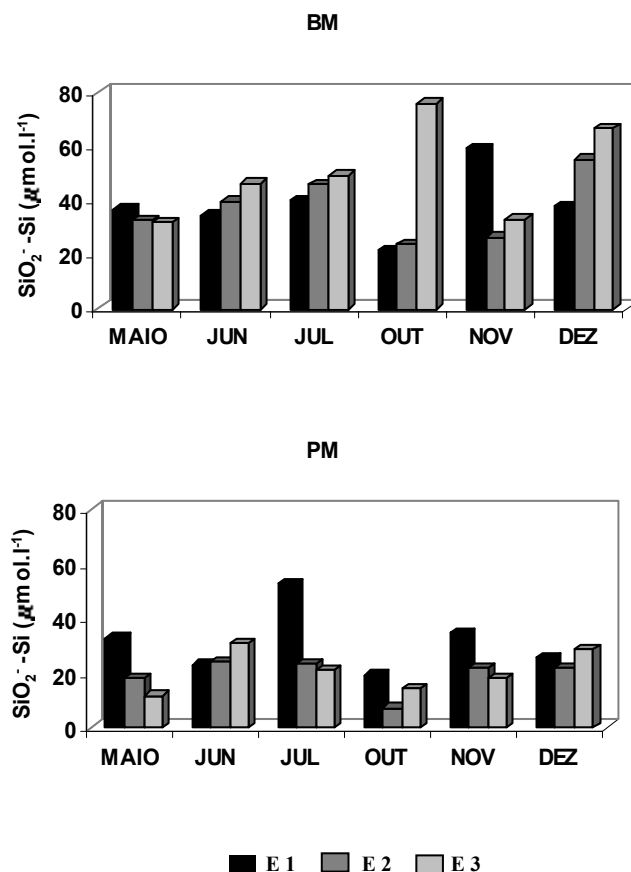
Figura 16. Variação sazonal do silicato – Si ( \mu\text{mol.l}^{-1} ), no estuário do rio Formoso, Pernambuco, durante a baixa-mar e a preamar no período chuvoso (maio, jun., jul/02) e de estiagem (out., nov. e dez/02). E = Estação; BM = Baixa-mar; PM = Preamar.
