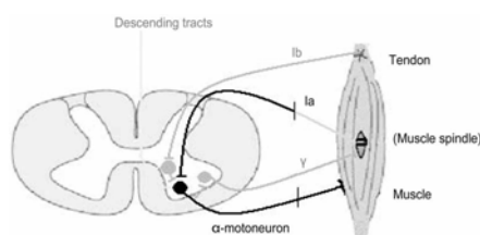
Figura 6. Representação esquemática da via neural do reflexo H (linha preta) (VOERMAN et al., 2005).
