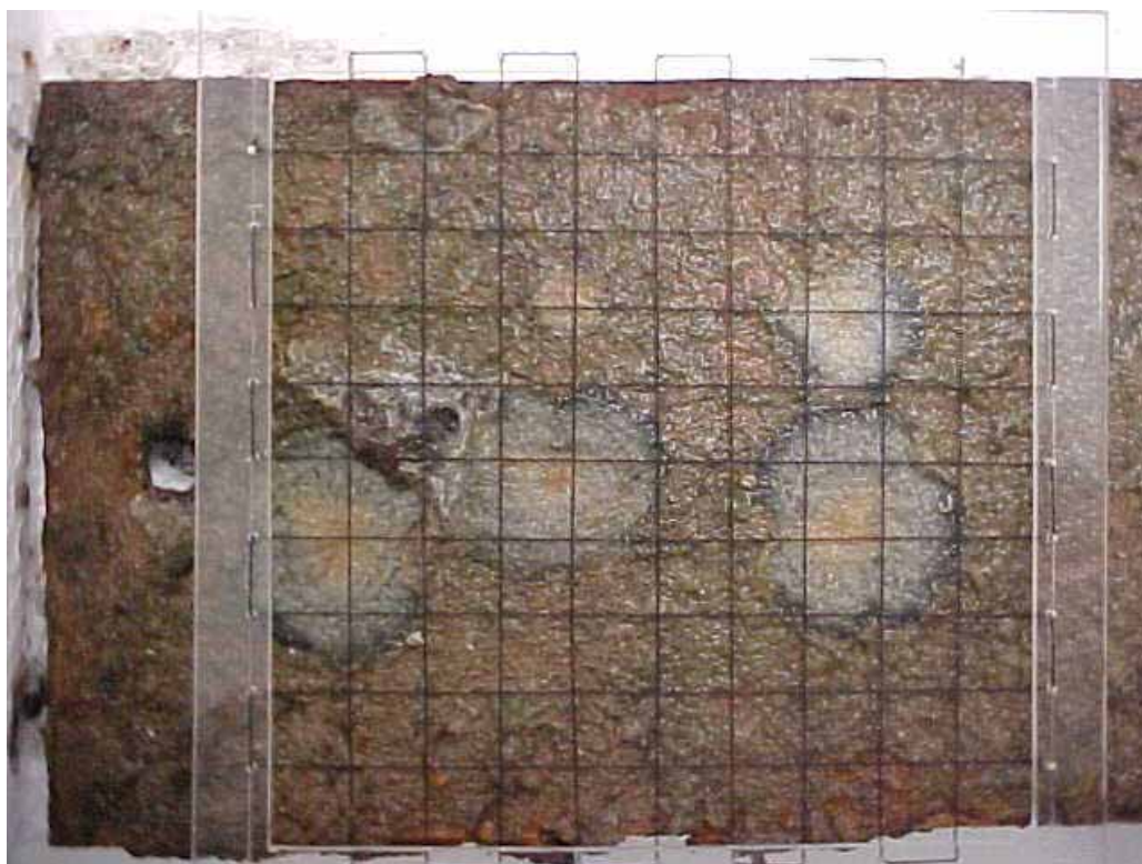
Figura 07: Exemplo Placa controle, mostrando área de recobrimento de 10 cm x 10 cm, com placa reticulada de nylon com moldura de acrílico, nas mesmas dimensões da área estimada para estudo.
