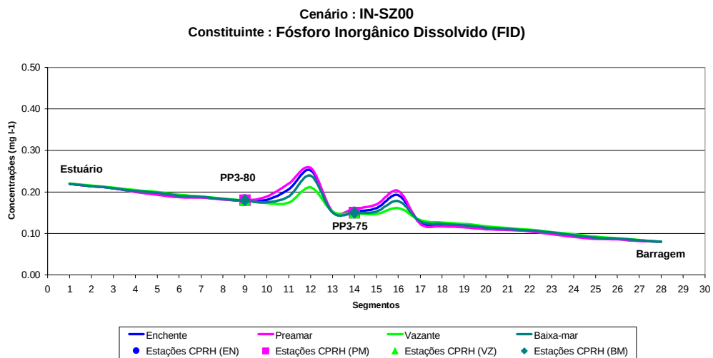
Figuras 7.13a a 7.13c. Calibração do Modelo de QA para OD, DBO 5,20 e FID. Cenário: IN-SZ00
