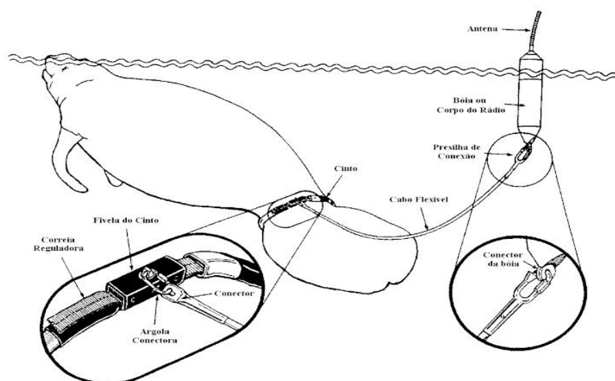
Figura 13. Esquema dos equipamentos e acessórios de radio telemetria utilizados para monitoramento dos peixes-bois reintroduzidos no litoral nordeste do Brasil. (Fonte: Reid et al , 1995.)
