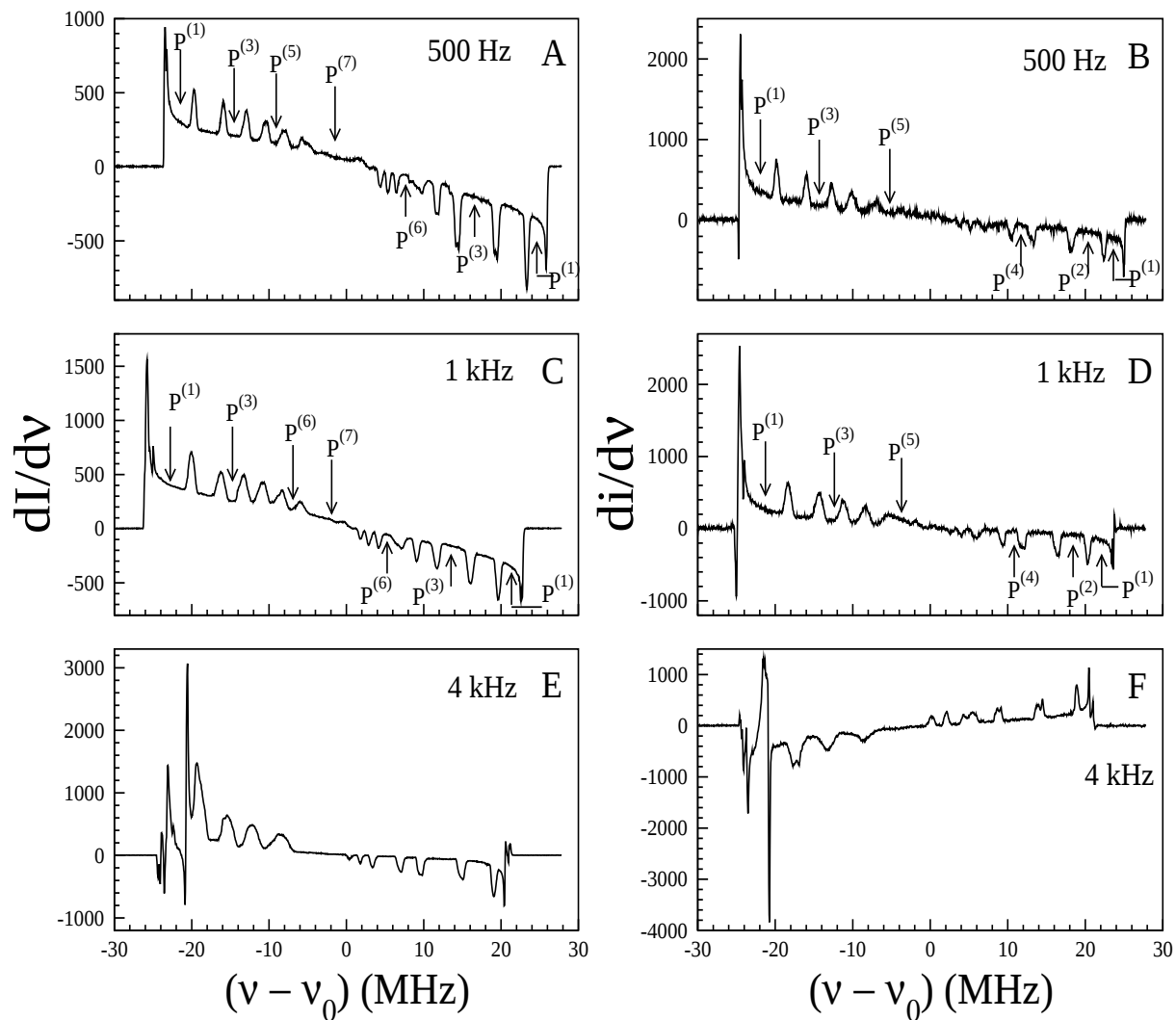
Figura 3.9: Bifurcações na dinâmica manifestadas na média da intensidade ( \frac{dI}{d\nu} ) e da corrente ( \frac{di}{d\nu} ) do laser.
