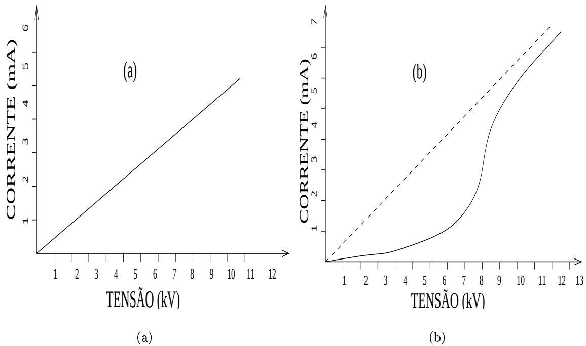
Figura 2.3: Esquema do comportamento da corrente em função da tensão aplicada: (a) em um resistor ôhmico, (b) na ampola de gás com resistor em serie.
