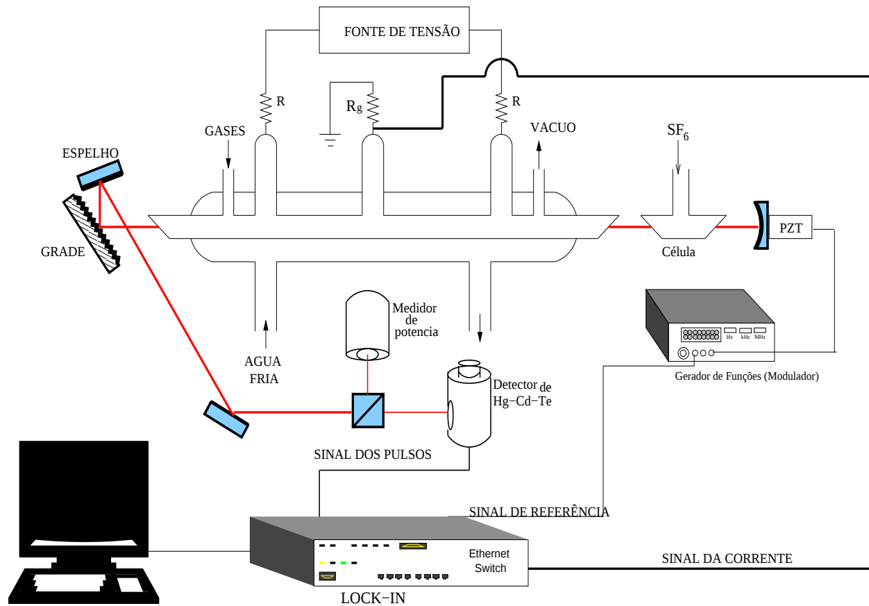
Figura 3.1: Esquema do montagem experimental para estudar o efeito fotogalvânico no laser de CO_2 , operando no modo Q-switching.
