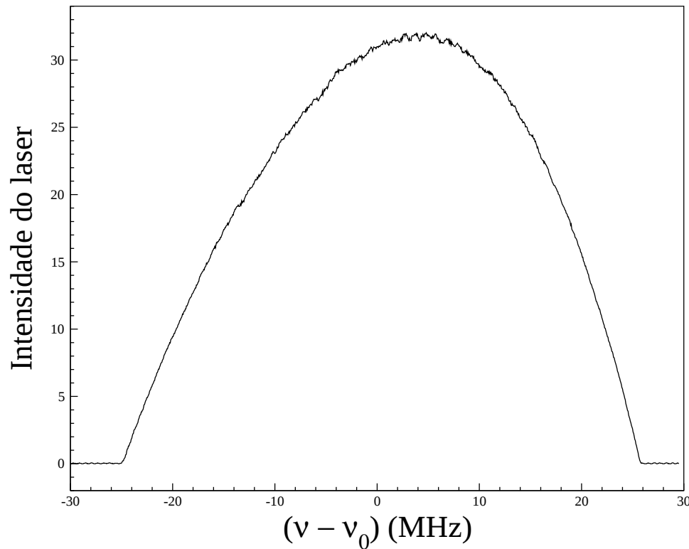
Figura 3.2: Intensidade do laser de \text{CO}_2 em operação contínua, com chopper de referência no Lock-in. Na ordenada temos uma intensidade máxima de 3 Watts, medida no detetor de potência. O valor de pico ocorre em \nu_0 é 28359773,8165 MHz correspondente a linha espectral P(18) da banda de 10.6 \mu\text{m} [Pag.22 da ref. [2]].
