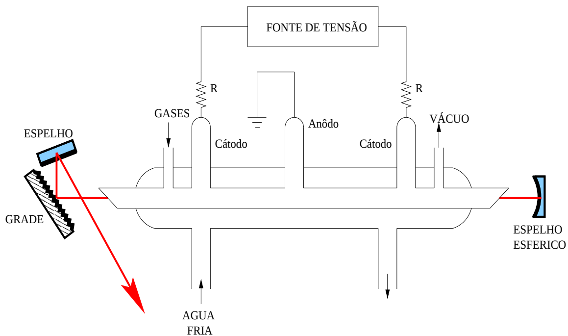
Figura 1.1: Laser de \text{CO}_2 com espelho esférico e grade de difração. O gás é uma mistura de \text{CO}_2 , \text{N}_2 e He.
