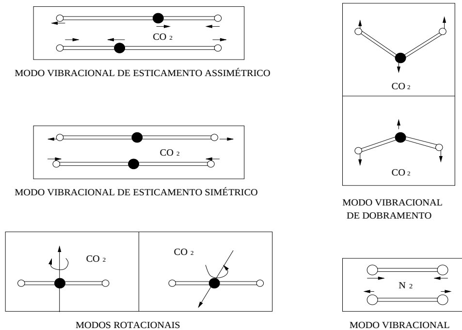
Figura 1.3: Esquema das moléculas de CO 2 e N 2 com indicação dos modos vibracionais e rotacionais [15, ?].
