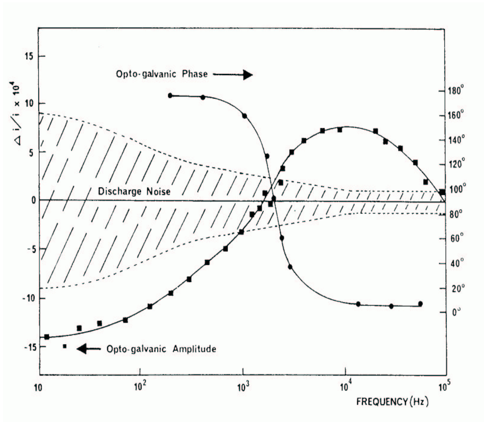
Figura 2.8: Fase do efeito fotogalvânico com respeito a fase de modulação da potência de um laser de CO 2
