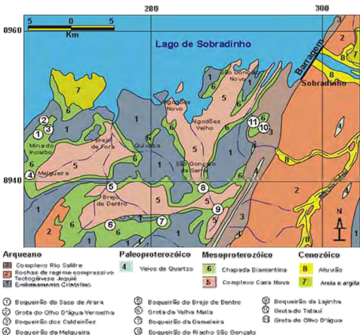
Figura 3 – Esboço geológico da unidade de pesquisa
