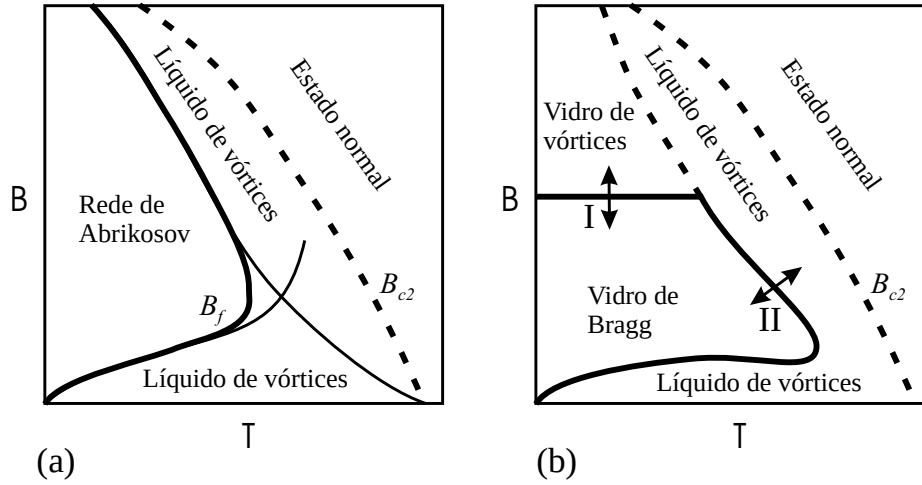
Figura 2.6: Diagramas de fase B-T para um sistema de vórtices em cristais perfeitos (a) e com desordem (b). As linhas contínuas indicam transições de fase abruptas, de primeira ordem, enquanto que as linhas intermitentes indicam transições contínuas. As linhas contínuas finas em (a) correspondem às curvas B_f(T) nos limites \mu_0 H_{c1} \ll B \ll \mu_0 H_{c2} e B \lesssim \mu_0 H_{c1} estudados acima pelo modelo cage . As setas em (b) indicam fusão induzida por desordem (I) e fusão induzida termicamente (II).
