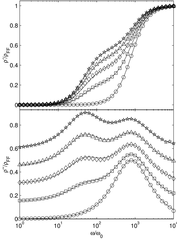
Figura 4.8: Partes real \rho' (painel superior) e imaginária \rho'' (painel inferior) da resposta ac para um potencial periódico de ancoragem com periodicidade a_p = \Lambda/4 e força restauradora de ancoragem \alpha_p = 8\pi\epsilon/a_p^2 . Os símbolos são os resultados da simulação de dinâmica molecular para n = B/B_\Phi = 1 ( \circ ), 1.25 ( \square ), 1.5 ( \diamond ), 1.75 ( \triangle ) e 2 ( \star ). As linhas cheias correspondem ao resultado analítico do modelo de duas espécies [Eq. 4.25]. Nenhum parâmetro de ajuste foi usado. Os dados de \rho'' foram deslocados verticalmente para melhor visualização.
