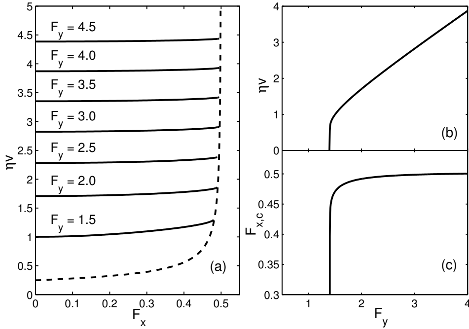
Figura 5.6: Resultados do modelo cage dinâmico para movimento comensurável ao longo da direção [0,1] e a T = 0 , mostrando a dependência da velocidade longitudinal, v , com as componentes transversal F_x (a) e longitudinal F_y (b) da força motriz. A linha intermitente corresponde à força crítica transversal, a partir da qual a fase comensurável se torna instável. (c) F_{x,c} em função de F_y . As forças estão normalizadas pela força máxima de ancoragem F_{max} = 8\pi|U_1|/a_p .
