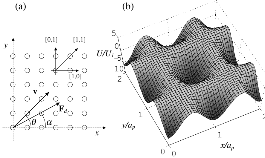
Figura 5.2: (a) Rede quadrada de armadilhas. As direções de maior simetria estão indicadas. Também é indicado o sistema de coordenada e são definidas as variáveis angulares da velocidade do centro de massa \mathbf{v} e da força motriz \mathbf{F}_d . (b) Potencial de ancoragem gerado pela Eq. (5.35) com U_2 = U_1/2 .
