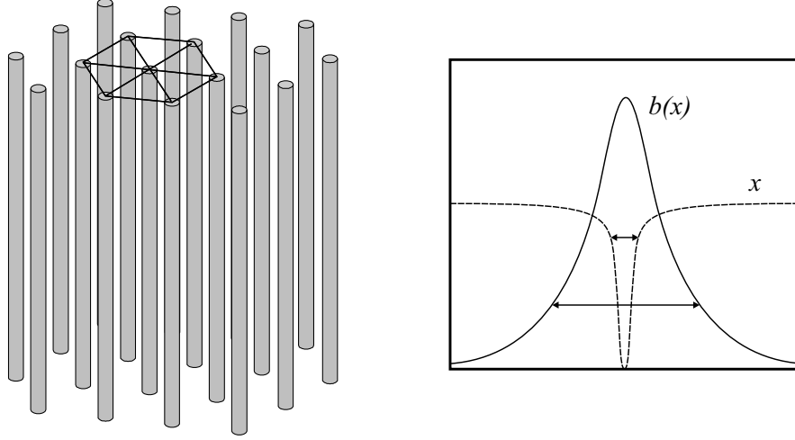
Figura 2.2: Esquerda: Representação da rede triangular de Abrikosov em seu estado não perturbado ( T = 0 e sistema homogêneo). Direita: estrutura de um vórtice isolado, mostrando o comportamento espacial do parâmetro de ordem e da indução magnética local nas proximidades do núcleo e os comprimentos característicos do vórtice.
