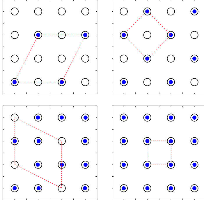
Figura 4.1: Configurações de equilíbrio da rede de vórtices no potencial de ancoragem dado pela Eq. (4.2) para números de ocupação n = 0, 25, 0,5, 0,75 e 1 , da esquerda para a direita e de cima para baixo. Os círculos menores (pretos) representam os vórtices e os grandes (brancos) representam os centros de ancoragem. Os polígonos tracejados correspondem às respectivas células unitárias. As configurações foram obtidas pelo procedimento de annealing simulado descrito no texto, usando a_p = \Lambda/4 , r_p = 0,1a_p e \alpha_p = 8\pi\epsilon/a_p^2 .
