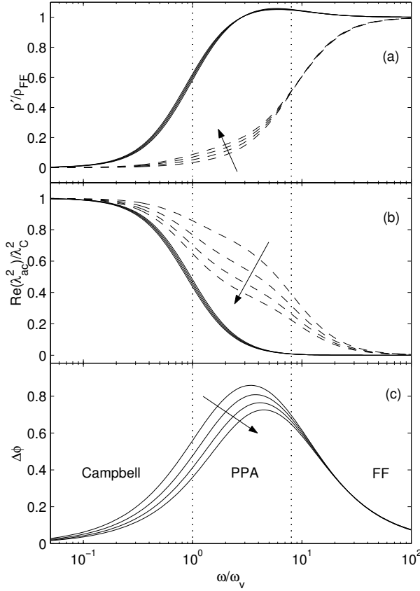
Figura 4.7: Espectro de frequência da resistividade ac e do comprimento de penetração para campos entre o primeiro e segundo campos de matching , com n = 1, 1\frac{1}{8}, 1\frac{1}{4}, \dots, 2 . A seta indica o sentido crescente de n . Adotamos como escala de frequência a frequência de acoplamento vórtice-vórtice, \omega_v . A frequência de ancoragem escolhida foi \omega_p = 8\omega_v .
