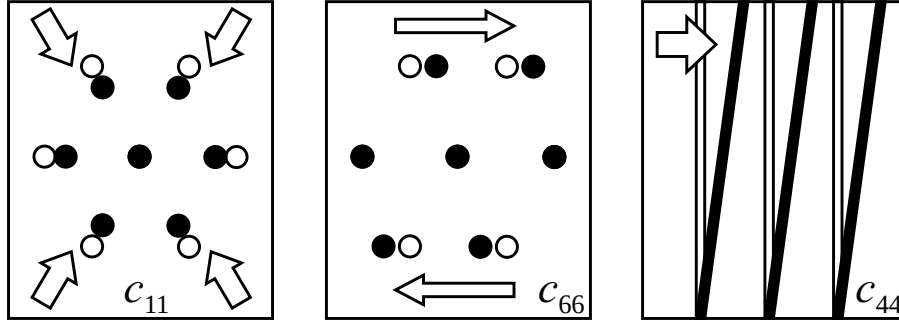
Figura 2.4: Três deformações diferentes na rede de vórtices correspondendo aos módulos elásticos de, da esquerda para a direita, compressão ( c_{11} ), cisalhamento ( c_{66} ) e entortamento ( c_{44} ).
