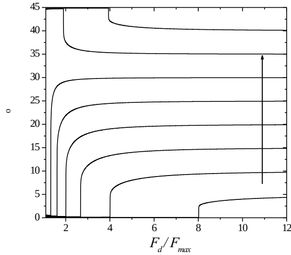
Figura 5.4: Direção do movimento \theta em função da intensidade da força motriz F_L para direções de \mathbf{F}_L no intervalo 5^\circ \leq \alpha \leq 45^\circ em incrementos de 5^\circ . A seta indica o sentido crescente de \alpha .
