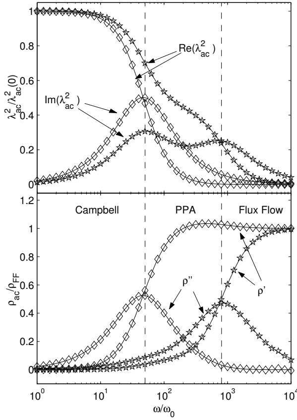
Figura 4.10: Contribuições parciais da rede de vórtices ancorados ( \star ) e da rede de vórtices intersticiais ( \diamond ) para o comprimento de penetração ac (em cima) e a resistividade ac (em baixo) para B = 2B_\Phi . Os comprimentos de penetração estão normalizados pelos respectivos limites de baixa frequência. As linhas intermitentes indicam as frequências características \omega_v (esquerda) e \omega_p (direita), as quais definem três regimes dinâmicos (veja texto).
