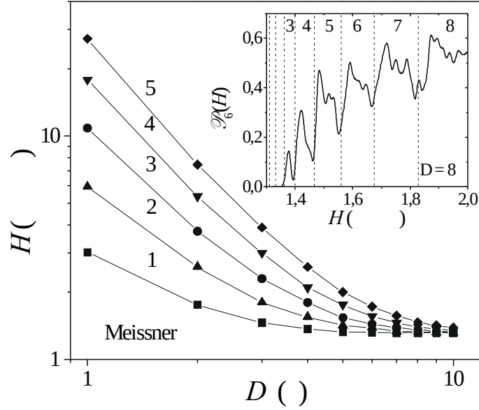
Figura 3.6: Diagrama de fase metaestável H - D (campo externo vs. espessura do filme) para o ramo crescente do ciclo de magnetização. Os dados correspondem aos campos de matching H_1 \equiv H_{en} (■), H_2 (▲), H_3 (●), H_4 (▼) e H_5 (◆) obtidos pelas simulações realizadas para filmes de espessura \lambda \leq D \leq 10\lambda .
