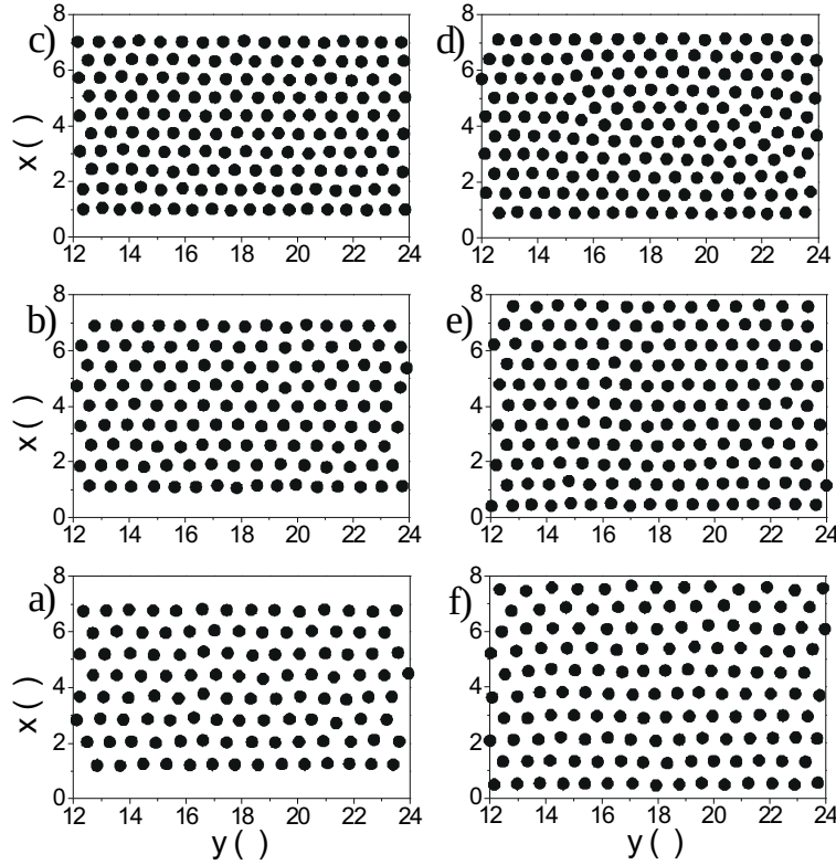
Figura 3.5: Configurações da rede de vórtices em um pedaço do filme de D = 8\lambda para os pontos A, B, C, D e F indicados na Fig. 3.4. Os valores do campo externo em unidades de \Phi_0/\mu_0\lambda^2 são, respectivamente: 1,9 (a), 2,2 (b) e 2,4 (c), para campo crescente, e 2,4 (d), 1,8 (e) e 1,52 (f), em campo decrescente.
