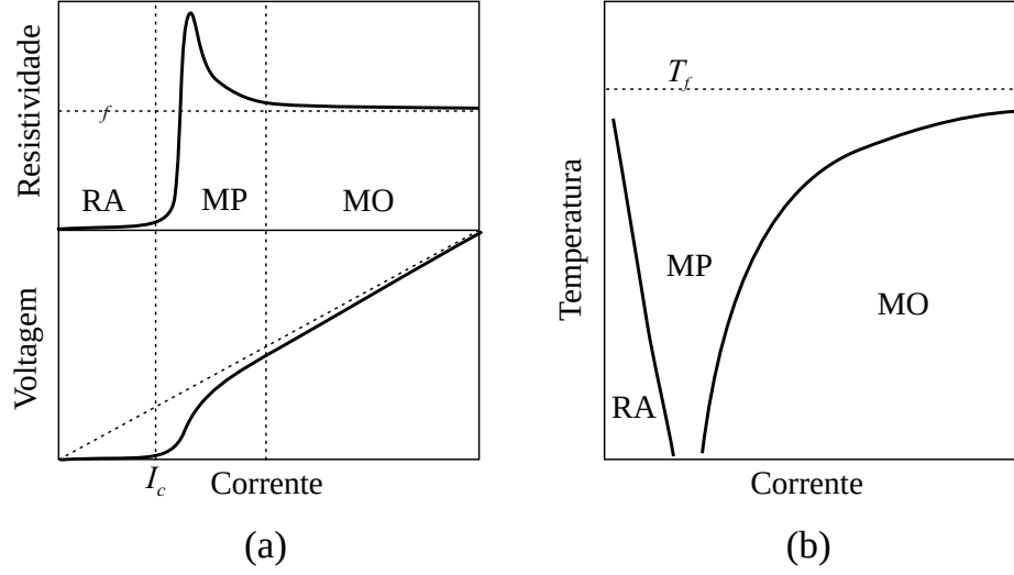
Figura 2.7: (a) Curvas características de voltagem-corrente (painel superior) e resistividade-corrente (inferior) típicas de um supercondutor desordenado. O sinal de voltagem é proporcional à velocidade média dos vórtices no interior do espécime. A queda abrupta do sinal de resistividade é usualmente associada a uma transição de uma fase desordenada para uma fase ordenada. (b) Diagrama de fases dinâmicas esquemático baseado em teorias recentes sobre fases dinâmicas de vórtices. Em baixas temperaturas e correntes, a rede de vórtices encontra-se ancorada (RA). Aumentando a corrente, os vórtices passam por uma fase de movimento plástico (MP) e, em seguida, cristalizam em uma fase de movimento ordenado (MO). A curva de recristalização (ou fusão dinâmica) assintota a temperatura de fusão de equilíbrio para correntes altas.
