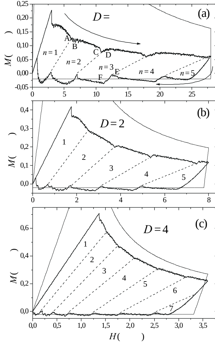
Figura 3.2: Curvas de magnetização (linhas contínuas espessas) calculadas para filmes homogêneos de espessura D = \lambda (a), 2\lambda (b) e 4\lambda (c). As linhas retas intermitentes são apenas guias para uma melhor identificação das fases estruturais. O número entre estas linhas indicam o número de cadeias de vórtices da fase respectiva. As linhas finas correspondem ao resultado macroscópico de Clem (veja texto).
