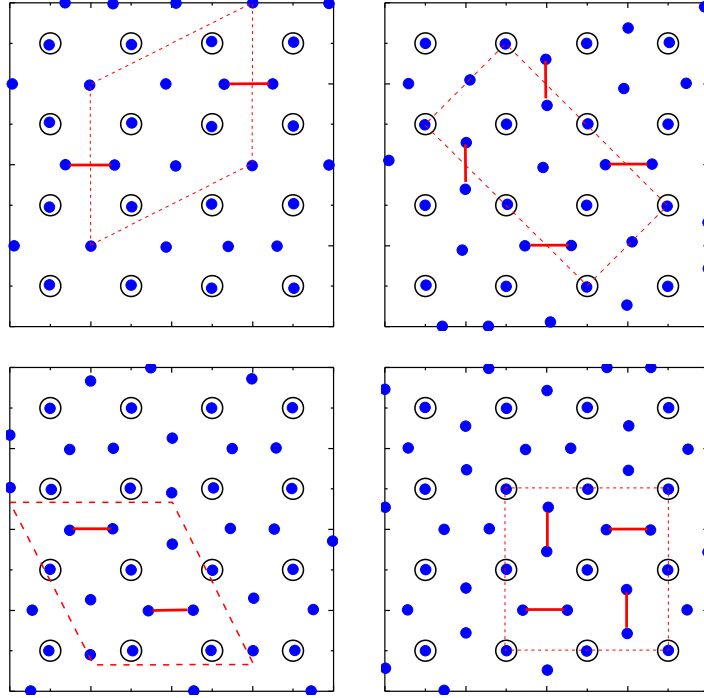
Figura 4.3: Mesmo que a Fig. 4.1, mas para n = 2, 25, 2,5, 2,75 e 3.
