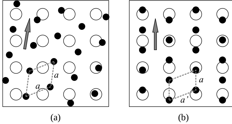
Figura 5.1: Movimento de uma rede de vórtices sobre um rede quadrada de centros de ancoragem. Em (a), a rede se move em uma direção (indicada pela seta) de baixa simetria do potencial de ancoragem. O movimento é incomensurável e a rede é essencialmente idêntica à rede de equilíbrio (triangular) pois o potencial de ancoragem não é capaz de deformá-la (veja texto). Em (b), o movimento é comensurável sobre uma direção de alta simetria da rede de ancoragem. A comensurabilidade é parcial, ocorrendo apenas na direção perpendicular ao movimento.
