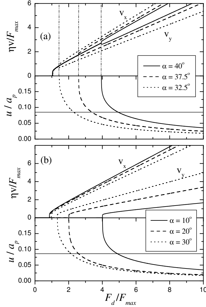
Figura 5.3: Componentes v_x e v_y da velocidade do centro de massa e raiz da média quadrática das flutuações u como funções da intensidade da força motriz F_d para várias direções \alpha da força motriz. (a) 32,5^\circ \leq \alpha \leq 40^\circ : o movimento dos vórtices é capturado pela direção [1,1] do potencial de ancoragem ( v_x = v_y ) para valores de F_d menores que os indicados pelas linhas ponto-tracejadas verticais. (b) 0^\circ < \alpha < 32,5^\circ : o movimento é capturado na direção [1,0] ( v_y = 0 ). As linhas horizontais nos painéis inferiores de (a) e (b) correspondem a u = c_L a para B = 2B_\Phi e c_L = 0, 12 (veja texto), acima da qual a fase elástica se torna instável em relação a flutuações.
