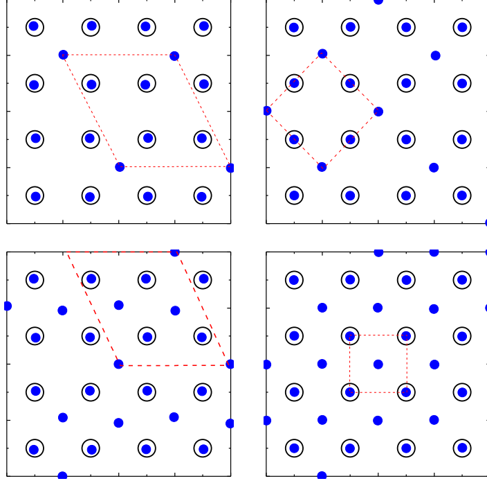
Figura 4.2: Mesmo que a Fig. 4.1, mas para n = 1, 25, 1,5, 1,75 e 2 .
