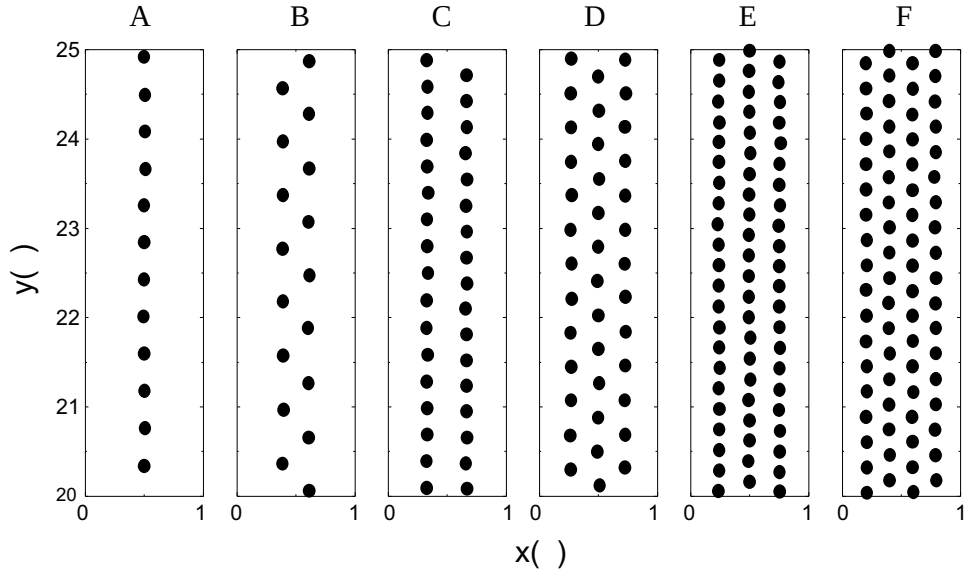
Figura 3.3: Configurações da rede de vórtices em um pedaço do filme de D = \lambda para os pontos A, B, C, D, E e F indicados na Fig. 3.2.
