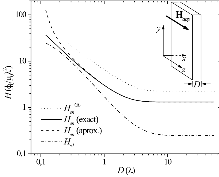
Figura 3.1: Campo de entrada H_{en} dos vórtices em função da espessura do filme D calculado usando a Eq. (3.27) (linha contínua) e a Eq. (3.27) (linha tracejada). A linha pontilhada corresponde ao campo de penetração H_{en}^{GL}(D) obtido pela teoria de Ginzburg-Landau unidimensional (de Gennes, 1965). A linha ponto-tracejada corresponde ao campo crítico inferior H_{cl}(D) .
