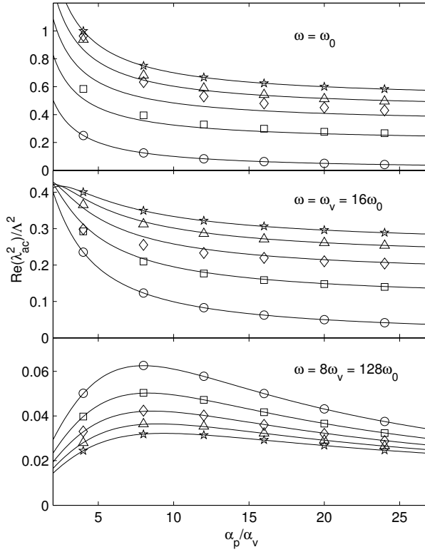
Figura 4.9: Parte real do comprimento de penetração ac \lambda_{ac} em função de \kappa_p para os valores de frequência \omega = \omega_0 , \omega_v , e 8\omega_v (de cima para baixo). Os símbolos têm o mesmo significado que na Fig. 4.8. As linhas foram obtidas do modelo de duas espécies usando a Eq. 4.26.
