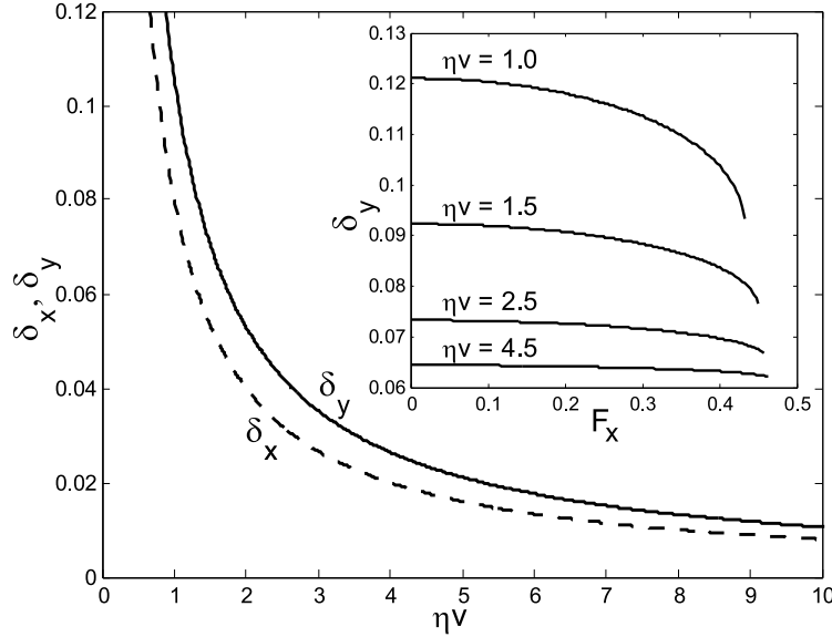
Figura 5.7: Raiz do desvio quadrático médio das flutuações transversais ( \delta_x ) e longitudinais ( \delta_y ) para movimento na direção [0,1] e T = 0 em função da velocidade do c.m., v . As forças estão normalizadas pela força máxima de ancoragem F_{max} = 8\pi|U_1|/a_p e os comprimentos estão normalizados pela periodicidade do potencial de ancoragem. Gráfico menor: Dependência de \delta_y com a força transversal F_x para valores fixos de v .
