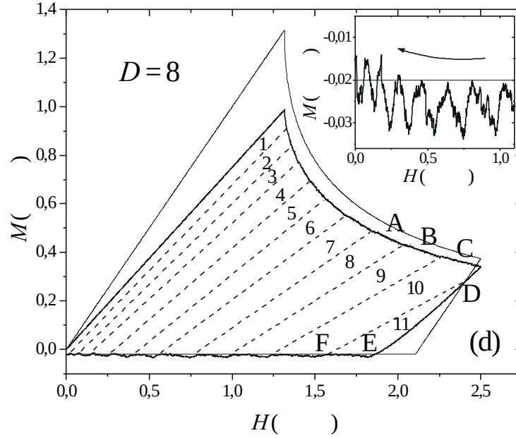
Figura 3.4: Mesmo que Fig. 3.2, mas para D = 8\lambda . No canto direito superior é mostrada uma ampliação de um trecho do ramo decrescente da magnetização.
