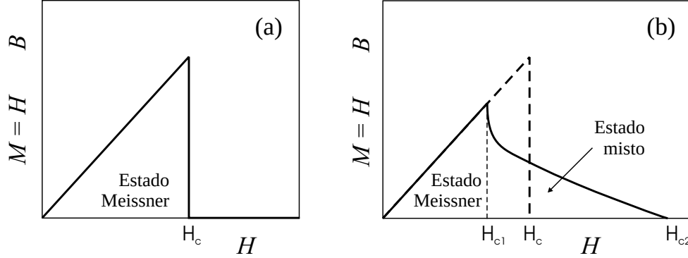
Figura 2.3: Magnetização de equilíbrio em função do campo externo para um supercondutor do tipo I (a) e um supercondutor do tipo II. Os campos críticos correspondentes estão indicados.
