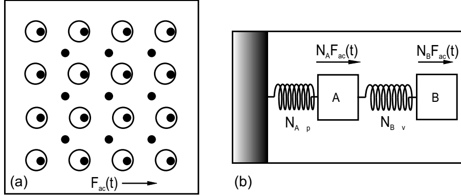
Figura 4.5: (a) Representação esquemática de uma rede de vórtices para B = 2B_\Phi sob a ação de uma força uniforme F_{ac} (os círculos vazios representam os centros aprisionados e os cheios representam os vórtices). Note que as sub-redes de vórtices ancorados e de vórtices intersticiais são deslocadas de suas posições de equilíbrio como corpos rígidos, i.e., sem sofrer deformações. Esse problema pode ser mapeado no análogo mecânico mostrado em (b), onde \kappa_p e \kappa_v representam as constantes elásticas de acoplamento vórtices-rede de defeitos e vórtices ancorados - vórtices intersticiais, respectivamente (veja texto).
