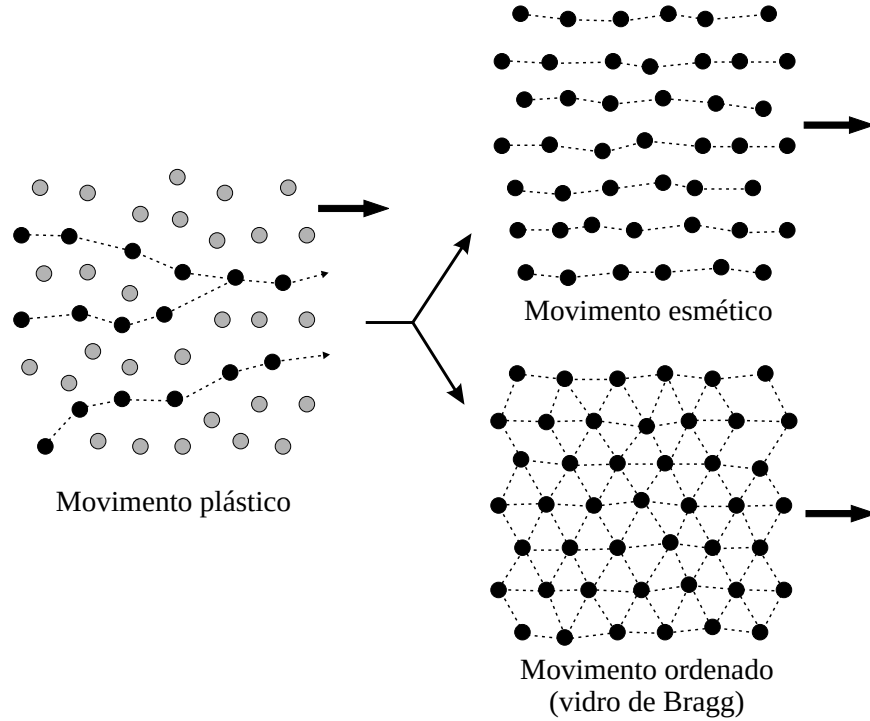
Figura 2.8: Algumas fases dinâmicas possíveis para um sistema de vórtices movidos por uma corrente de transporte. A fase plástica desordenada pode se ordenar em uma fase esmética, com ordem apenas na direção perpendicular ao movimento, ou em uma fase topologicamente ordenada, o vidro de Bragg.
