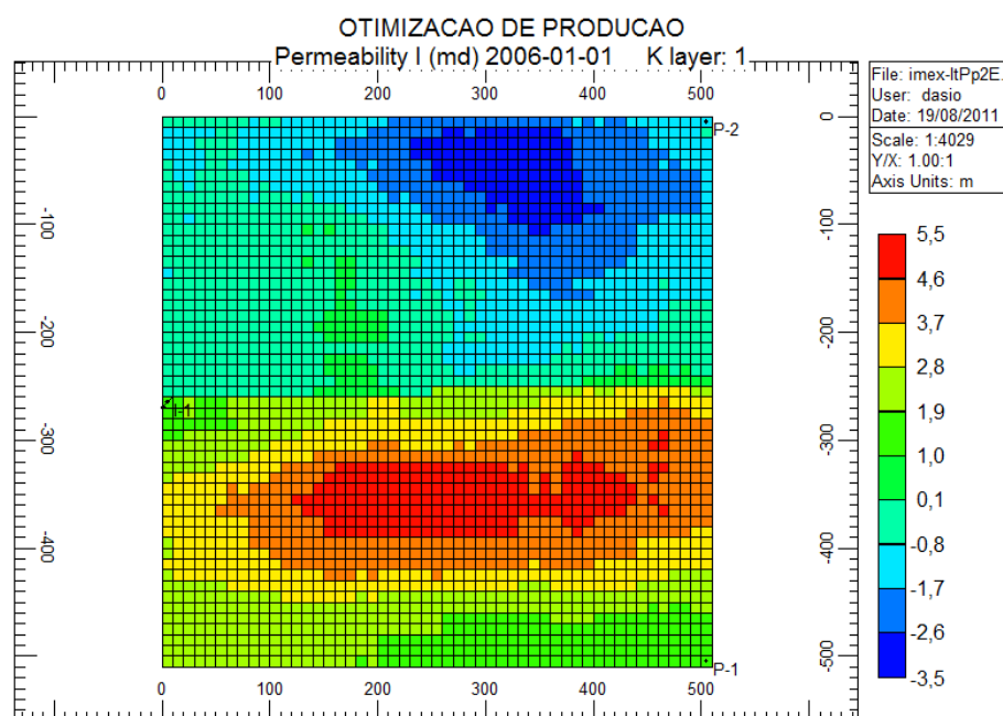
Figura 6.12: Campo de permeabilidades obtido com o processo de ajuste de histórico.
