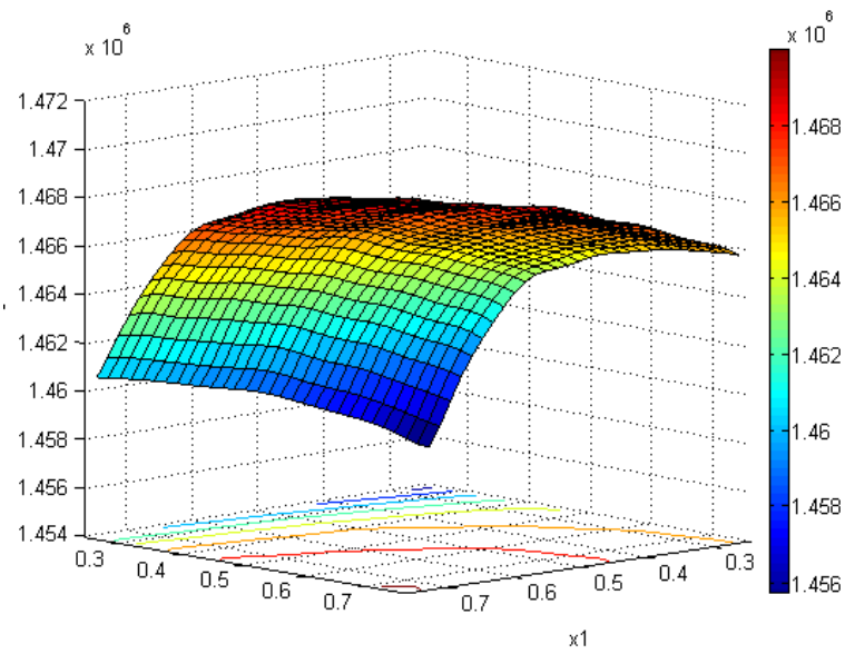
Figura 3.13: Superfícies de VPL para o caso C2 (Restrição de BHP).
