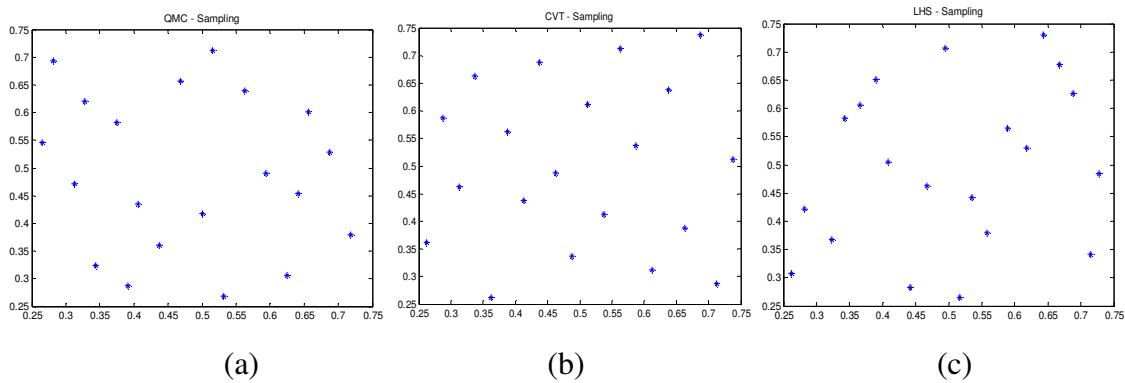
Figura 3.11: Amostras obtidas por DOE na aplicação de engenharia de reservatórios: (a) QMC, (b) LCVT and (c) LHS.
