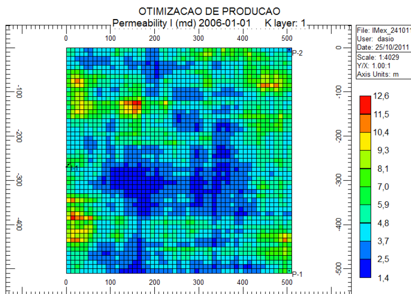
Figura 5.6: Realização escolhida para estudo de otimização determinística.
