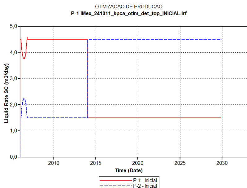
Figura 5.8: Curvas de vazões de líquidos nos poços produtores para o caso inicial.
