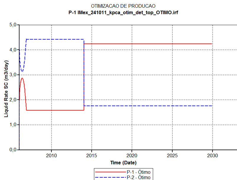
Figura 5.9: Curvas de vazões de líquidos nos poços produtores para o caso ótimo.
