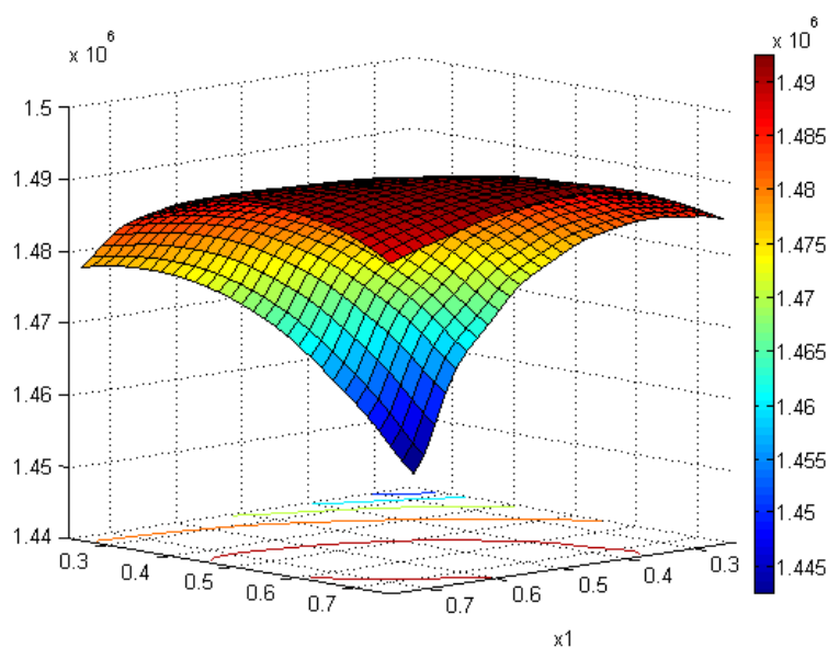
Figura 3.12: Superfícies de VPL para o caso C1 (Nenhuma Restrição).
