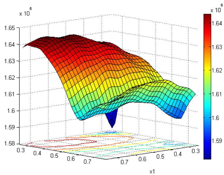
Figura 3.14: Superfícies de VPL para o caso C3 (Restrição de corte de água - WC).
