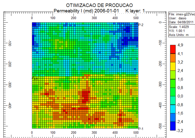
Figura 6.4: Realização escolhida como caso observado (escala logarítmica).
