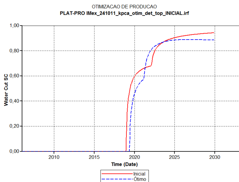
Figura 5.10: Cortes de água para os casos inicial e otimizado.
