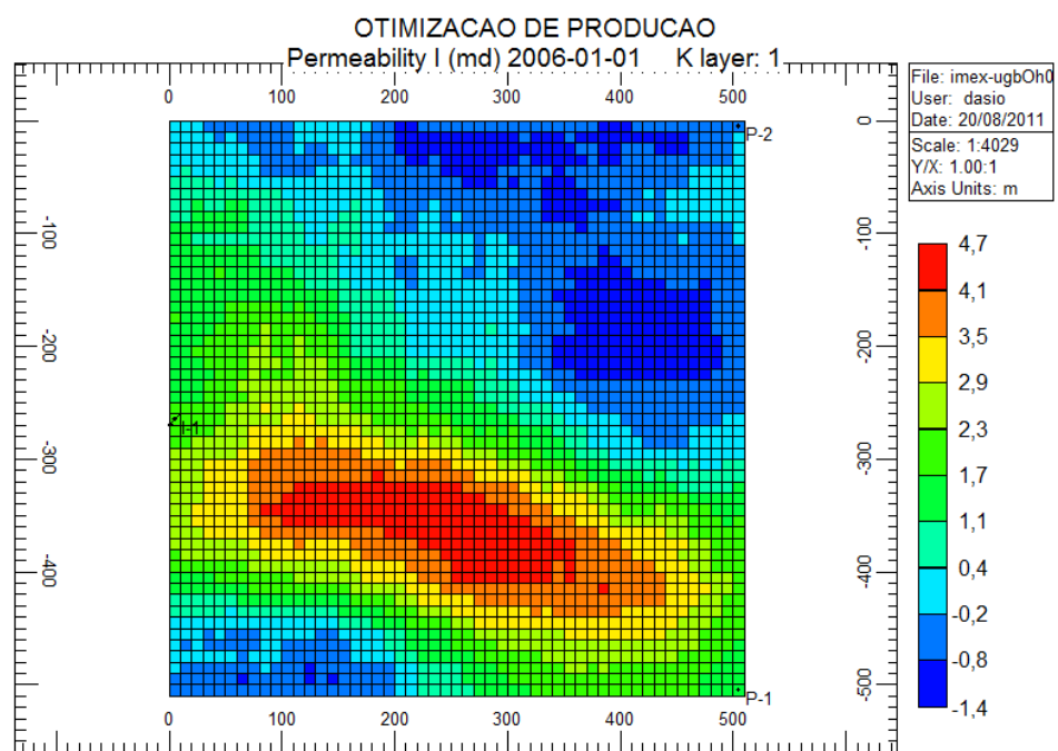
Figura 6.8: Campo de permeabilidades obtido com o processo de ajuste de histórico.
