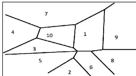
Figura 3.4: O método de tesselação de Voronoi para os pontos da Figura 3.3.
