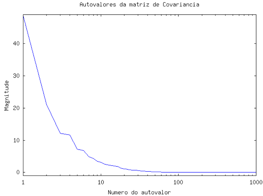
Figura 4.4: Magnitude dos autovalores da Matriz de Covariância.
