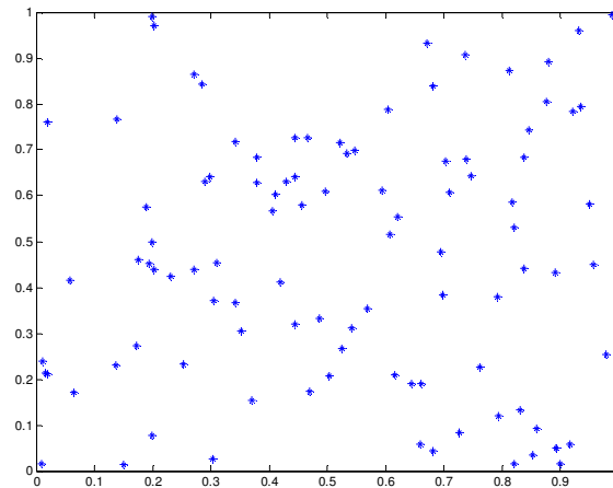
Figura 3.1: Amostragem gerada pelo método de Monte Carlo.
