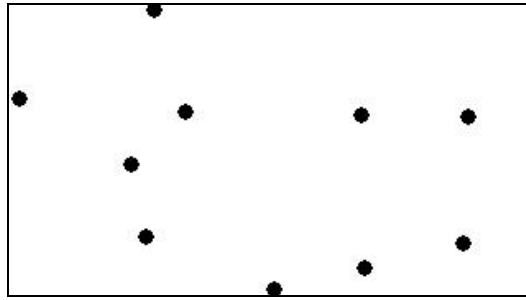
Figura 3.3: Conjunto inicial de pontos geradores.
