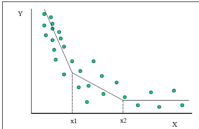
Figura 3.8: Aproximação no espaço bidimensional com aplicação do MARS (Briand et al, 2000).
