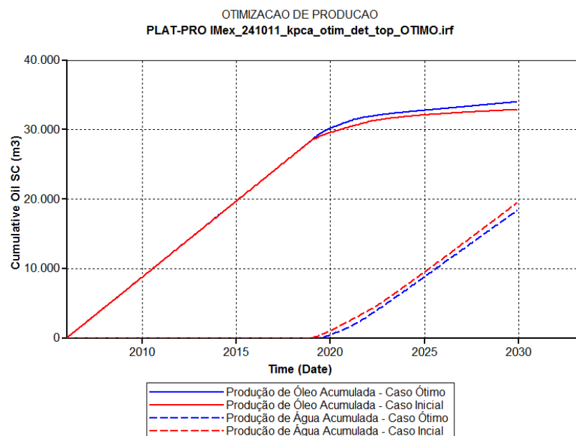
Figura 5.7: Curvas de produção acumulada de óleo e água para os casos inicial e otimizado.
