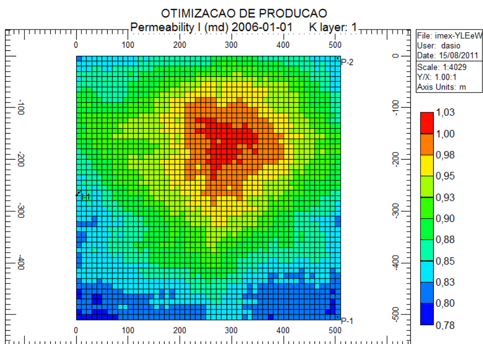
Figura 6.7: Estimativa inicial do campo de permeabilidades.
