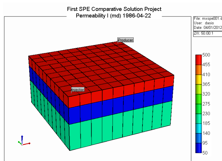
Figura 4.2: Modelo do reservatório com injeção de gás.
