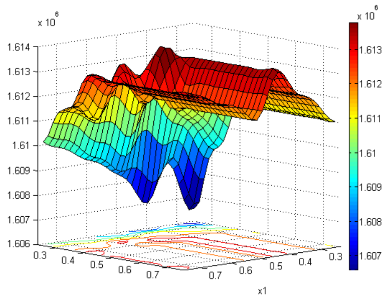
Figura 3.15: Superfícies de VPL para o caso C4 (Restrição de BHP e WC).
