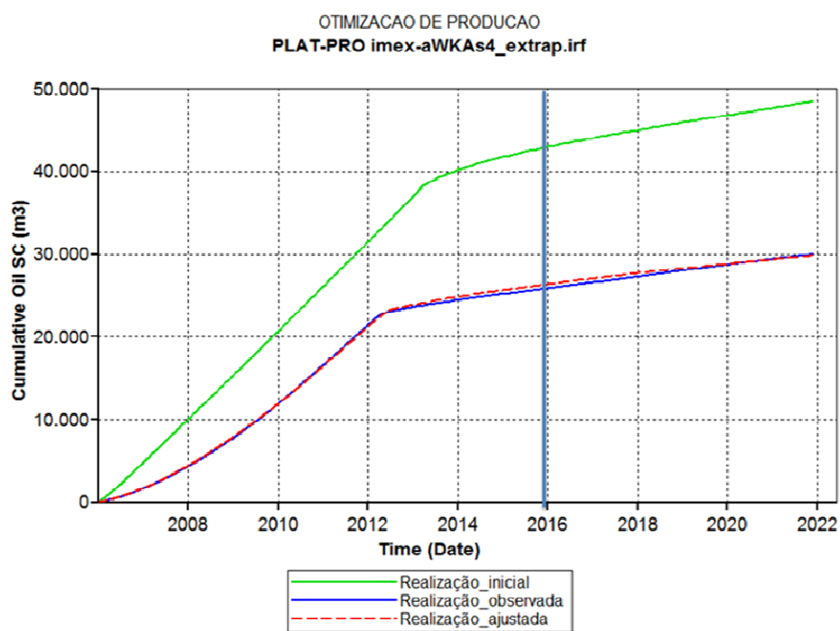
Figura 6.10: Extrapolação das curvas de produção acumulada de óleo obtidas no processo de ajuste de histórico.
