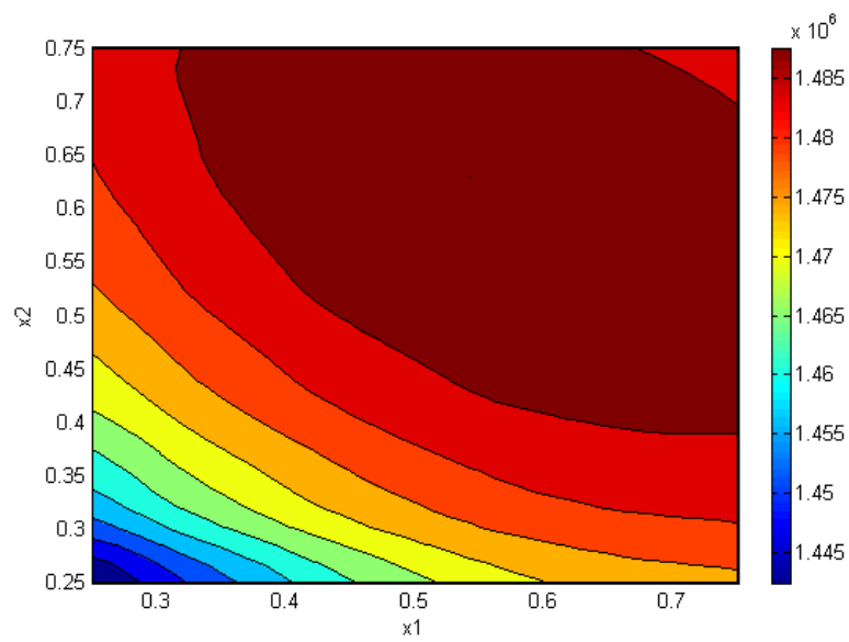
Figura 3.16: Contornos da função de VPL para o caso C1 (nenhuma restrição).
