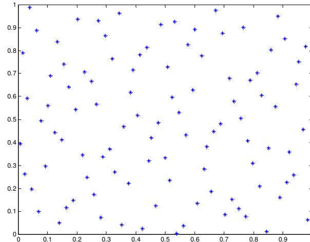
Figura 3.2: Amostragem gerada pelo método de Quasi-Monte Carlo.
