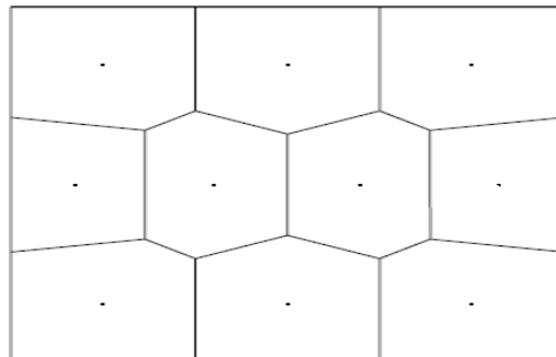
Figura 3.5: O método de tesselação de Voronoi (CVT) após atingir a condição final de uniformidade.
