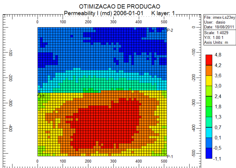
Figura 6.11: Estimativa inicial do campo de permeabilidades.
