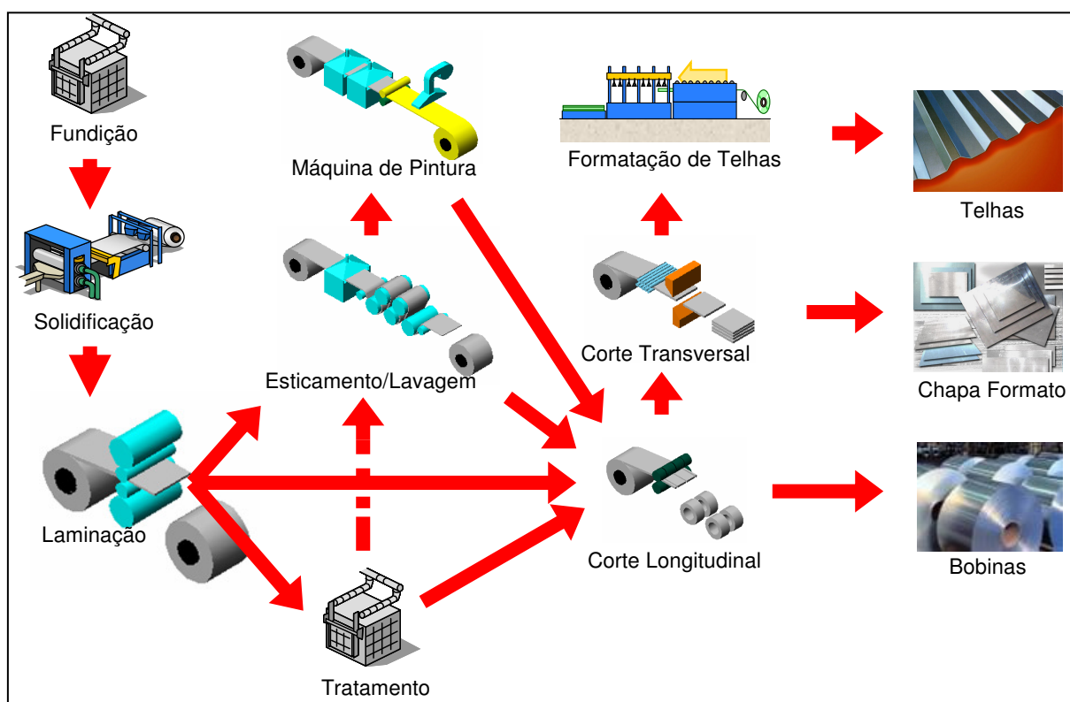
Figura 3.1: Fluxograma de processo da laminação de chapas/telhas
