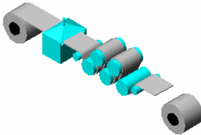
Figura 3.3: Processo de Esticamento e Lavagem
