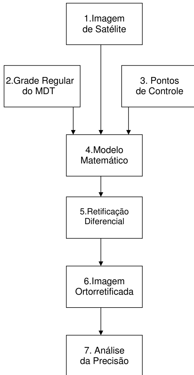
Figura 5.3 - Metodologia de Ortorectificação de Imagens
