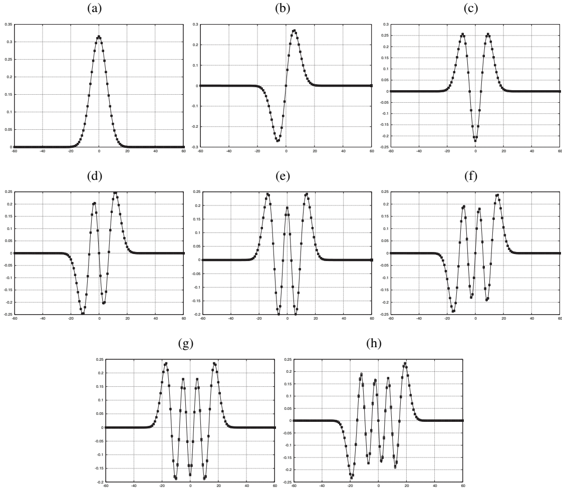
Figura 3 – Amostras dos autovetores HGL \Phi_m ( \square ), \hat{g}_m ( \circ ) e \hat{g}_m^\perp ( \times ), para N = 201 , e os sinais Hermite-Gaussianos contínuos correspondentes \psi_m(t) (linhas), m = 0, 1, \dots, 7 , no intervalo n = -60, -59, \dots, 59, 60 .
