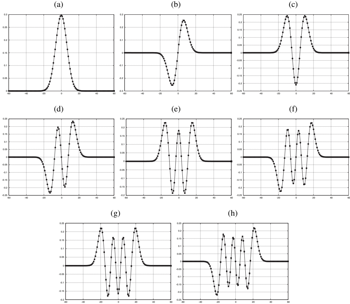
Figura 6 – Amostras dos autovetores HGL \Phi_m ( \square ), \hat{g}_m ( \circ ) e \hat{g}_m^\perp ( \times ), para N = 256 , e amostras dos sinais Hermite-Gaussianos contínuos correspondentes \psi_m(t) (linhas), m = 0, 1, \dots, 7 , no intervalo n = -60, -59, \dots, 59, 60 .
