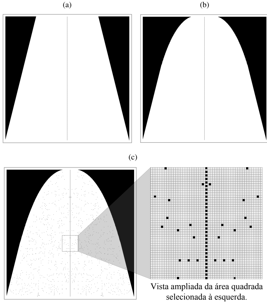
Figura 16 – Imagens da matriz \mathbf{E}^T , N = 512 , para (a) matriz sem arredondamento, (b) com arredondamento na nona casa decimal e (c) com arredondamento na terceira casa decimal; regiões pretas e brancas representam componentes nulas e não-nulas, respectivamente.
