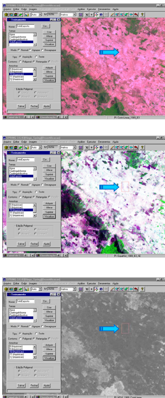
Figura 64 – Avaliação visual das amostras de treinamento para a classificação supervisionada, considerando-se os diversos PDI's anteriormente realizados (Data: 11/03/89): ao alto, análise de uma amostra da classe “Solo Exposto” sobre uma composição colorida RGB 543; ao centro, a mesma amostra sobre uma Equalização de Histograma; acima, a mesma amostra sobre o NDVI com Contraste Linear aplicado.
