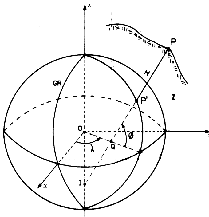
Figura 38 – Elipsóide Geocêntrico.
