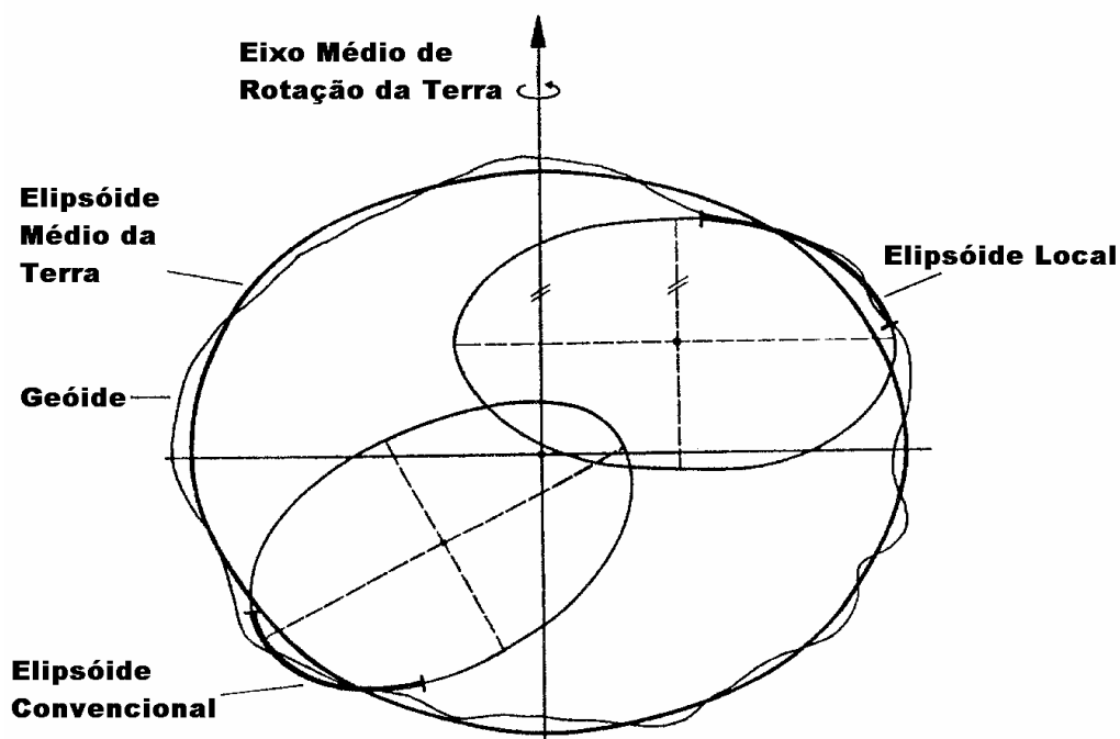
Figura 39 – Elipsóides Convencional e Local.
