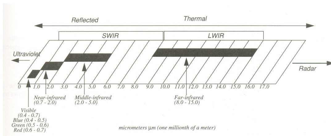
Figura 14 – Espectro Eletromagnético.
