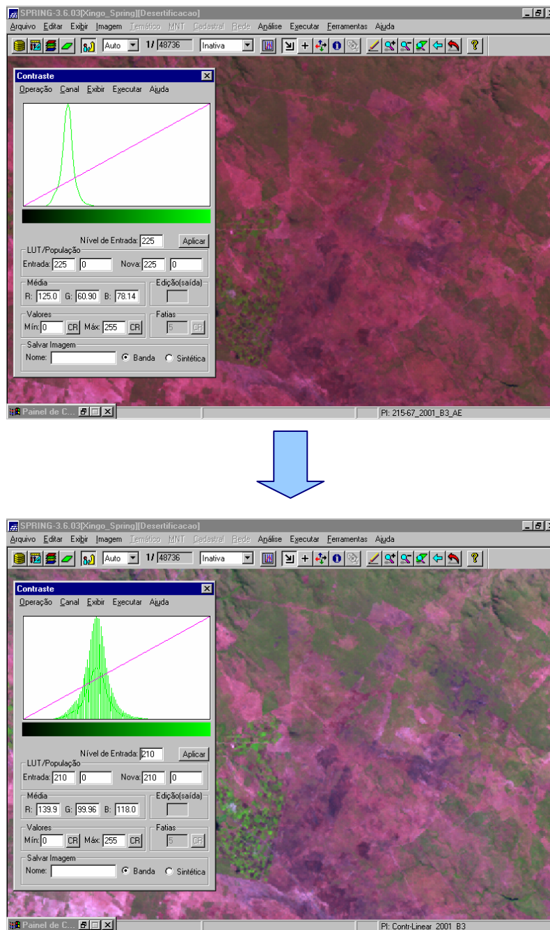
Figura 43 – Aplicação da técnica de realce linear: ao alto, antes da manipulação do histograma; acima, após a manipulação, observando-se a melhoria da qualidade na imagem resultante com o deslocamento do histograma ao longo do eixo de NC's (Combinação Espectral RGB 543 – Falsa Cor; Data: 05/01/03).
