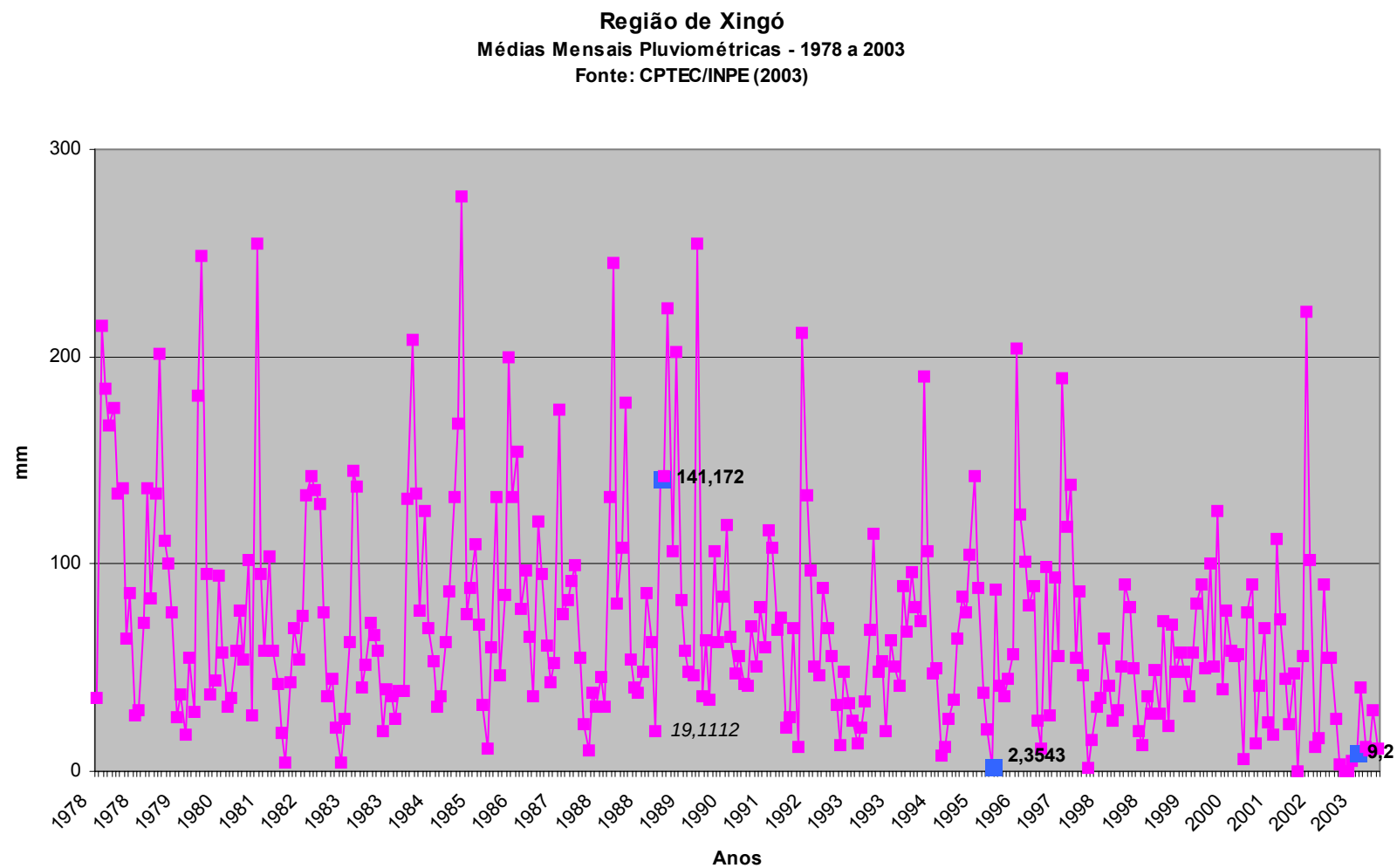
Figura 36 – Gráfico com os dados de médias mensais pluviométricas da Região de Xingó e datas escolhidas das imagens (azul).
