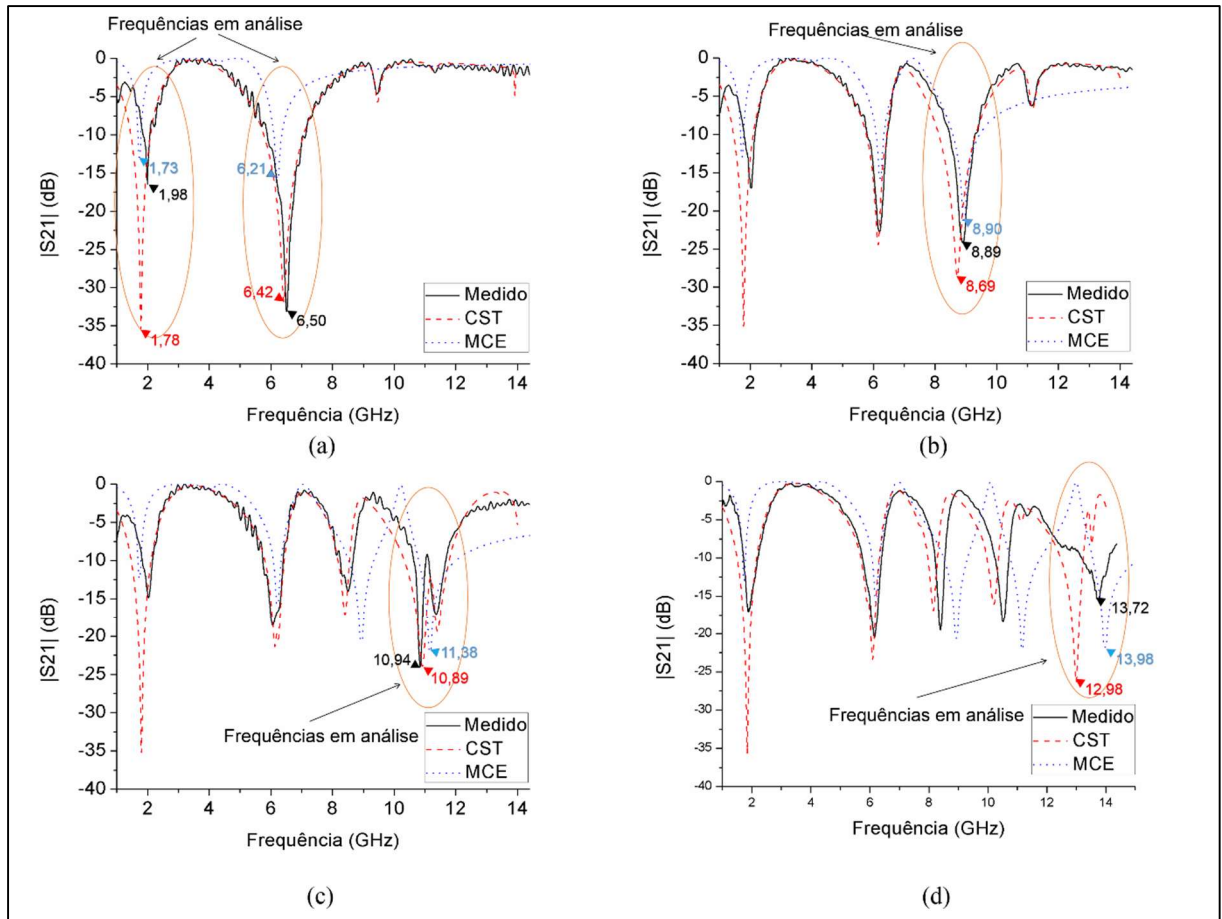
Figura 55 Comparação entre os modelos simulados, medidos e numéricos para a FSS-CJM com efeito do substrato (a) Iteração 0; (b) Iteração 1; (c) Iteração 2; (d) Iteração 3.
