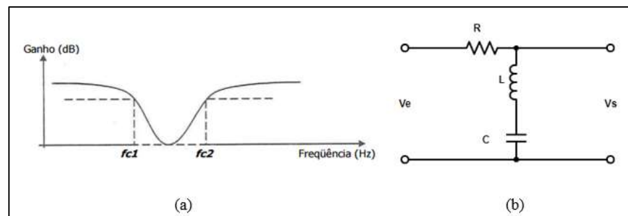
Figura 4 Rejeita-Faixa; (a) Resposta em frequência do filtro ideal; (b) Modelo em circuito discreto.
