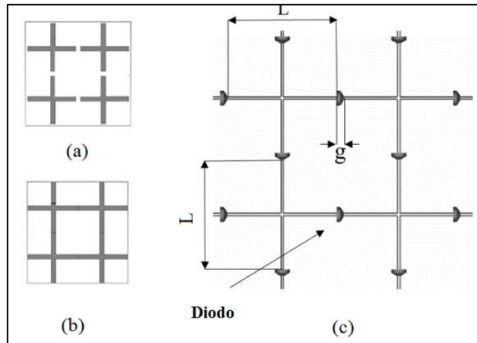
Figura 14 Células unitárias da FSS: (a) Elemento Dipolo Cruzado; (b) Elemento de Grade; (c) Dipolos Cruzados conectados por diodos.
