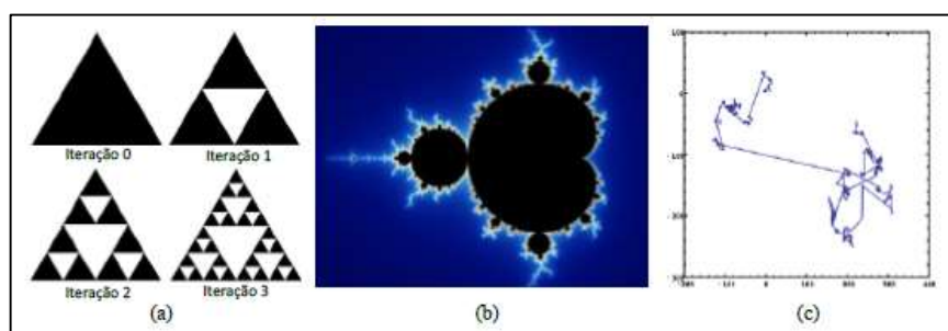
Figura 24 Exemplos de fractais. (a) Triângulo de Sierpinski (auto-similaridade exata). (b) Conjunto de Mandelbrot (quase-auto-similaridade). (c) Voo de Lévy (auto-similaridade estatística).
