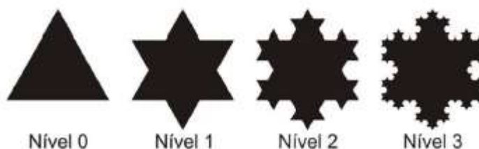
Figura 23 Fractal Ilha de Koch
