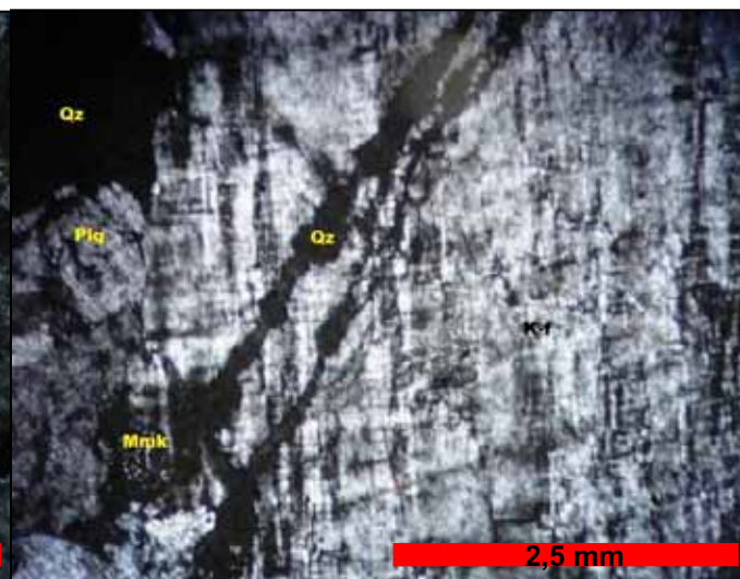
Figura 2: Intrusão de quartzo (Qz) na Microclina (K-f). Também presente um pequeno cristal com textura mirmekítica (Mmk). Nicóis cruzados.
