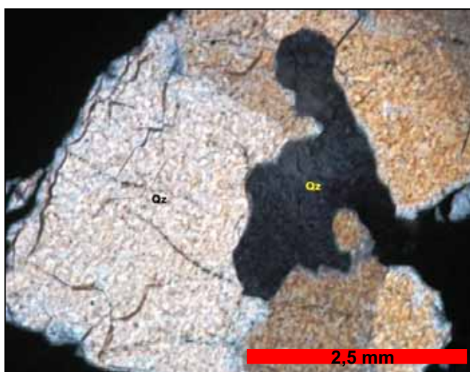
Figura 1: Cristal de quartzo (Qz) bastante fraturado com formato anedral. Nicóis cruzados.
