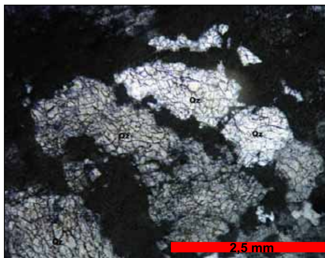
Figura 1: Cristais de quartzo (Qz) micro-fraturados. Nicóis cruzados.
