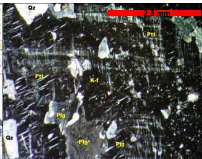
Figura 6: Presença de pertita (Ptt), representada pelo intercrecimento de plagioclásio (plg) em um megacrystal de K-feldspato (K-f). Também presentes alguns cristais de quartzo (Qz). Nicóis cruzados.
