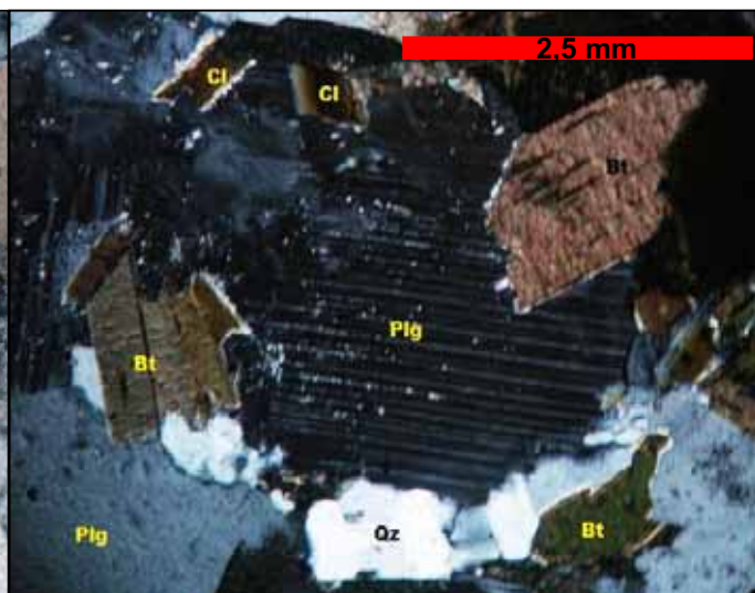
Figura 4: Megacrystal de plagioclásio (Plg) com geminação albita bem definida associado à palhetas de biotita (Bt) com bordas corroídas, em alguns pontos alterando para clorita (Cl). Nicóis cruzados.
