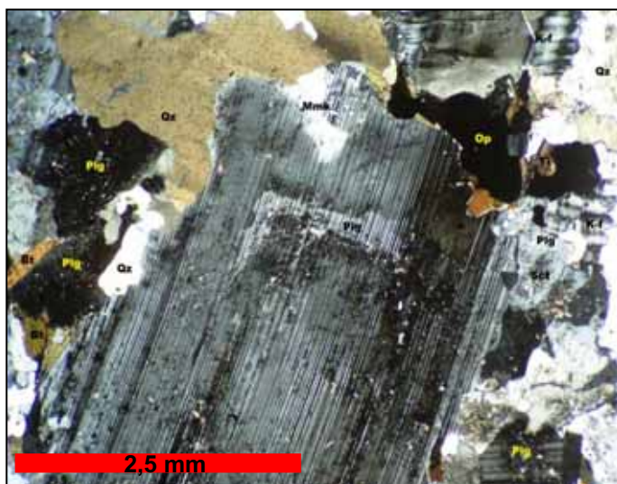
Figura 5: Megacrystal de plagioclásio (Plg) com bordas corroídas associado a quartzo (Qz), K-feldspato (K-f), minerais opacos (Op) e biotita (Bt). Também há presença de alteração sericita (Sct) pontual em alguns cristais de plagioclásio (Plg) menores. Nicóis cruzados.
