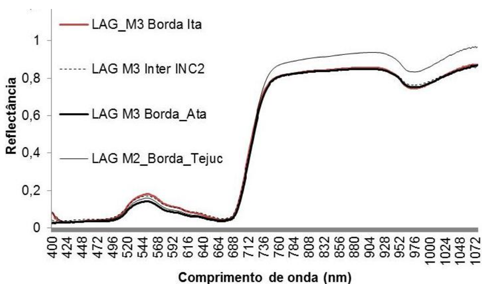
Figura 07: Comportamento espectral médio (n=4) da espécie L. racemosa .
