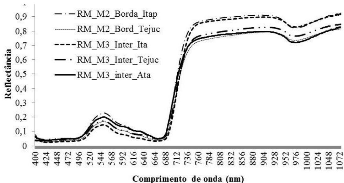
Figura 05: Comportamento espectral médio (n=5) da espécie R. mangle .
