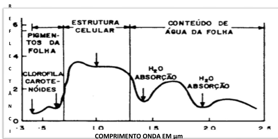
Figura 02: Comportamento espectral de uma folha verde sadia.
