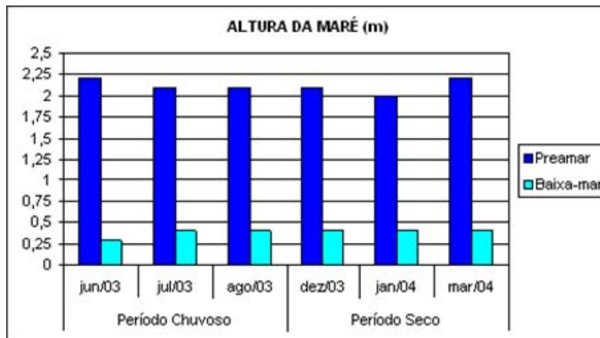
Figura 7 – Altura das marés referentes aos dias da coleta no sistema estuarino de Barra das Jangadas.
