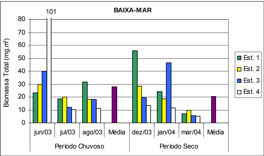
Figura 51 – Variação sazonal da biomassa total no sistema estuarino de Barra das Jangadas durante a baixa-mar.
