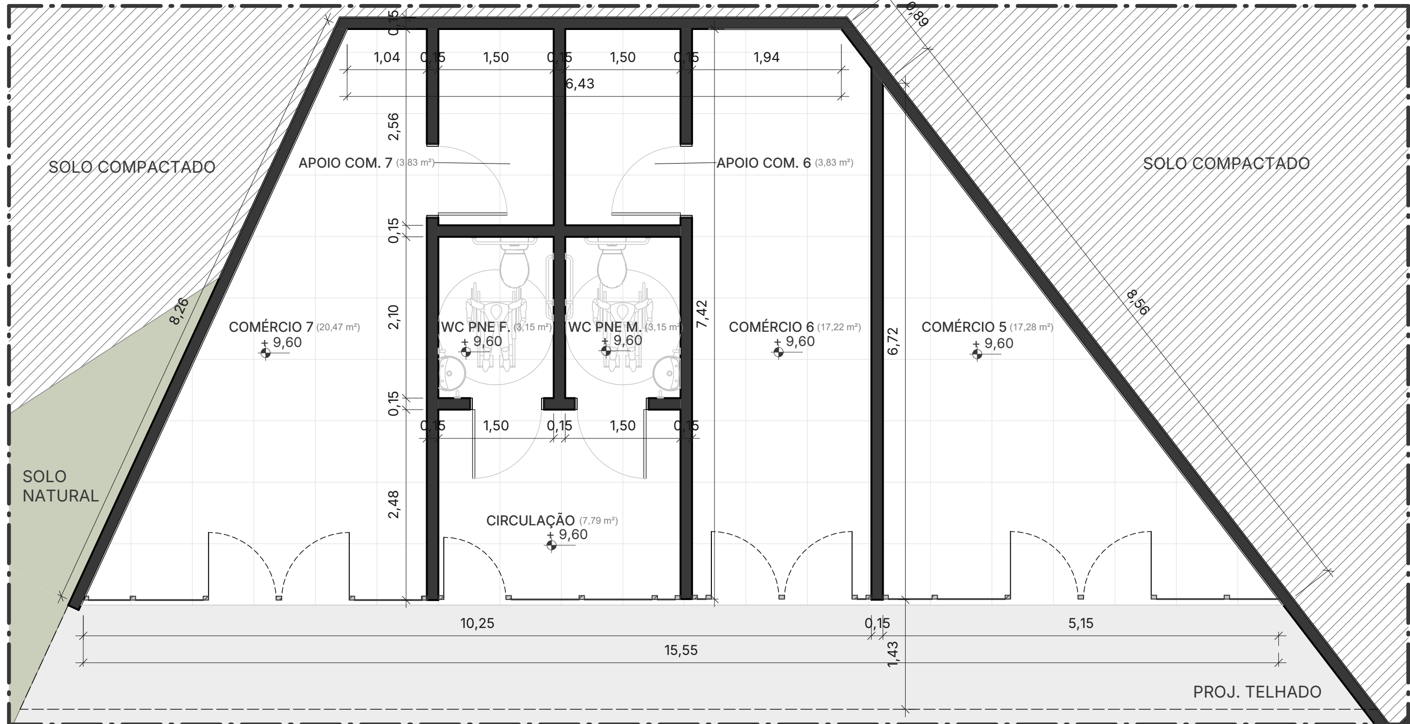
PLANTA BAIXA - COMÉRCIO 5, 6 E 7 ESC: 1: 50
