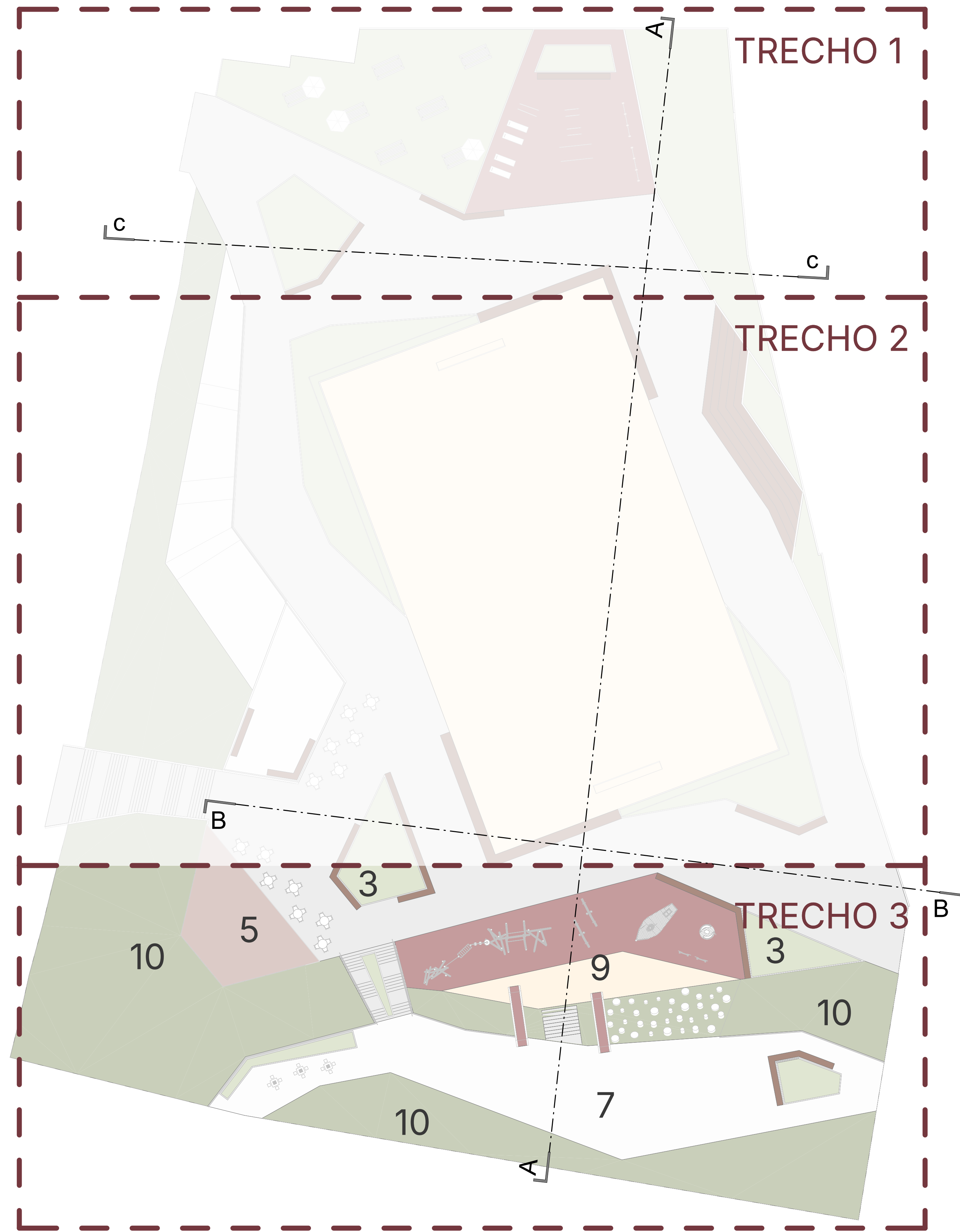
PLANTA CHAVE PRAÇA - TRECHO 3 ESC: 1: 250
