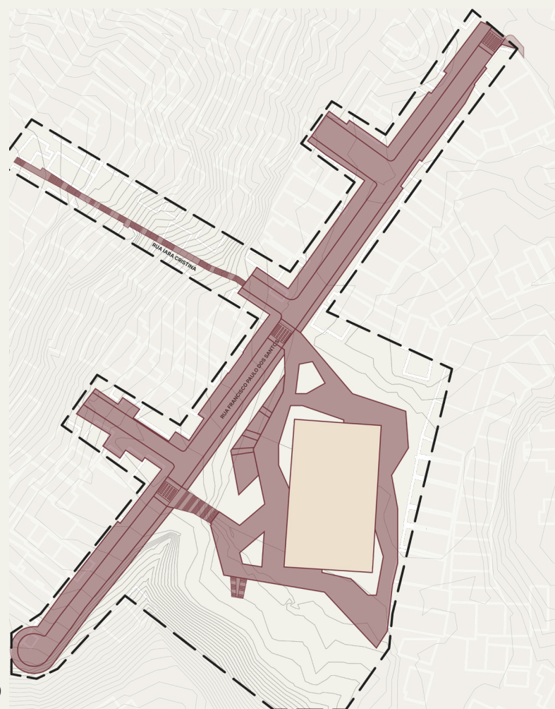
Figura 53 - Conectar: requalificar caminhos existentes e criar novos. Fonte: Autora, 2025.
