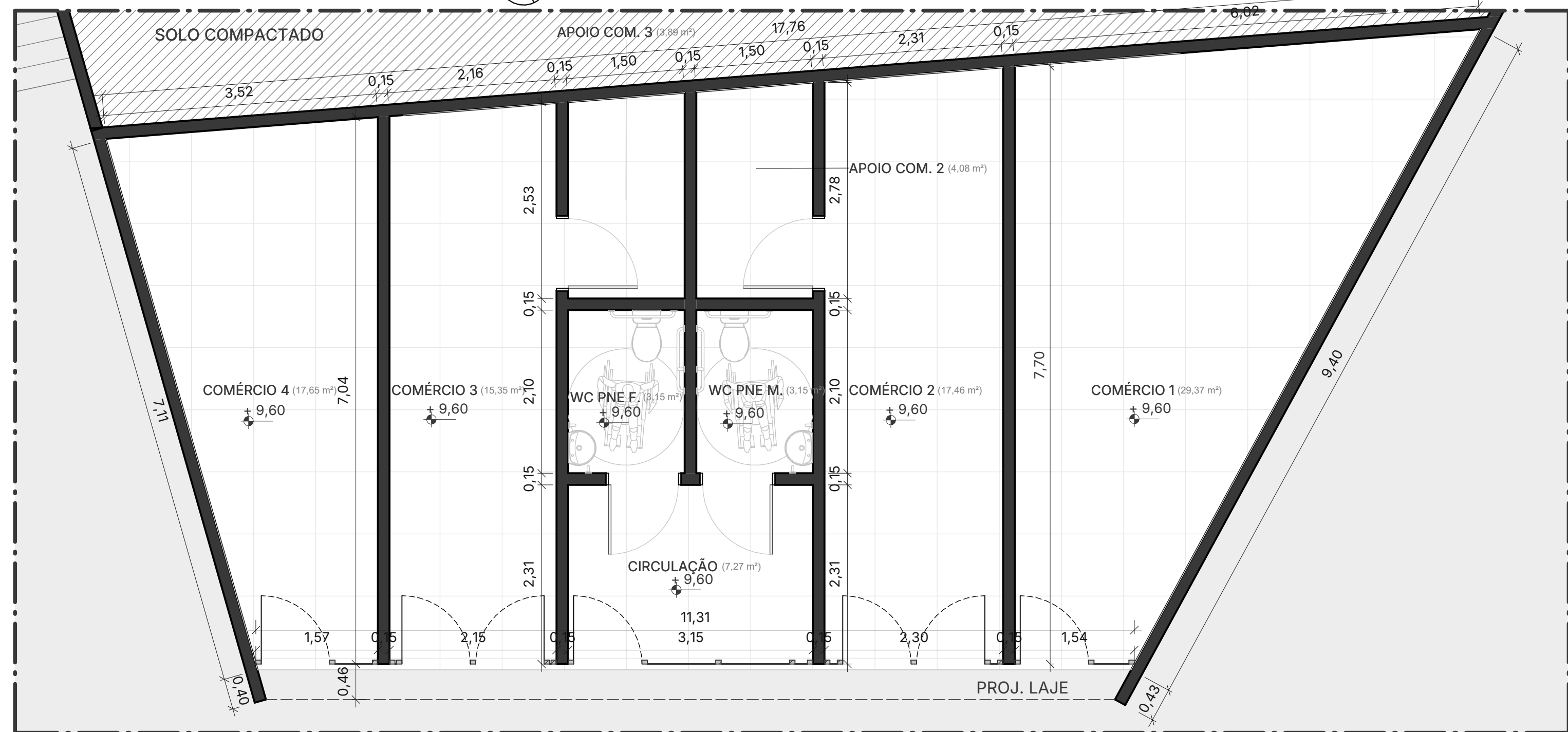
PLANTA BAIXA - COMÉRCIO 1, 2, 3 E 4 ESC: 1: 50
