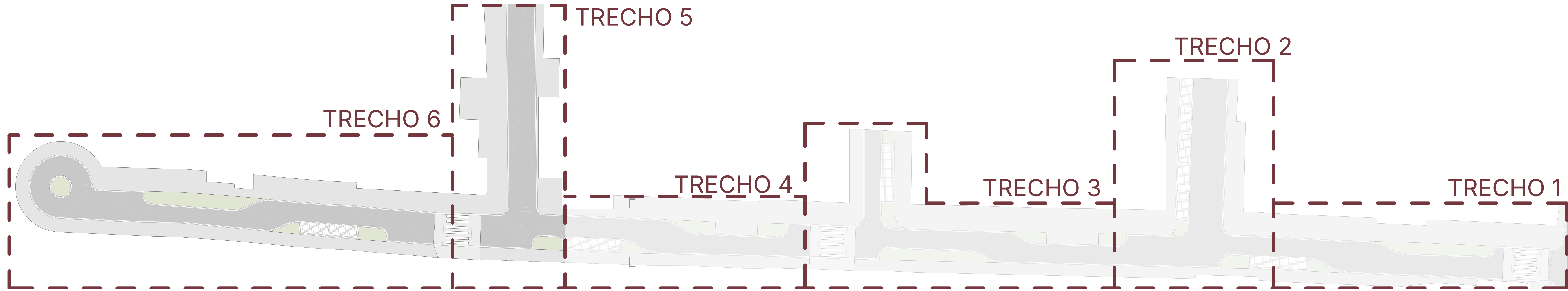
PLANTA CHAVE RUA - TRECHO 4, 5 E 6 ESC:1 : 300
