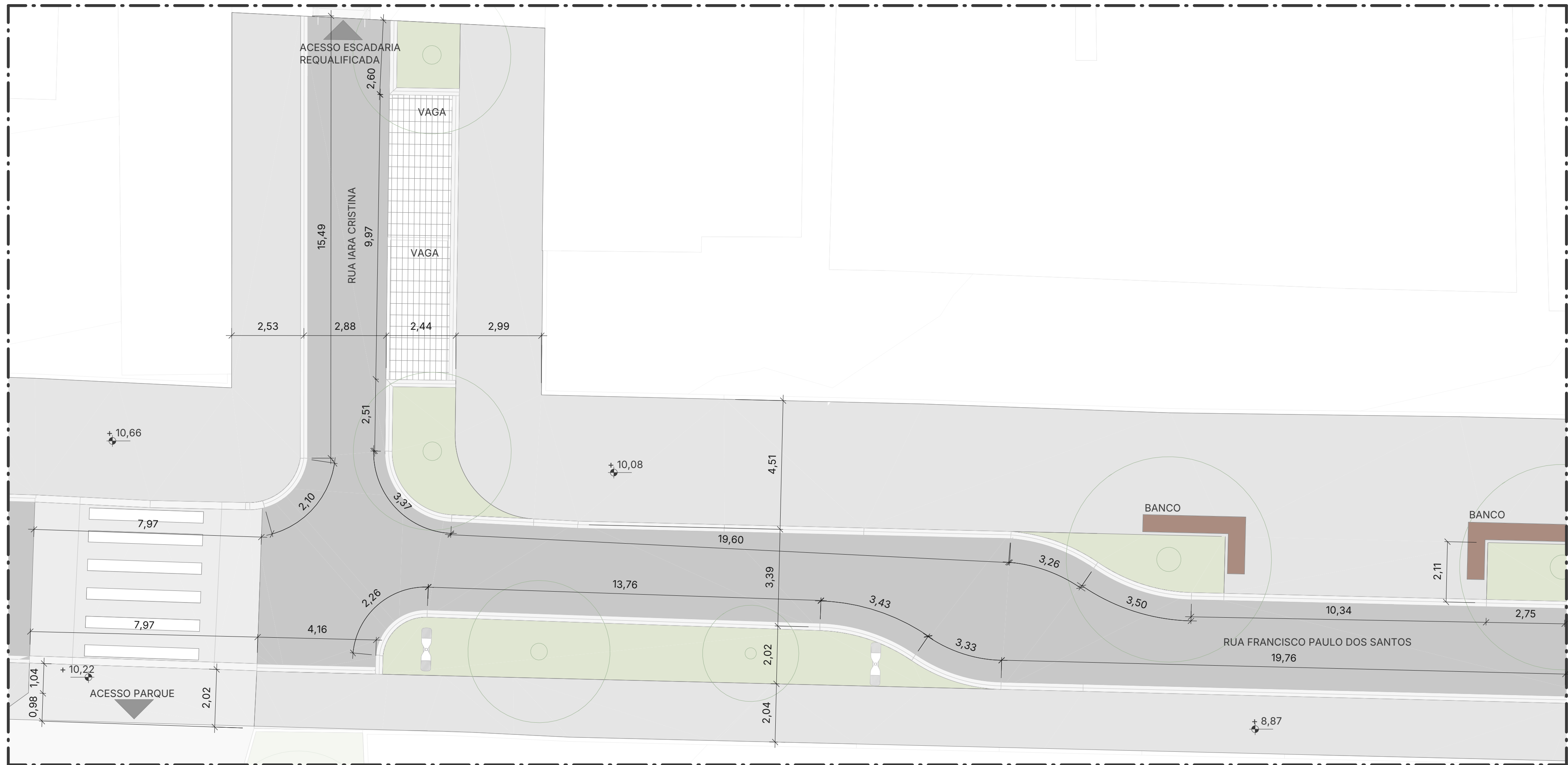
TRECHO 3 - PLANTA BAIXA RUA ESC: 1 : 100
