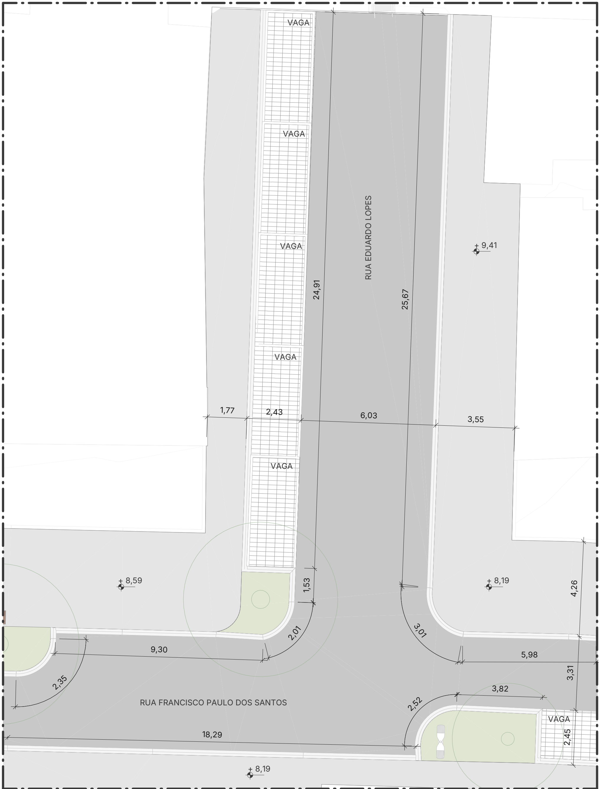
TRECHO 2 - PLANTA BAIXA RUA ESC: 1 : 100
