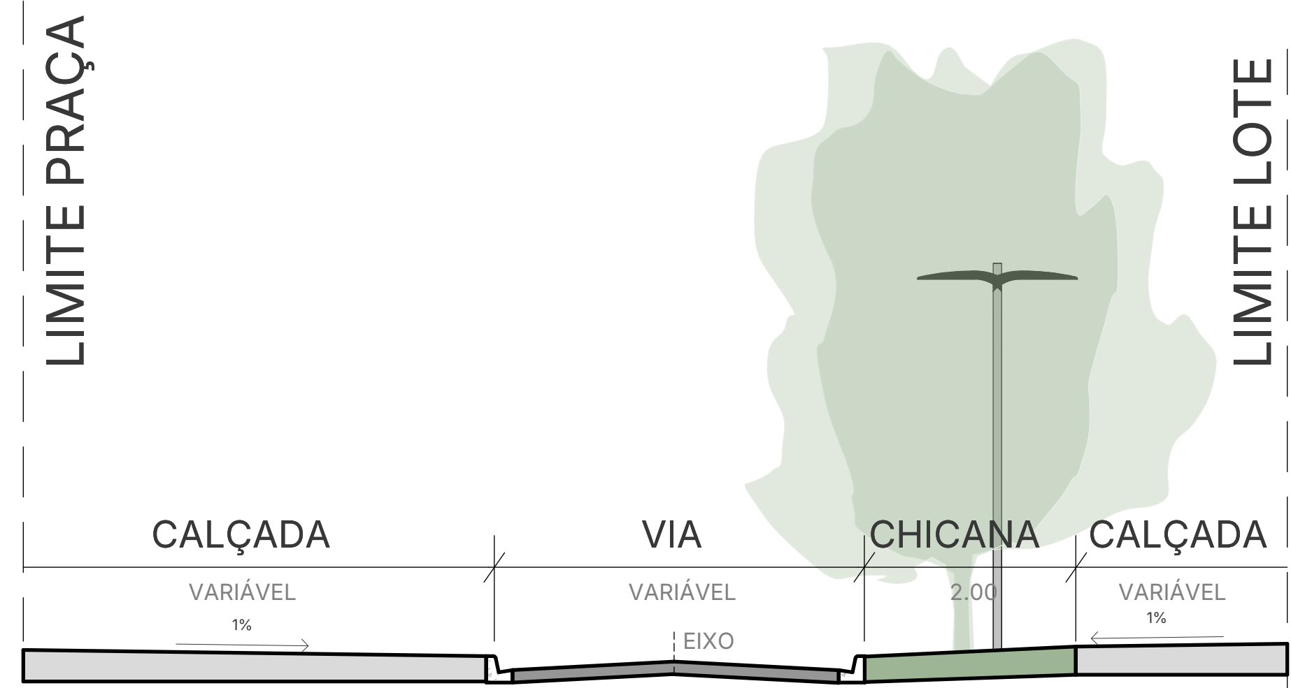
PERFIL DA RUA ESQUEMÁTICO ESC: 1 : 50
