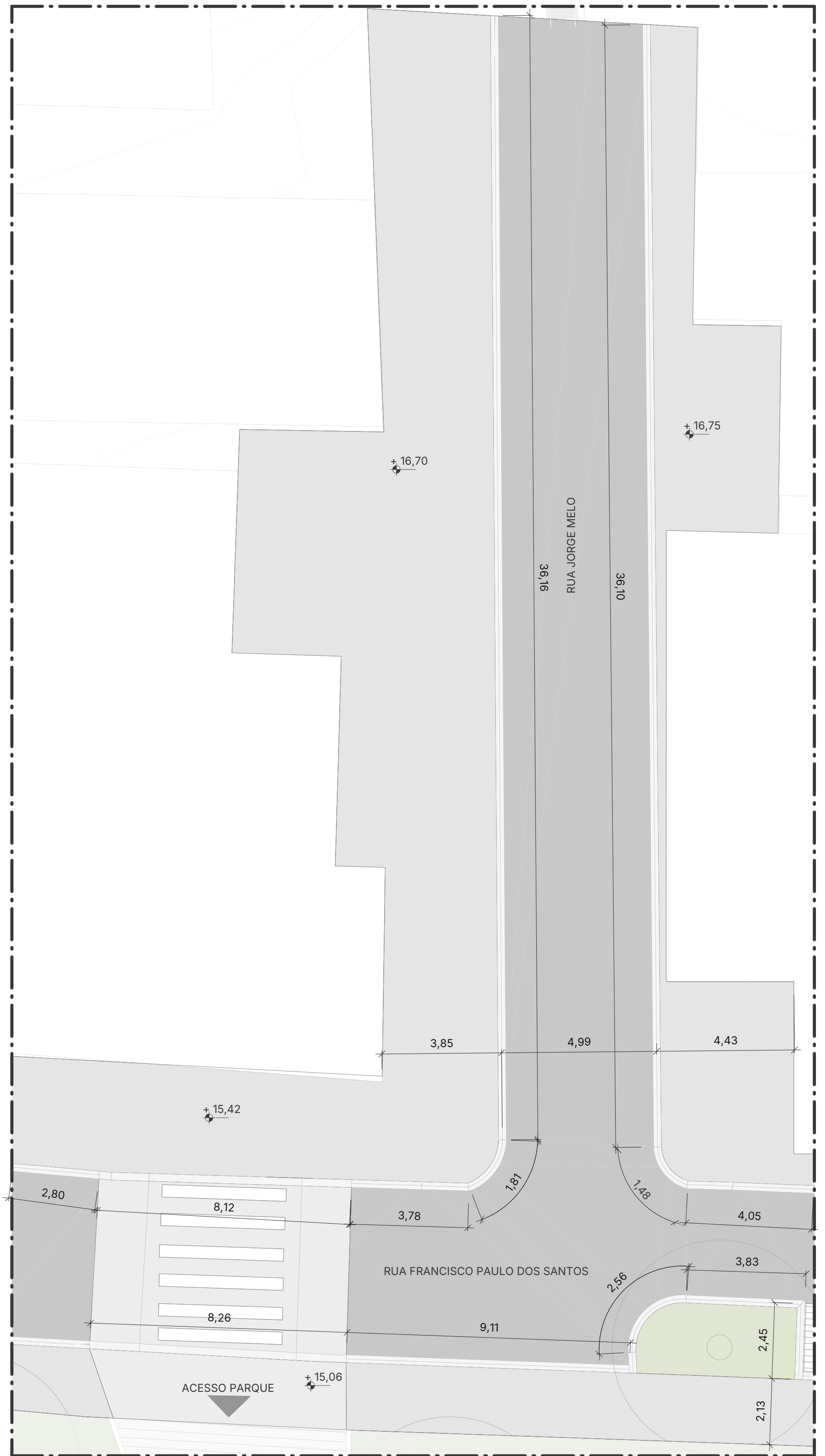
TRECHO 5 - PLANTA BAIXA RUA ESC: 1 : 100
