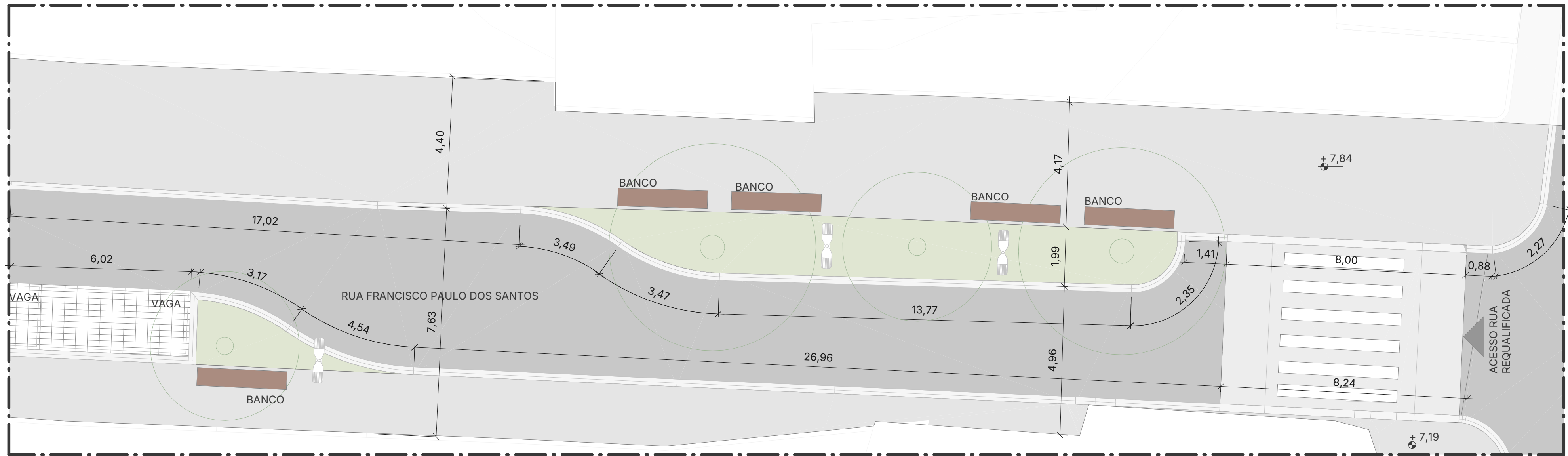
TRECHO 1 - PLANTA BAIXA RUA ESC: 1 : 100
