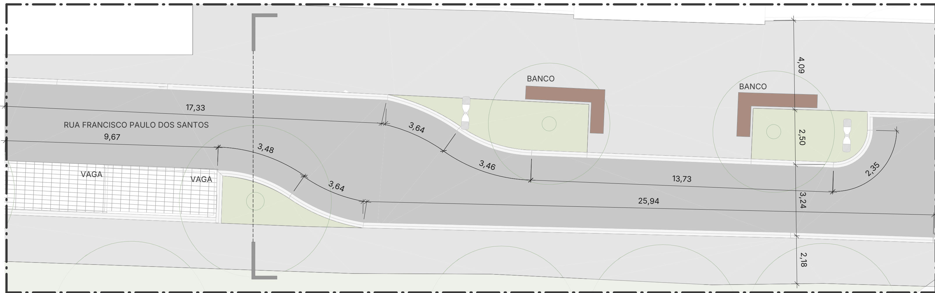
TRECHO 4 - PLANTA BAIXA RUA ESC: 1 : 100
