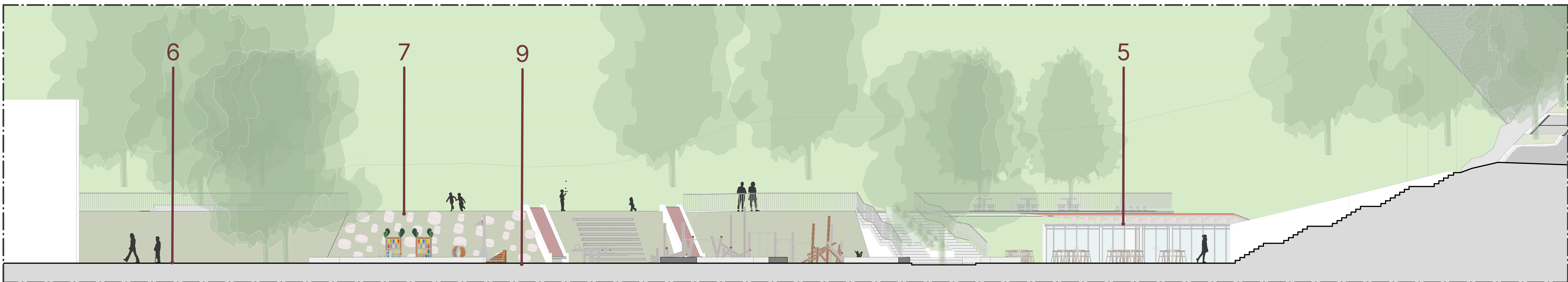
CORTE BB - PRAÇA ESC: 1:100
