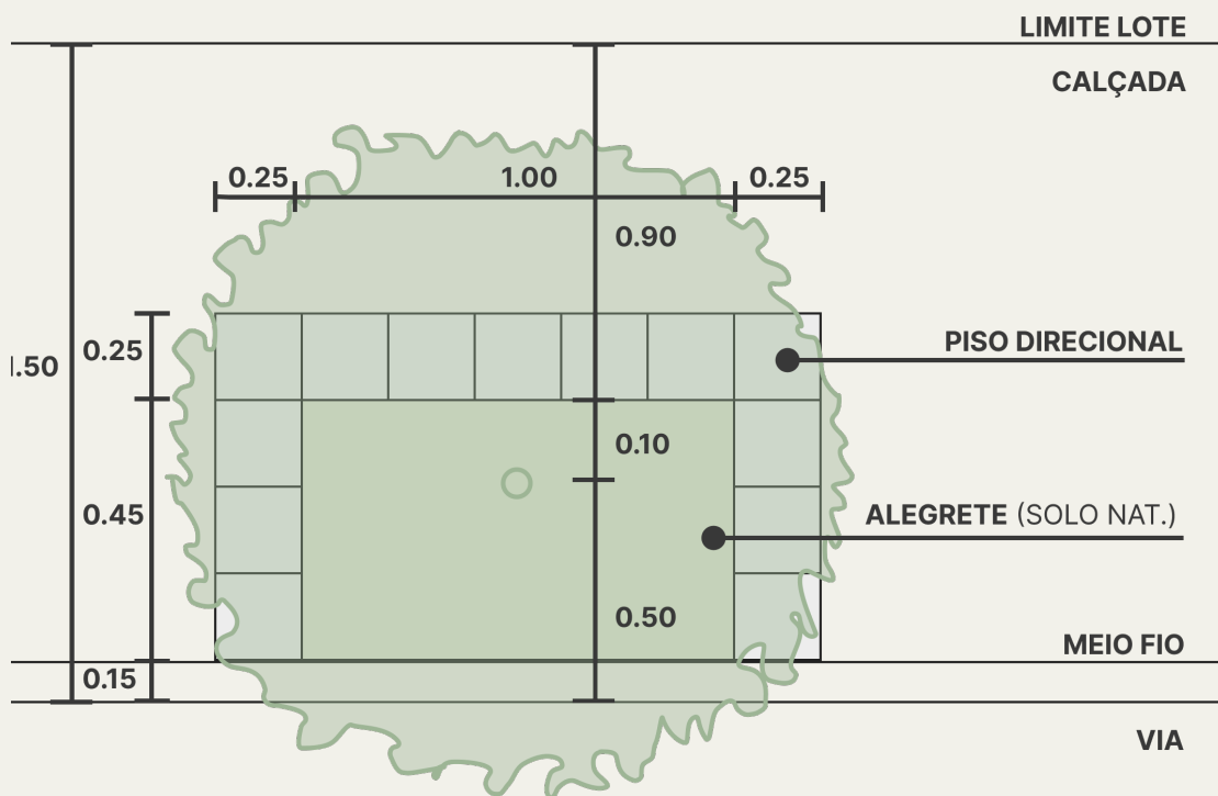
Figura 37 – Dimensionamento de alegretes em vias de 1,50m
