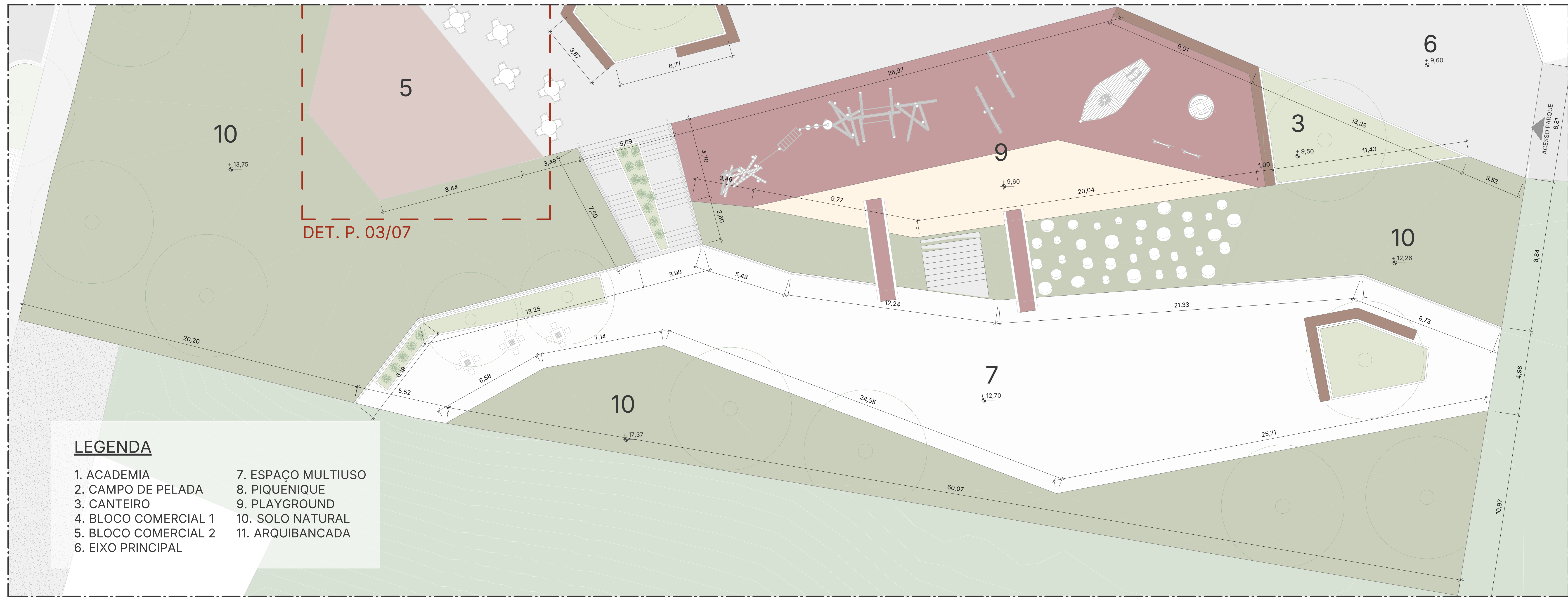
TRECHO 3 - PLANTA BAIXA PRAÇA ESC: 1: 100
