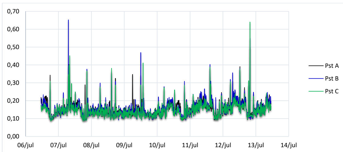
Figura 47 - Indicador Pst - Elev. Cortegadas
