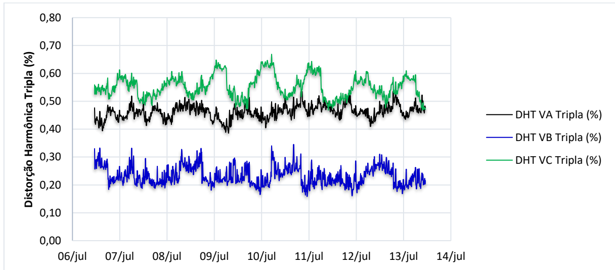
Figura 45 - DHT Tripla - Elevatória Cortegadas
