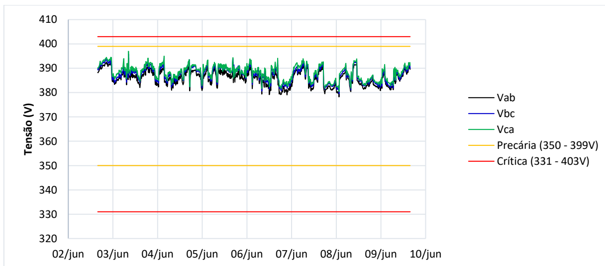
Figura 14 - TRP - Elevatória Totó
