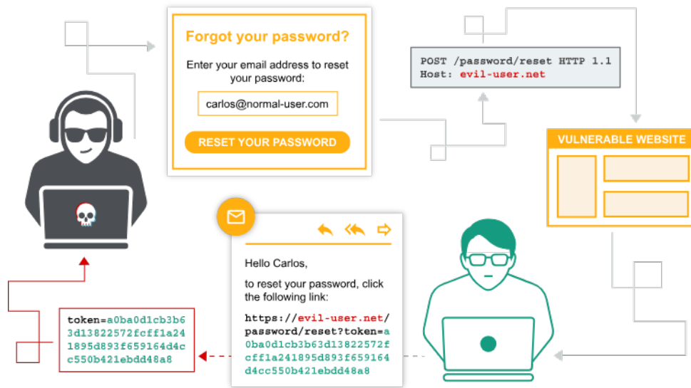
Figura 7: Autenticação inadequada. Fonte: https://portswigger.net/web-security/authentication
