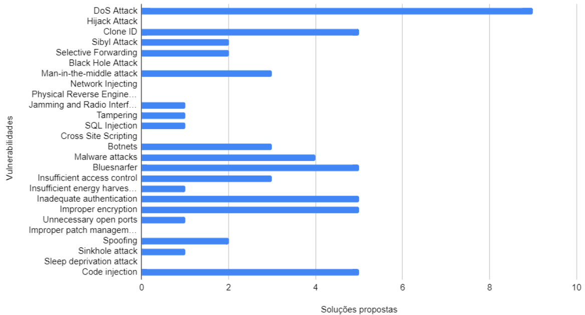
Figura 3: Soluções propostas para cada vulnerabilidade encontrada na literatura
