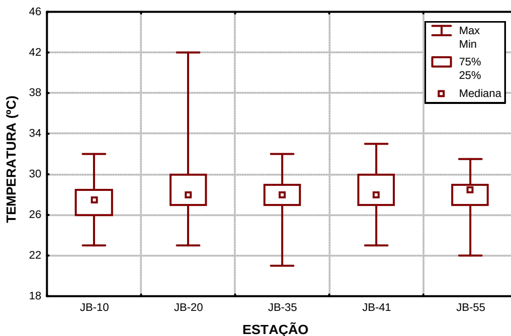
Figura 10 – Variação da temperatura ao longo do curso do rio Jaboatão no período de 1997- 2005.
