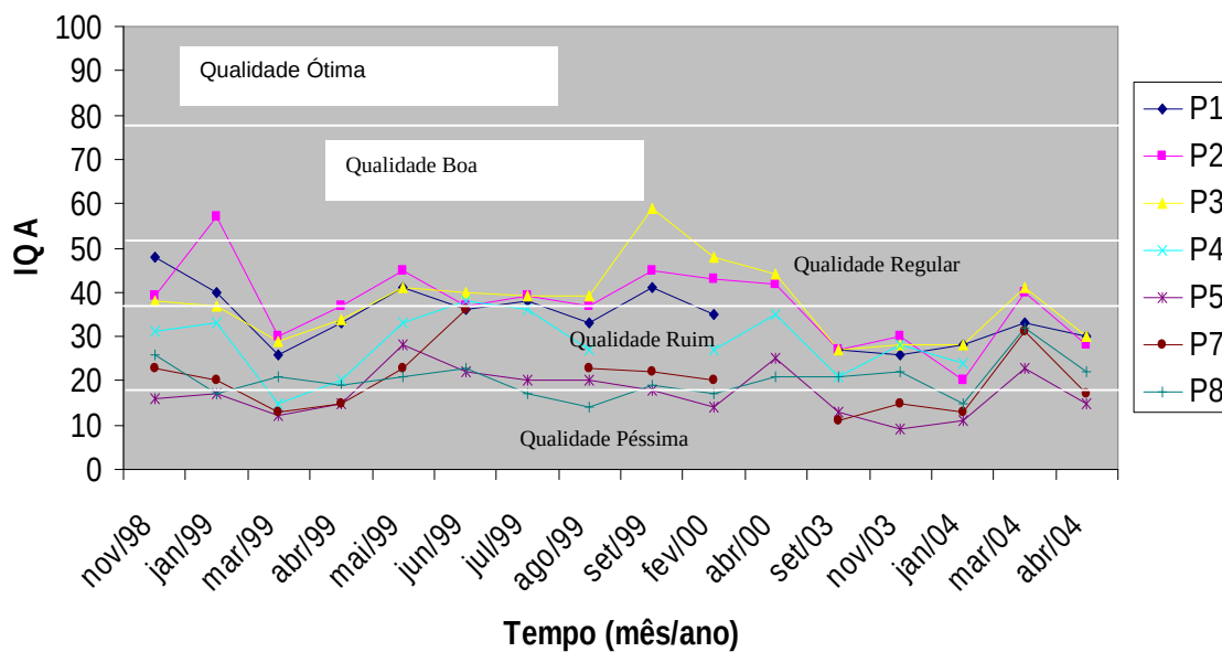
Figura 25 – Variação espacial e temporal do IQA no Rio Jaboatão.
