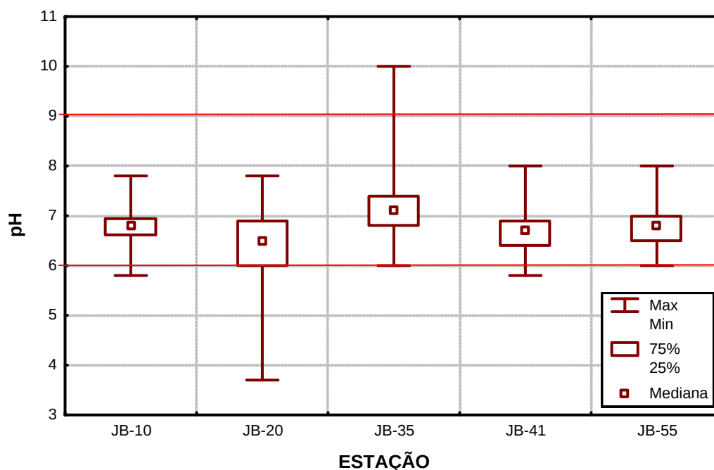
Figura 11 – Variação de pH ao longo do curso do rio Jaboatão no período de 1997- 2005.
