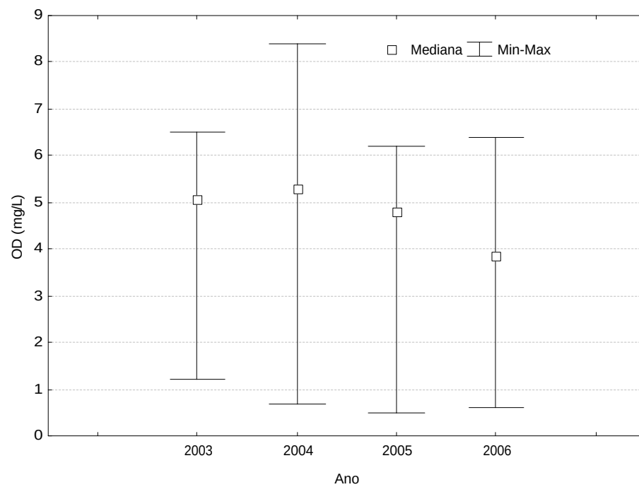
Figura 24 – Variação temporal de OD.
