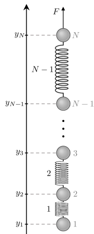
Figura 4: Sistema com N esferas de pequeno diâmetro e N - 1 molas de massa desprezível, inicialmente suspenso (em equilíbrio) pela aplicação de uma força \mathbf{F} na esfera mais acima.
