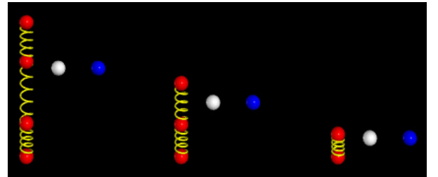
Figura 11: Imagens obtidas a partir de uma animação criada pelo programa em Python (sistema inicialmente com 6 partículas).
