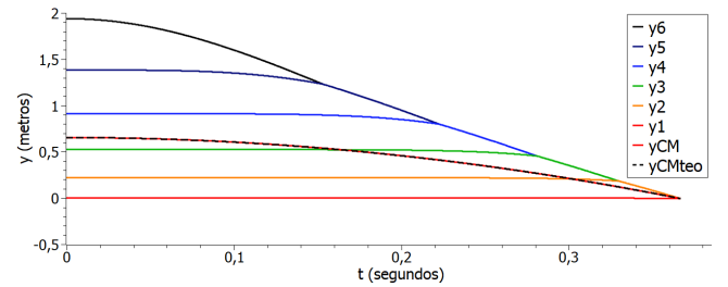
Figura 10: Gráficos a partir da tabela gerada pelo programa em C apresentado na Fig. 8.
