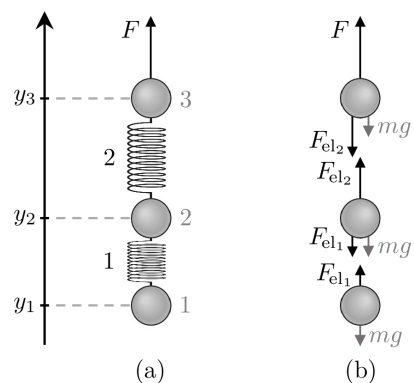
Figura 5: (a) Sistema com 3 pequenas esferas de massa m e 2 molas de massa desprezível, inicialmente suspenso (em equilíbrio) pela aplicação de uma força \mathbf{F} na esfera mais acima. (b) Diagramas de forças para as três esferas, na situação de equilíbrio.
