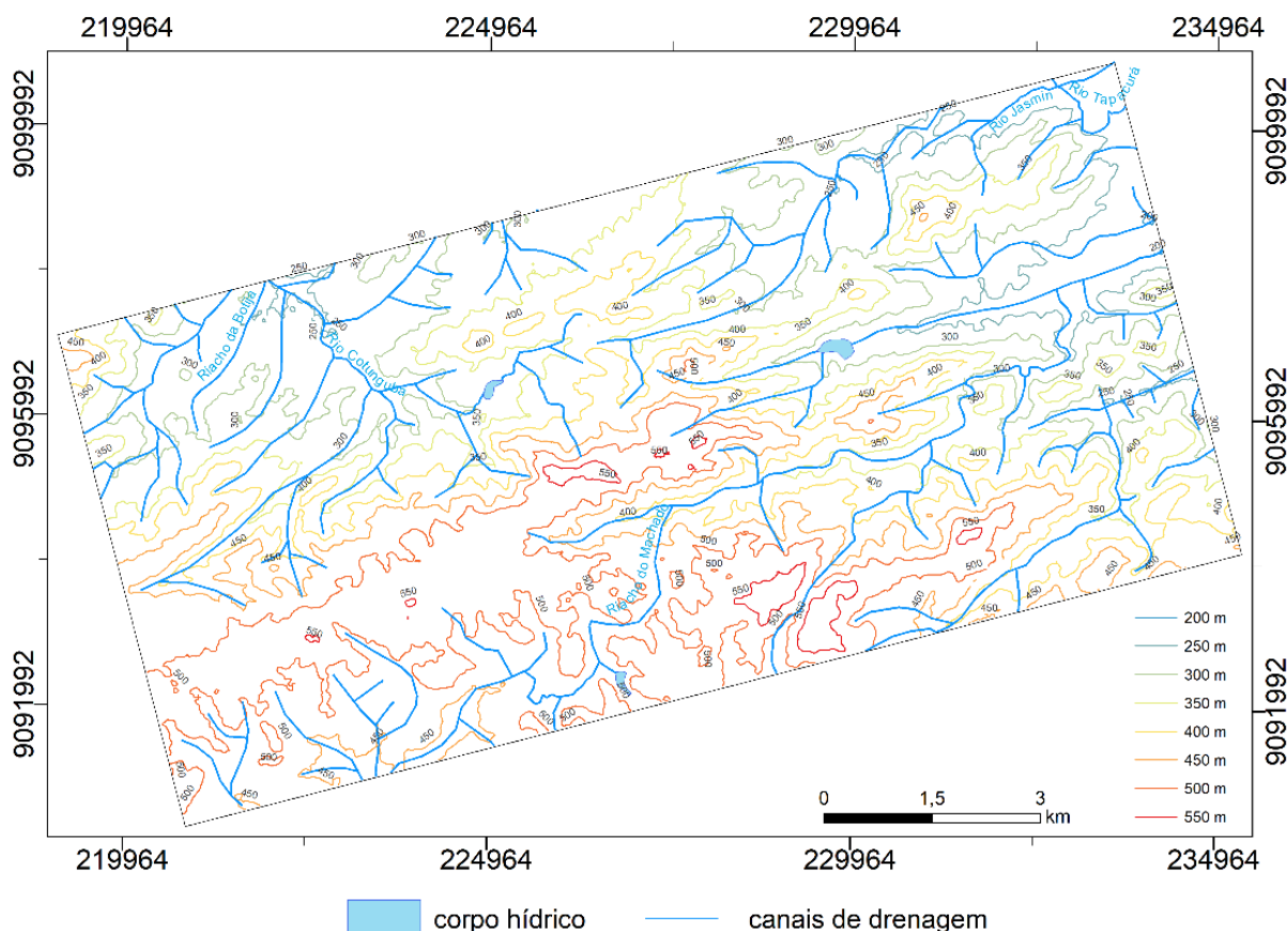
Figura 12: Mapa de rede de drenagem interpretada e curvas de nível da região na área de estudo
