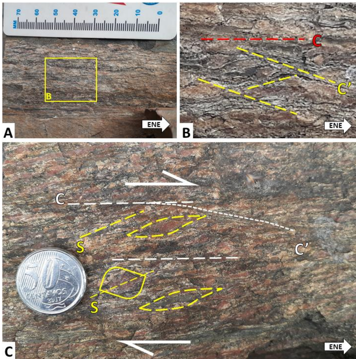
Figura 29 - Fotografia dos indicadores cinemáticos da ZCPE
