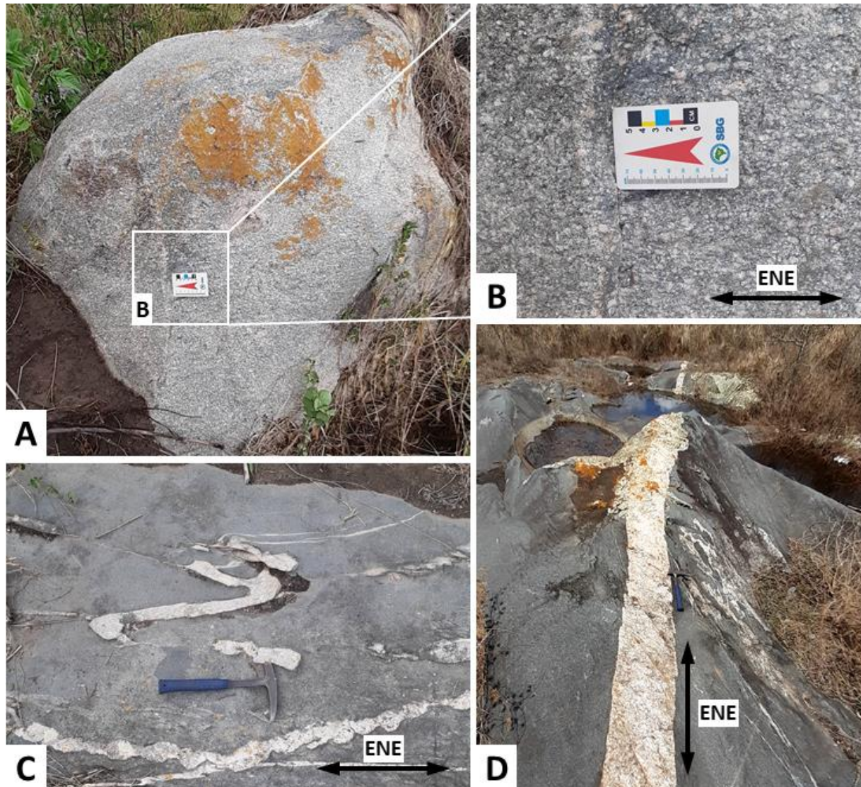
Figura 23 - Fotografias dos afloramentos dos granitoides sintranscorrentes tipo 1
