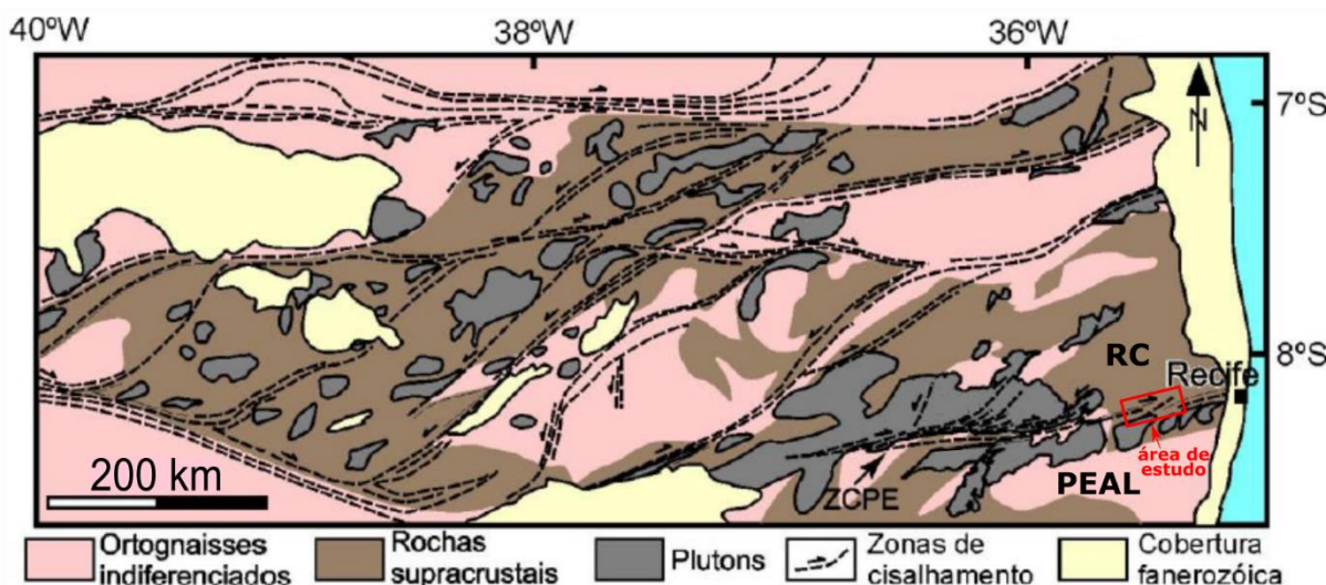
Figura 4 - Mapa geológico simplificado das subprovíncias central e sul (porção nordeste) da Província Borborema
