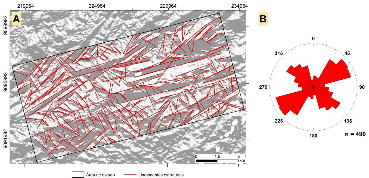
Figura 14: Lineamentos identificados sobreposto ao MDE de iluminação 0Az (A), com as direções preferenciais interpretadas em diagrama de roseta (B)
