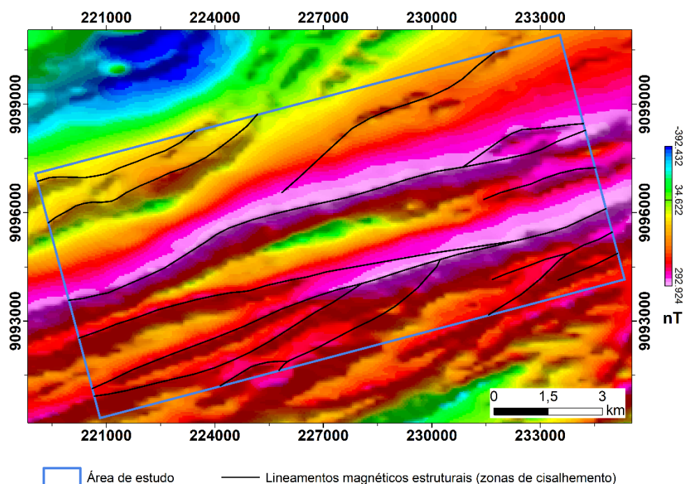
Figura 9 - Padrão anastomosado dos lineamentos magnéticos estruturais interpretados a partir da imagem do campo magnético anômalo
