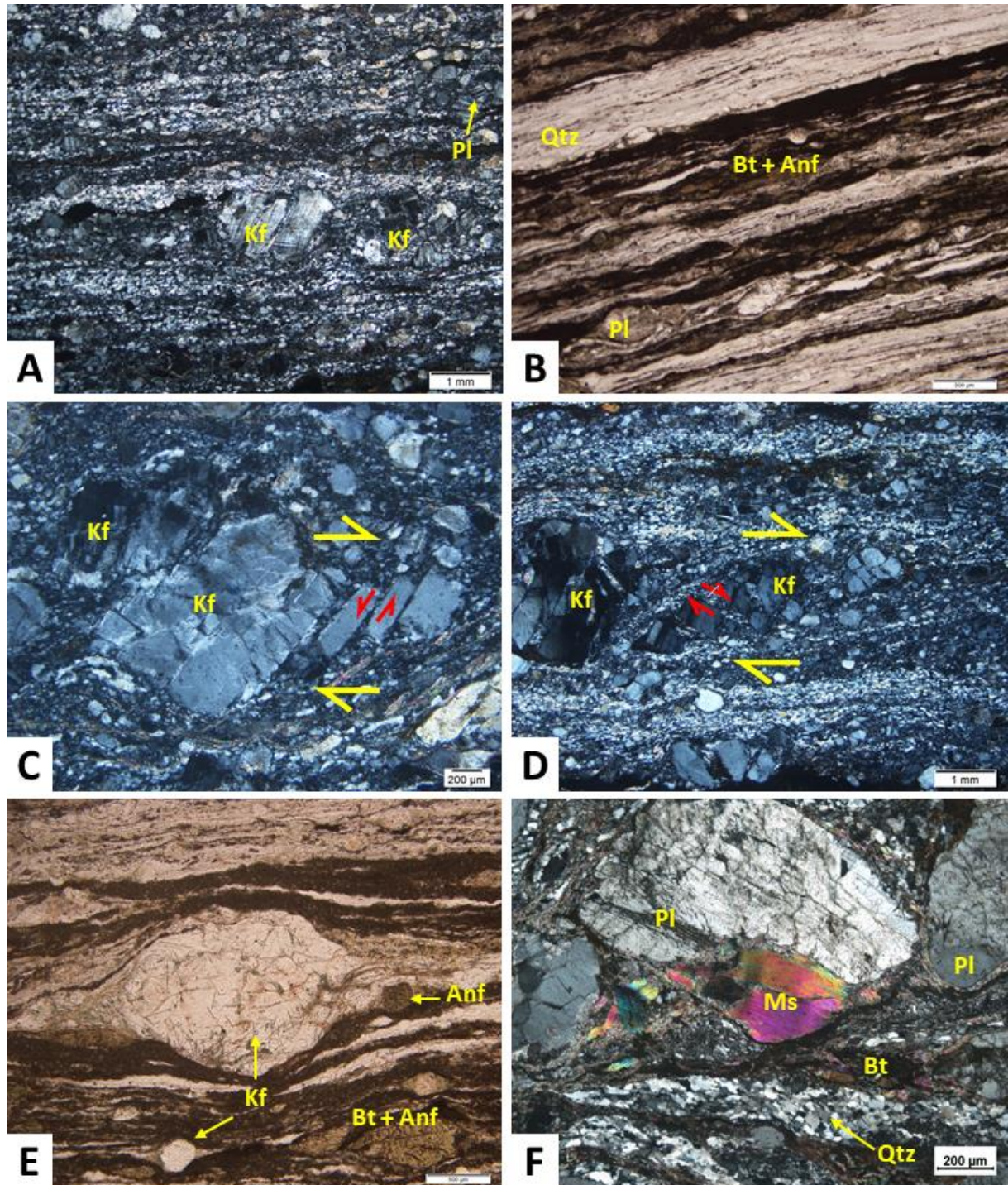
Figura 20 - Fotomicrografia dos ultramilonitos bandados (porção norte da ZCPE) da faixa milonítica
