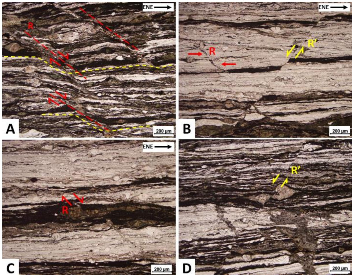
Figura 40 - Fotomicrografia ilustrando as microfalhas R (destal) e R' (sinistral) presentes nos ultramilonitos bandados da ZCPE (SR02)
