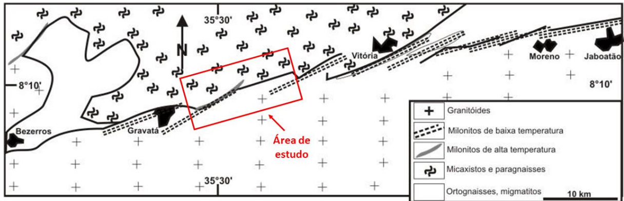
Figura 5 - Mapa esquemático exibindo a geometria de recobrimento à direita para a ZCPE
