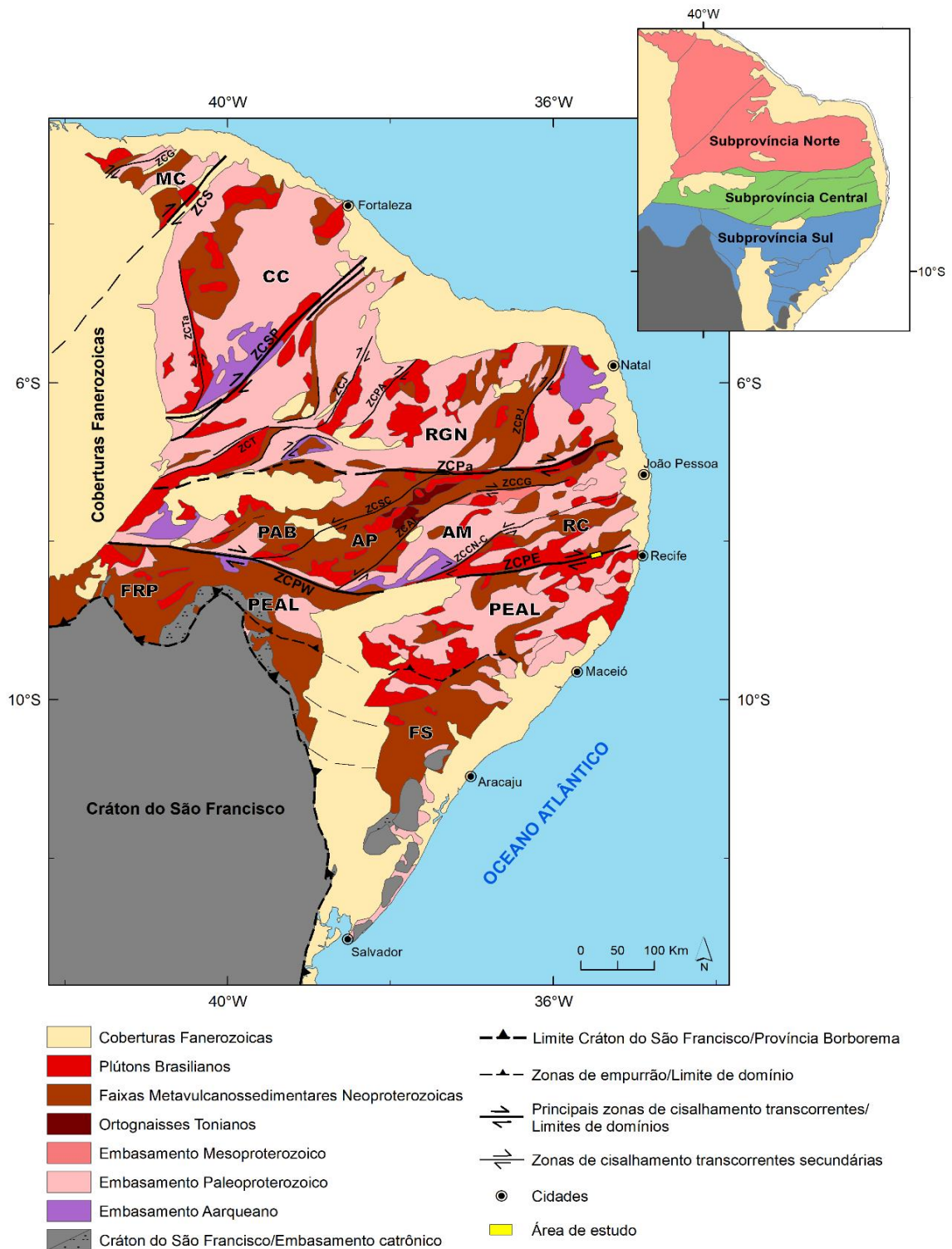
Figura 3 - Mapa geológico simplificado da Província Borborema
