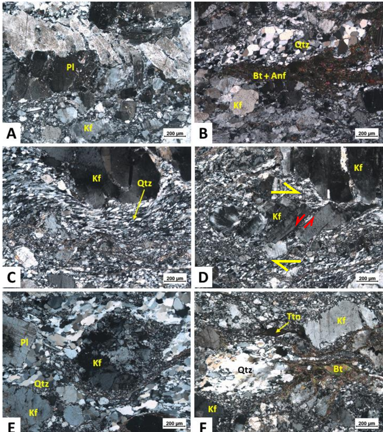
Figura 22 - Fotomicrografia dos milonitos graníticos (porção sul da ZCPE)
