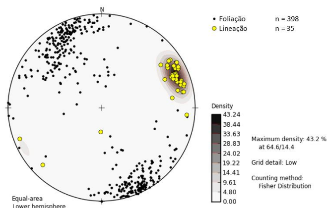
Figura 28 - Estereograma de polos das foliações e lineações da área de estudo.
