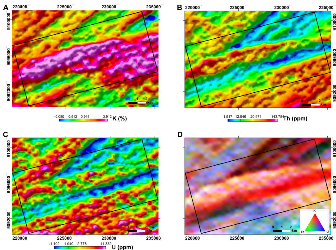
Figura 6 - Imagens obtidas por aerogamaespectrometria da área de estudo
