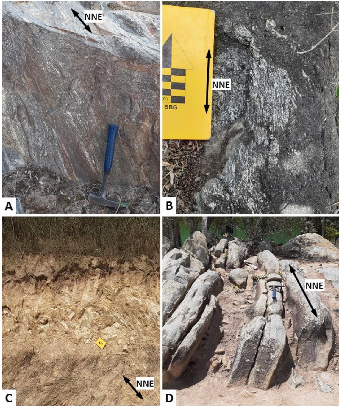
Figura 16: Fotografias dos afloramentos dos paragneisses do Complexo Surubim-Caroalina
