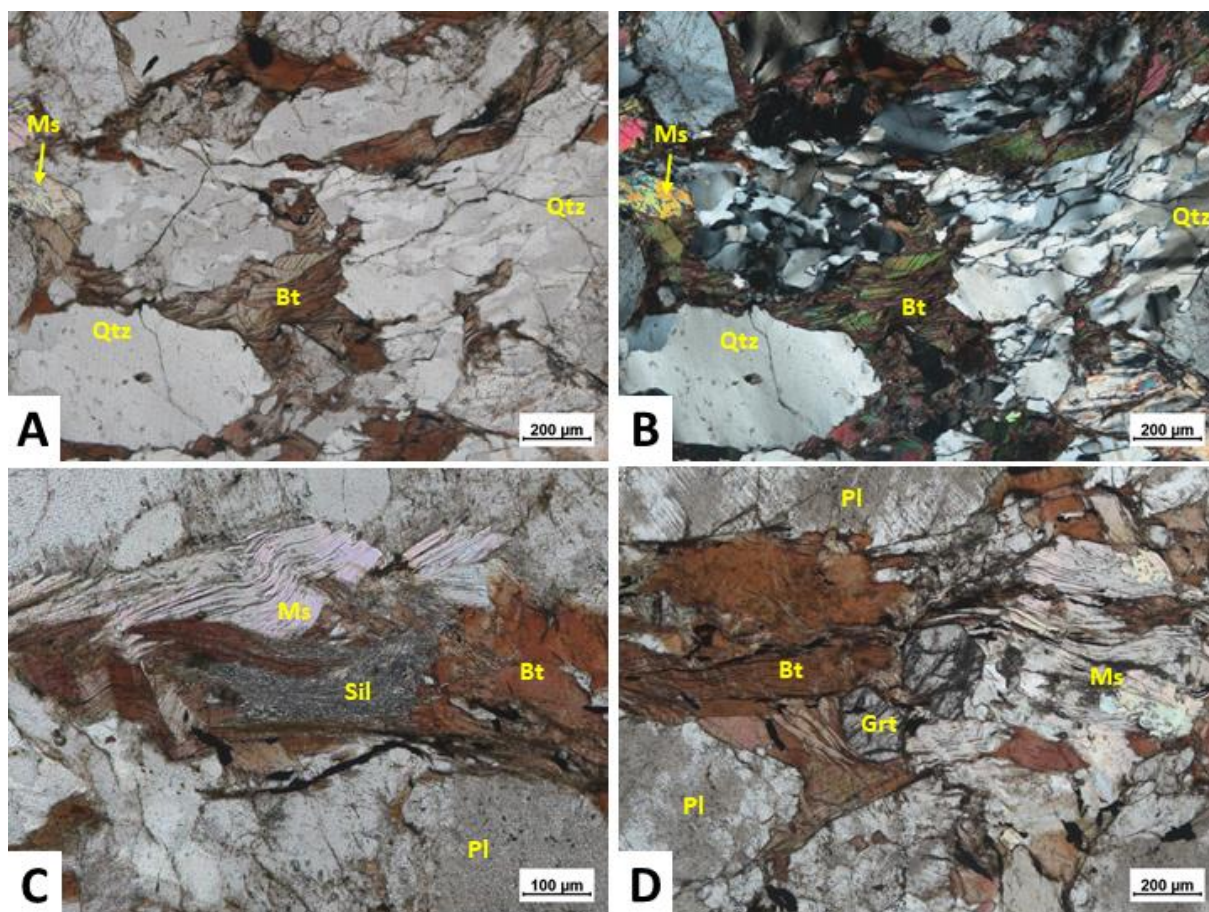
Figura 18: Fotomicrografia das lâminas delgadas das rochas metassedimentares com textura lepidogranoblástica (LFM38)
