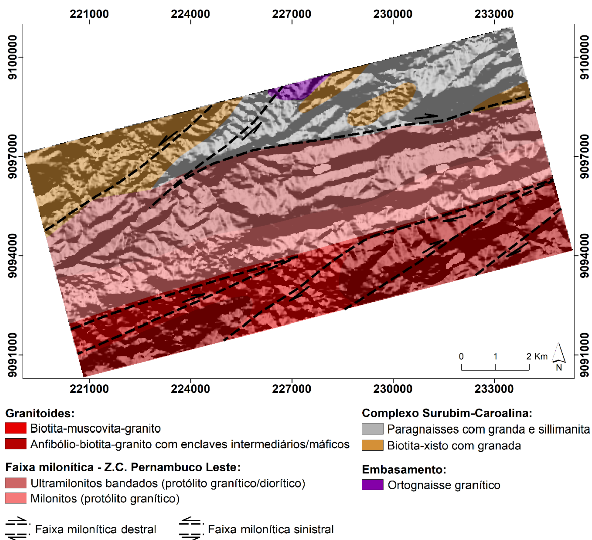
Figura 15: Mapa geológico-estrutural simplificado sobreposto ao MDE
