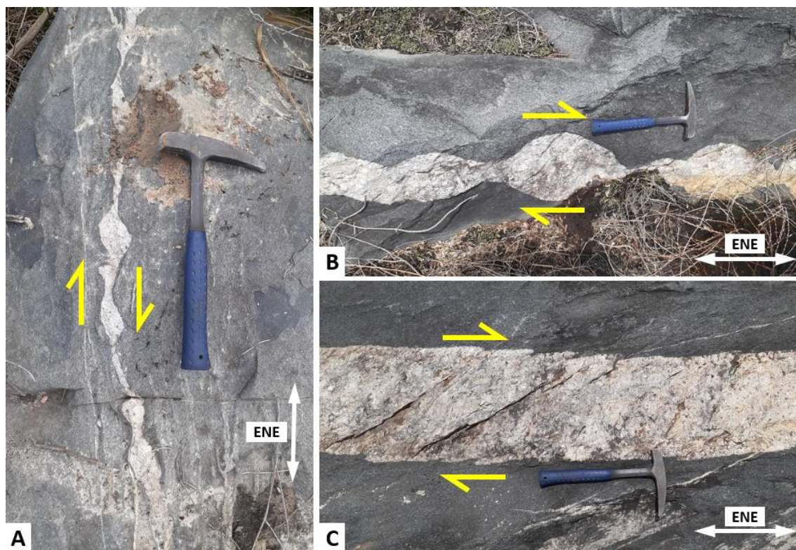
Figura 33 - Diques pegmatíticos deformados
