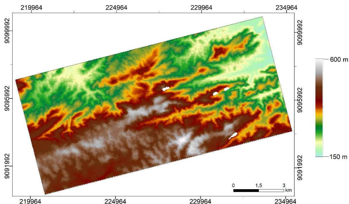
Figura 11: Imagem MDE (SRTM), com resolução espacial de 30m, da área de estudo utilizada para interpretação de rede de drenagem e estruturas
