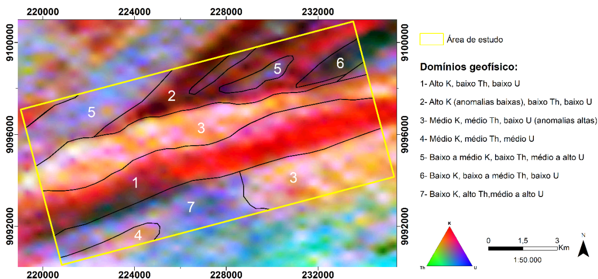
Figura 7 - Domínios gamaespectrométricos individualizados na área de estudo
