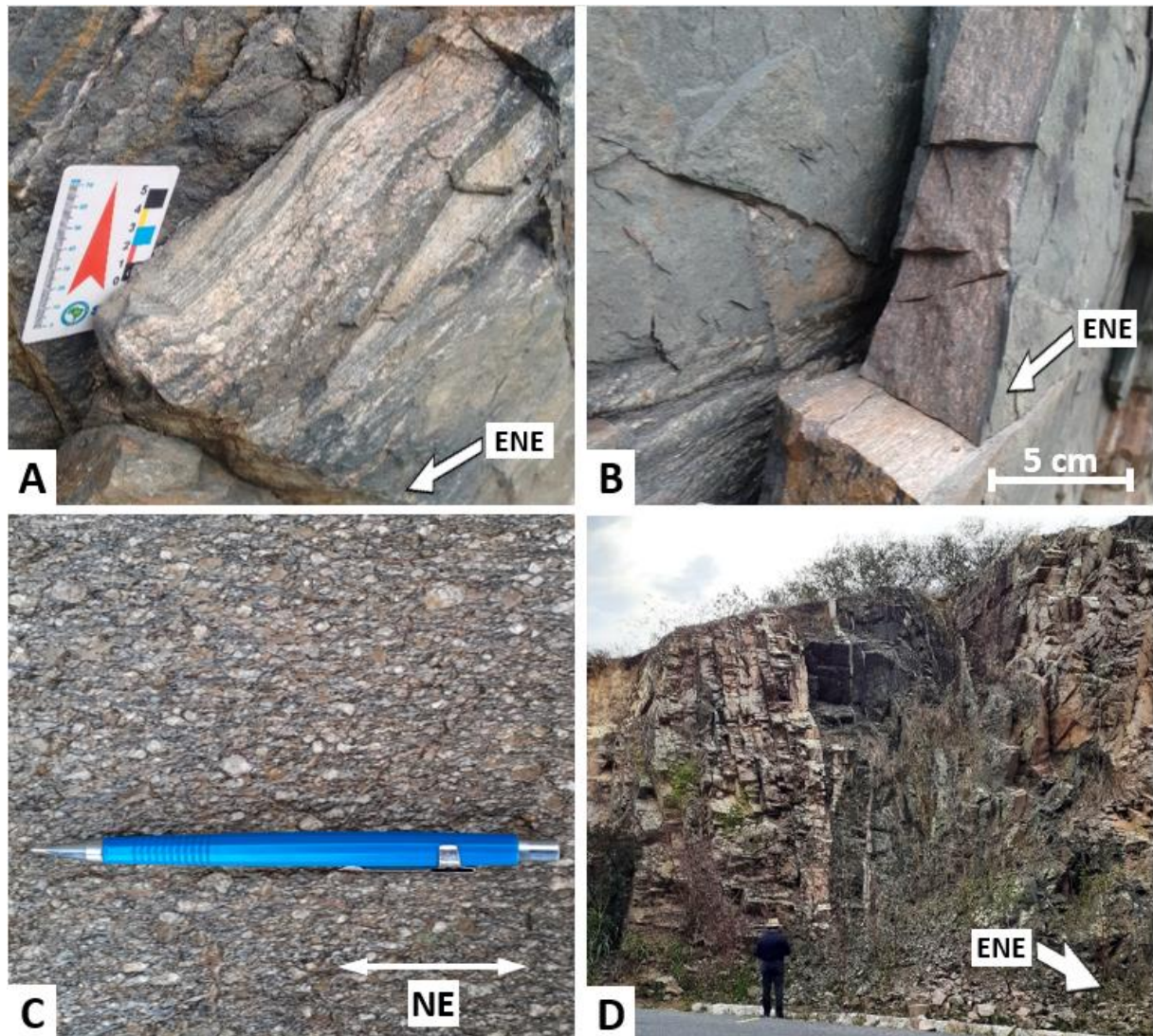
Figura 19: Fotografias dos afloramentos dos milonitos/ultramilonitos bandados (porção norte da ZCPE)
