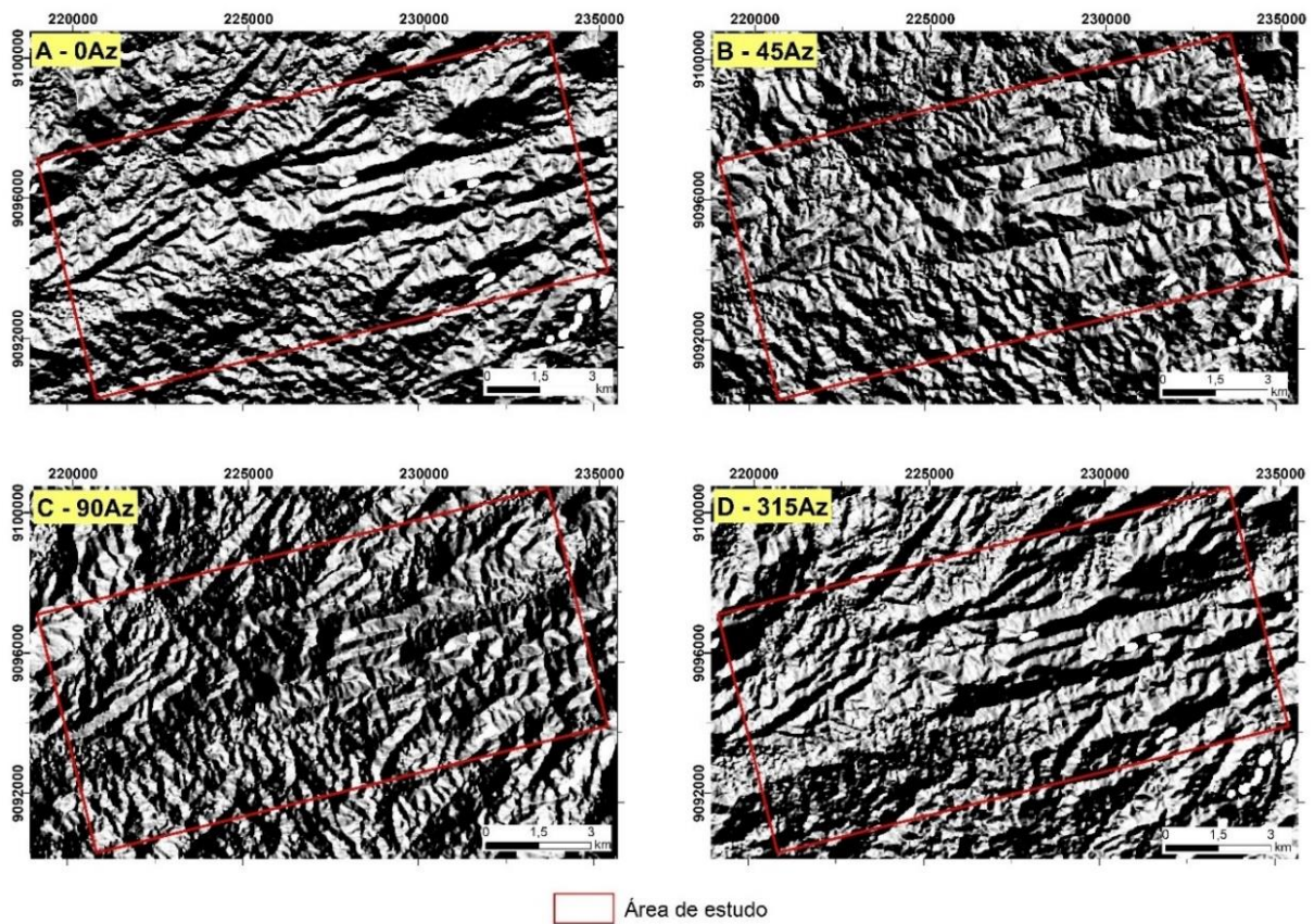
Figura 13: Imagens MDE com efeitos de iluminações nas direções 0Az (A), 45Az (B), 90Az (C) e 315Az (D), utilizadas para interpretação de lineamentos estruturais
