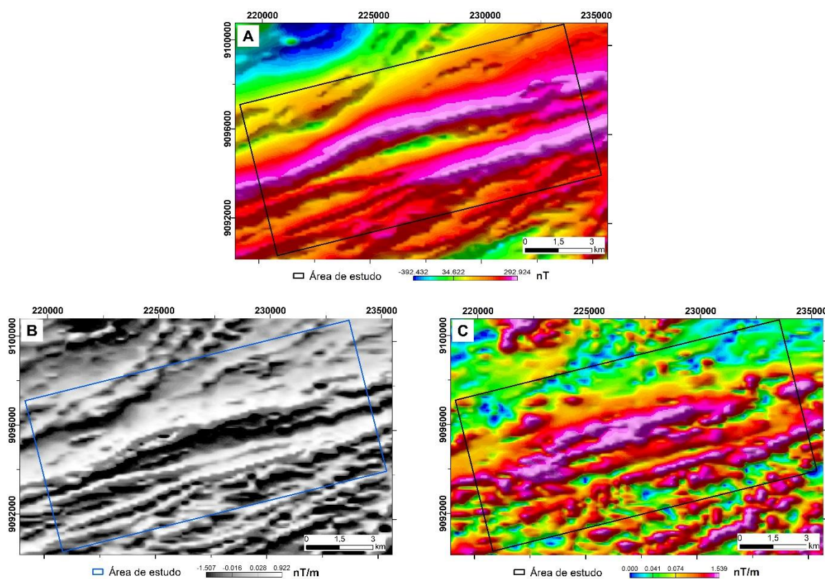
Figura 8 - Imagens obtidas por aeromagnetometria da área de estudo
