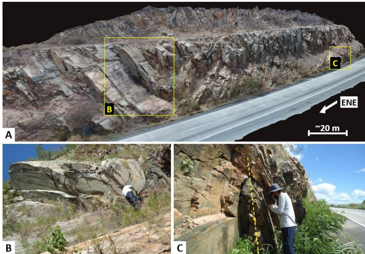
Figura 30 - Fotografias das dobras antiformes e sinformes nos ultramilonitos da Serra das Russas, Gravatá – PE (SR01)
