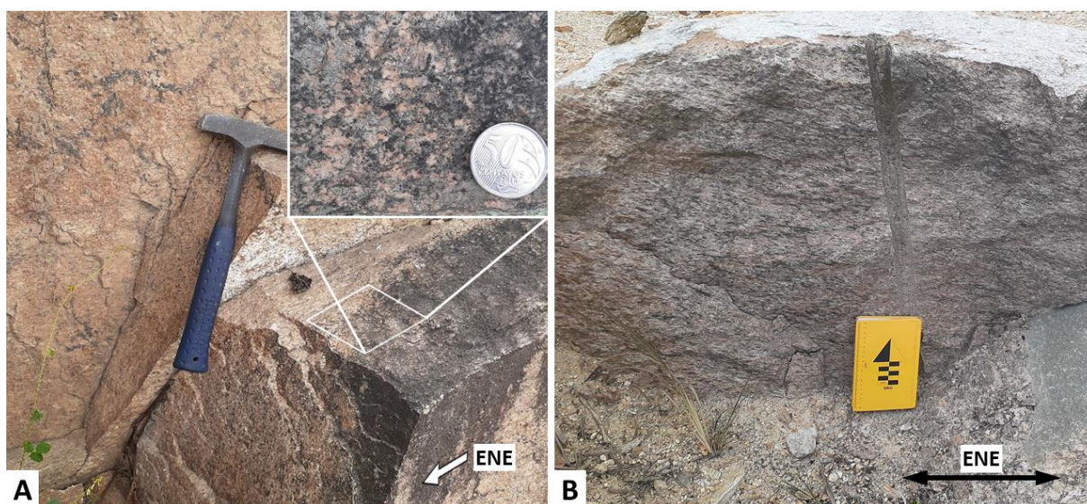
Figura 21 - Fotografias dos afloramentos miloníticos de protólito granítico (porção sul da ZCPE)
