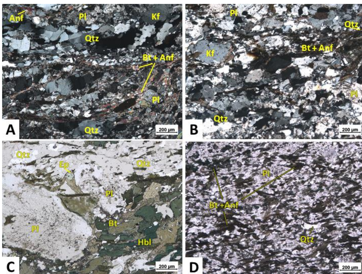
Figura 24 - Fotomicrografia das amostras dos granitoides tipo 1
