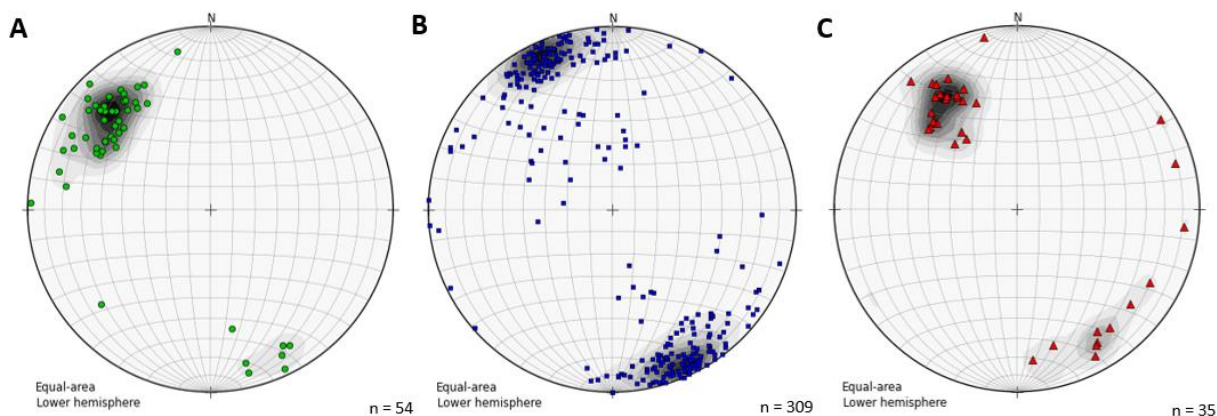
Figura 27 - Projeções estereográficas dos polos das foliações das unidades litológicas
