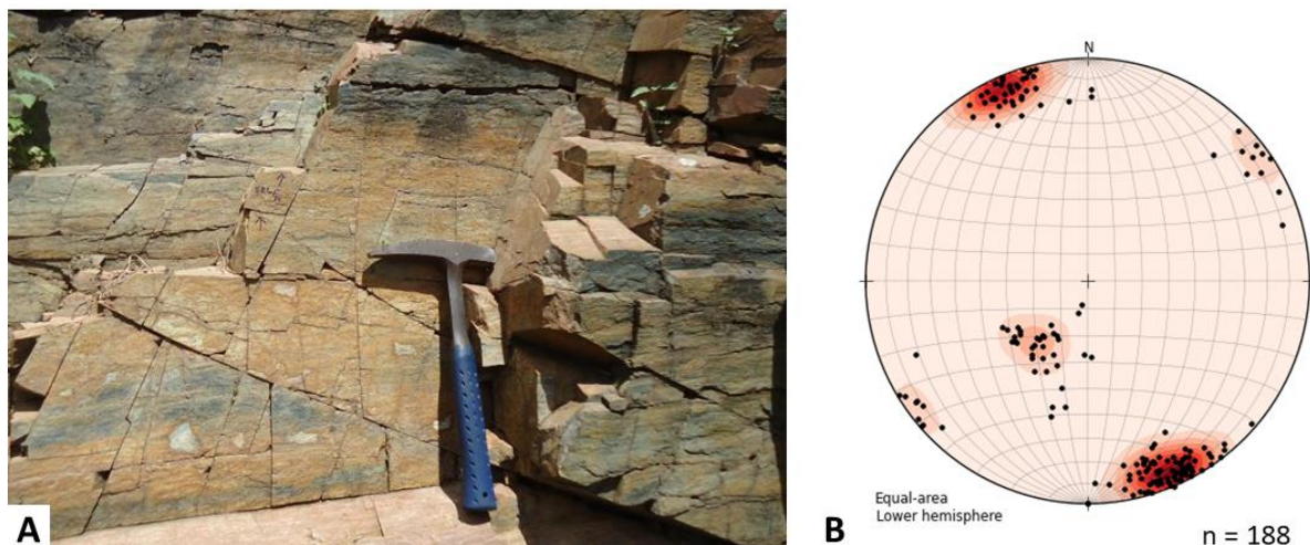
Figura 37 - Sistema de fraturas da área de estudo
