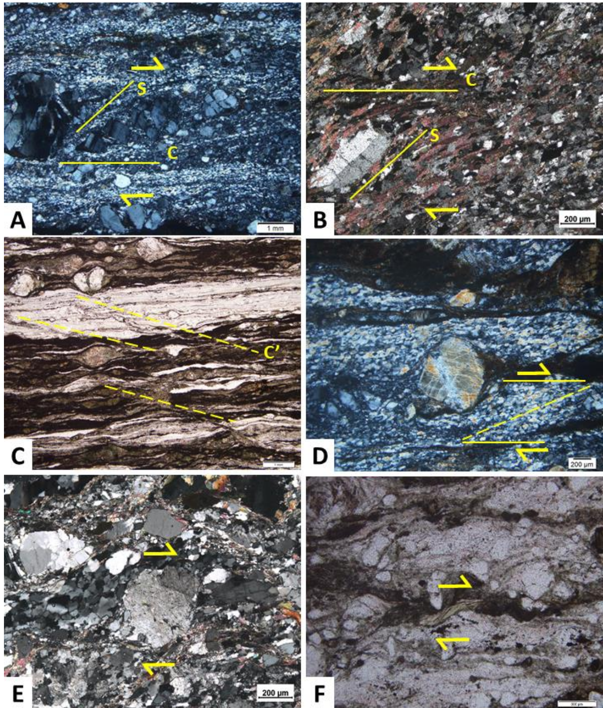
Figura 38 - Fotomicrografias ilustrando os critérios cinemáticos da tectônica transcorrente destrai regional (ZCPE)
