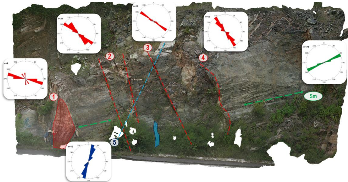
Figura 35 - Ortofotografia em perfil do afloramento-chave dos ultramilonitos bandados contendo o sistema de falhas, localizado na Serra das Russas (SR02)
