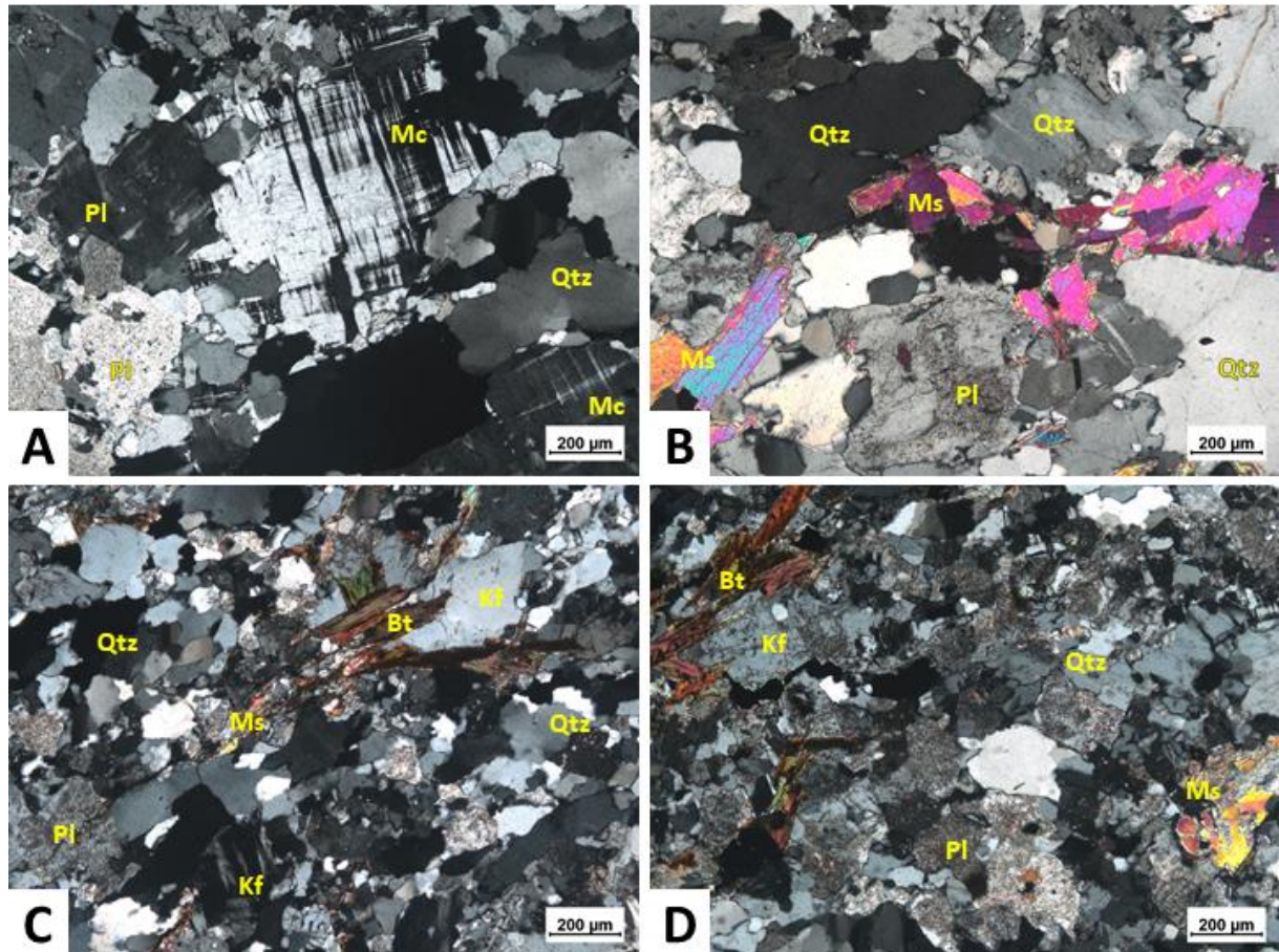
Figura 26 - Fotomicrografia das amostras dos granitoides tipo 2
