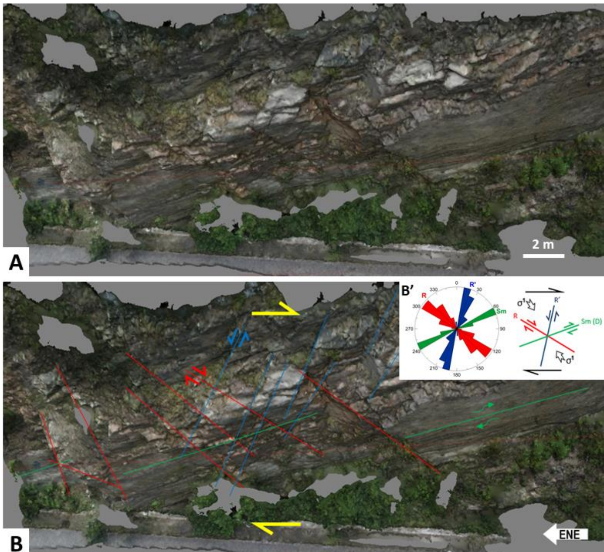
Figura 36 - Ortofotografia em planta do afloramento-chave dos ultramilonitos bandados contendo o sistema de falhas, localizado na denominada Serra das Russas (SR02)
