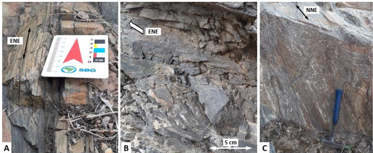
Figura 32 - Dobras intrafoliais
