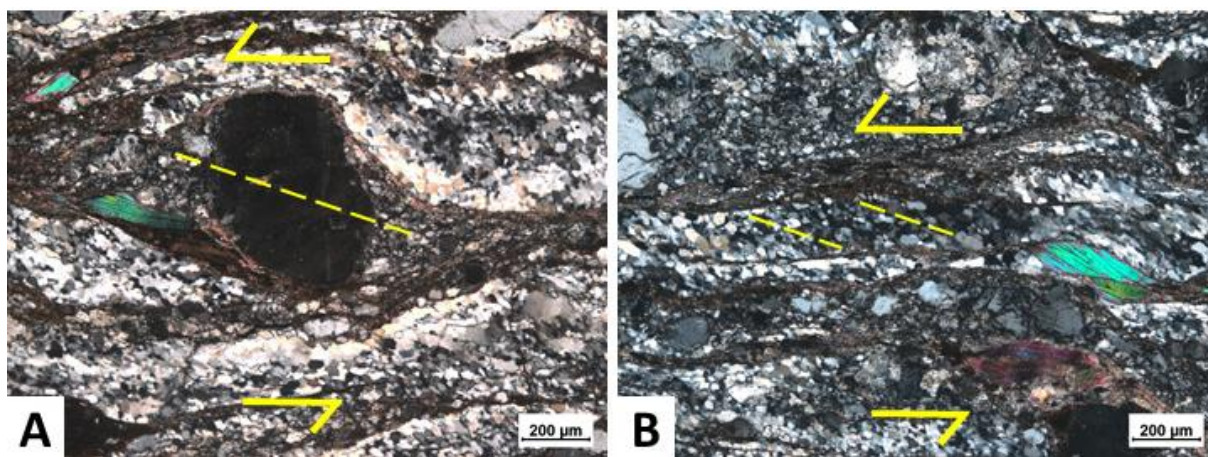
Figura 39 - Fotomicrografias ilustrando os critérios cinemáticos da zona de cisalhamento sinistral
