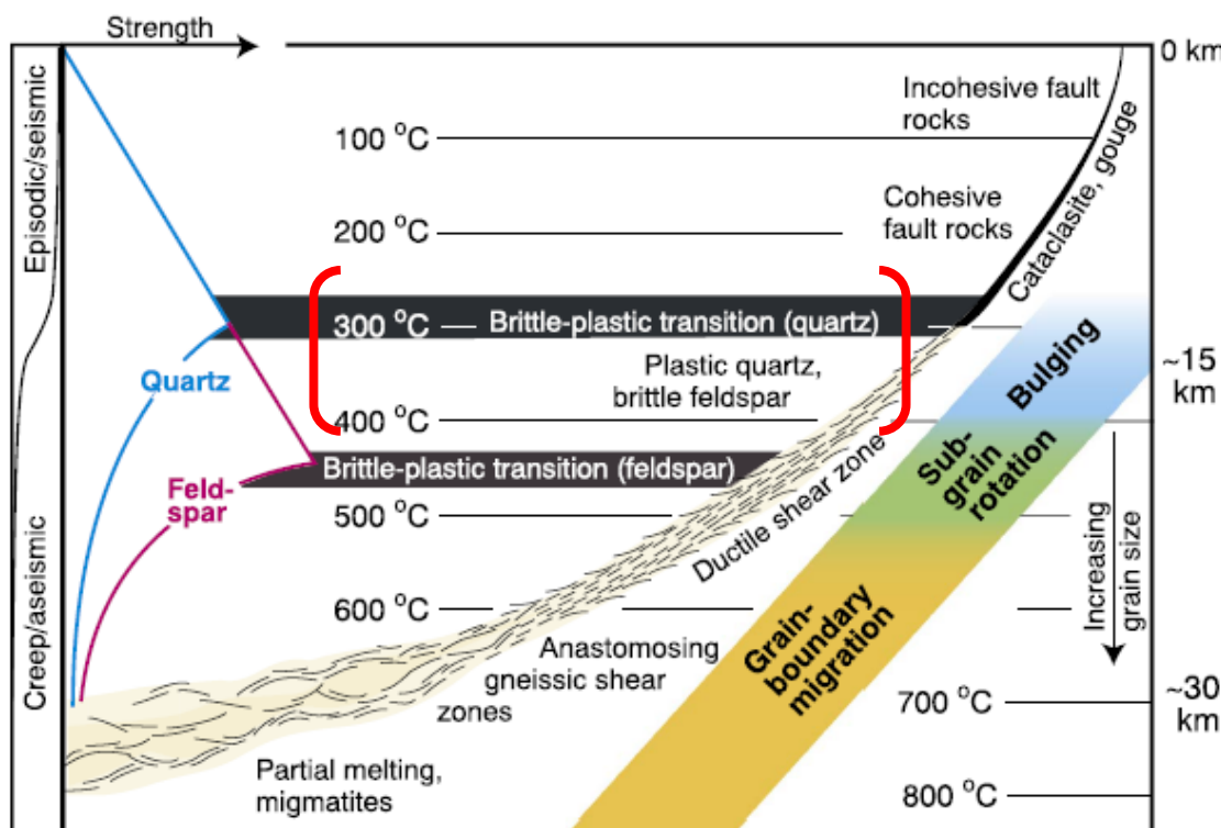
Figura 42 - Diagrama simplificado ilustrando a variação vertical de deformação em zonas de cisalhamento
