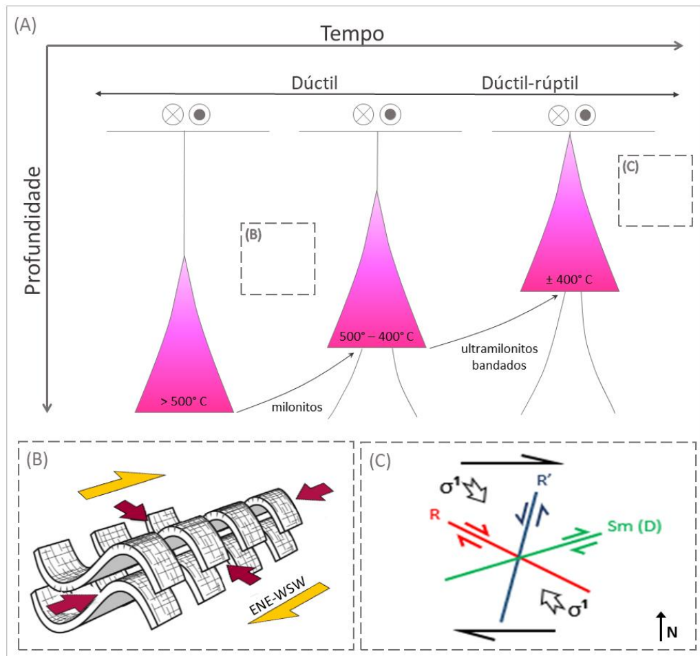
Figura 43 - Modelo de evolução esquemático da Zona de Cisalhamento Pernambuco Leste
