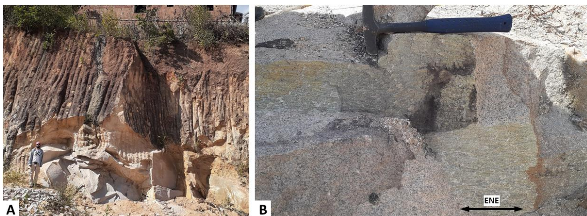
Figura 25 - Fotografias dos afloramentos dos granitoides sintranscorrentes tipo 2
