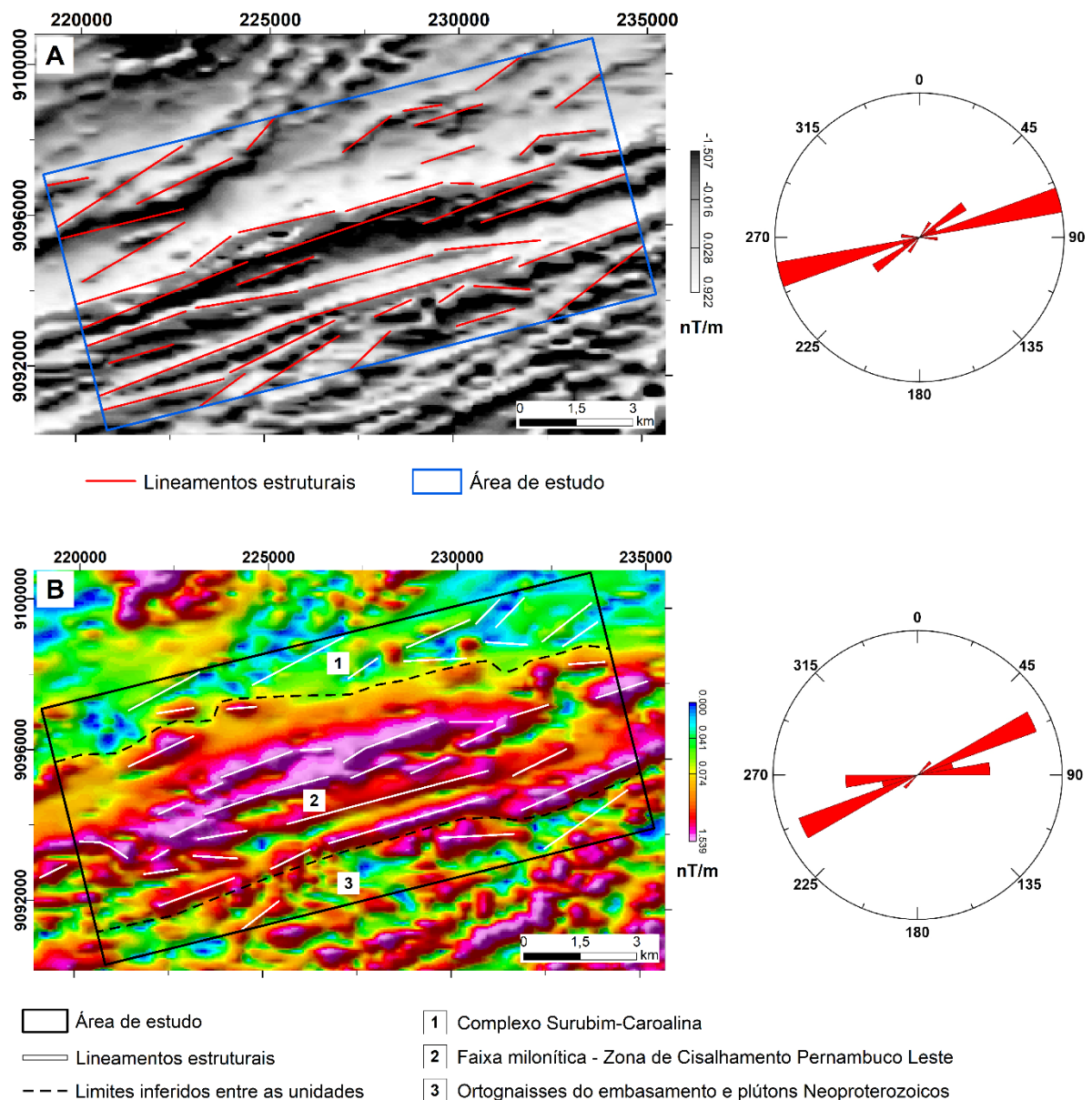
Figura 10 – A: Lineamentos magnéticos estruturais interpretados a partir da imagem da primeira derivada vertical; B – Lineamentos magnéticos estruturais e zonas litológicas interpretados a partir da imagem da amplitude de sinal analítico
