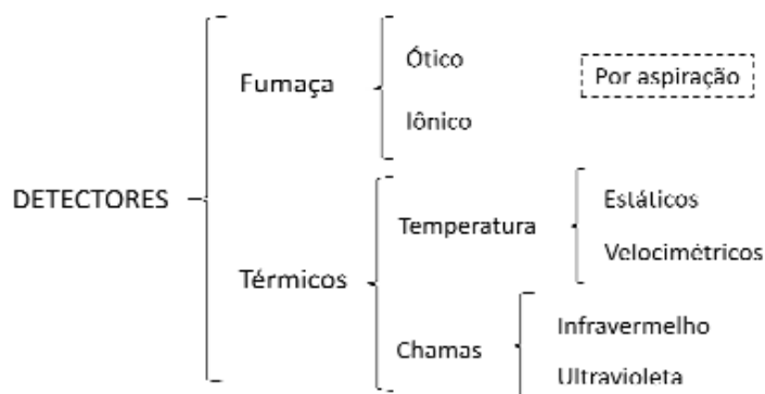
FIGURA 08 -Tipos de Detectores
