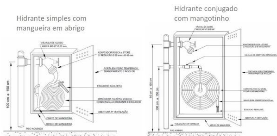
FIGURA 09 – Exemplos de sistema composto por hidrante.
