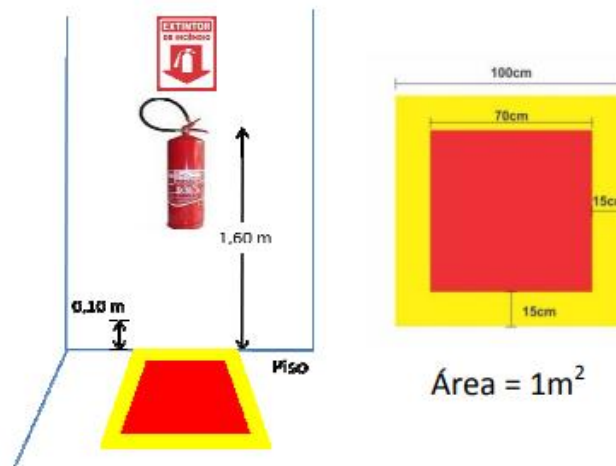
FIGURA 10 - Demarcação dos extintores
