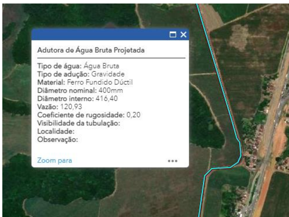
Figura 19 - Recorte da adutora de água bruta projetada para o SAA do município de Goiana
