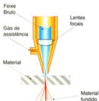
Figura 12 - Corte a laser - Fonte: Industria, 2016.
