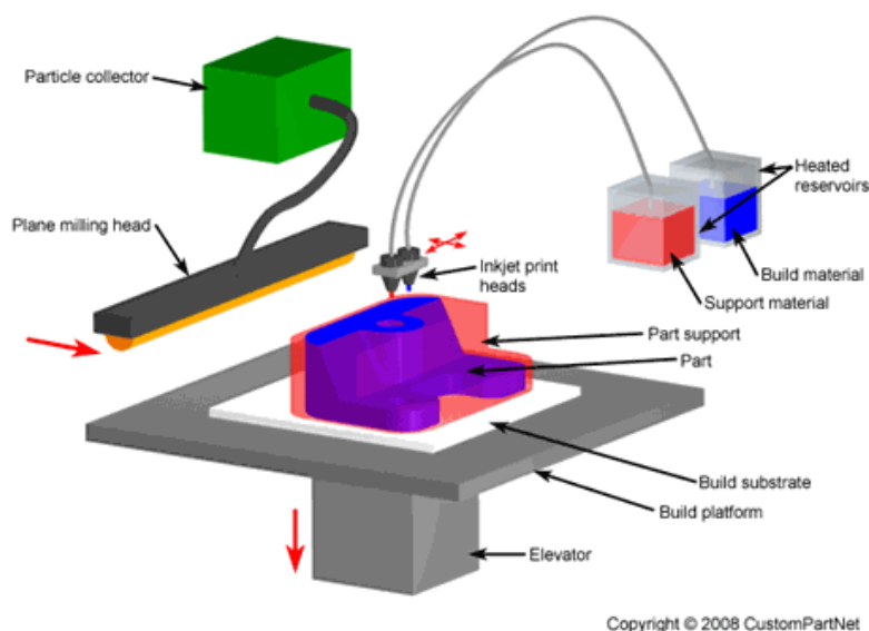
Figura 28 - Processo de conformação por MJT - Fonte: CUSTOMPARTNERT, 2015.
