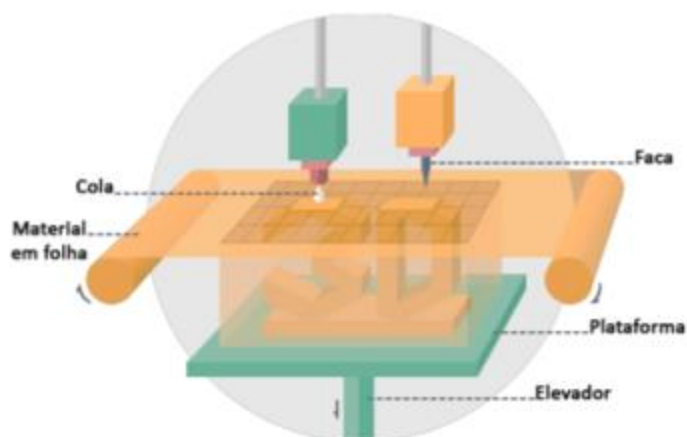
Figura 19 - Processo da impressão LOM - Fonte: THRE3D, 2014.
