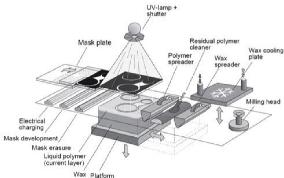
Figura 26 - Processo de conformação por SGC - Fonte: Upload, 2015.
