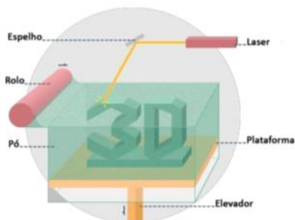
Figura 20 - Conformação em SLS - Fonte: THRE3D, 2014
