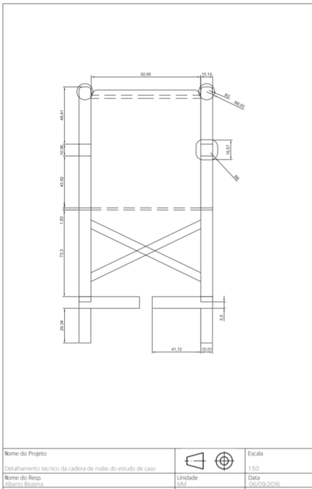
Figura 68 - Vista frontal da cadeira de roda - Fonte: o autor
