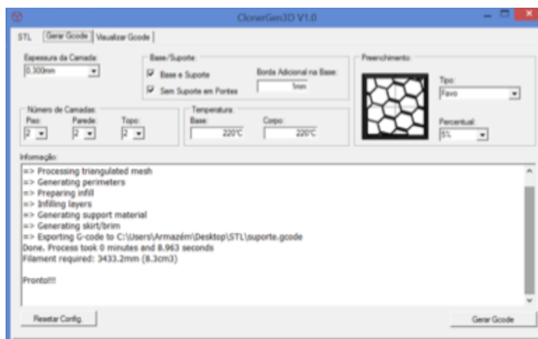
Figura 56 - Configuração para impressão das peças - Fonte: o autor.
