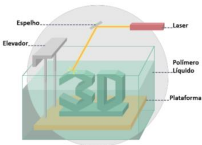
Figura 24 - Conformação por SLA - Fonte: THRE3D, 2014
