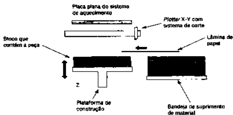
Figura 31 - Conformação em PLT - Fonte: VOLPATO et al, 2007
