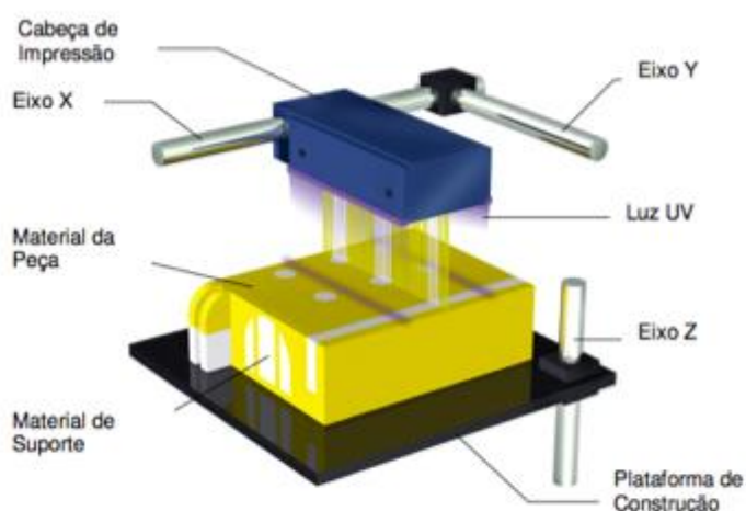
Figura 29 - Processo de conformação em IJP - Fonte: Volpato, 2007
