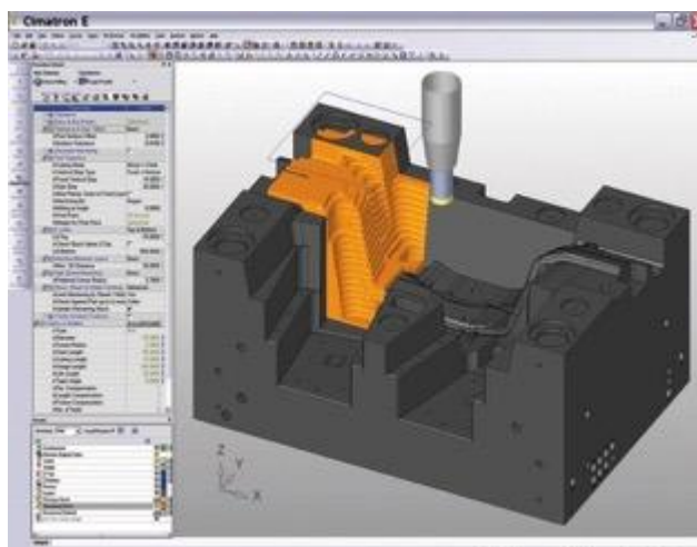
Figura 10 - Software CAD/CAM - Fonte: Plastico, 2015.
