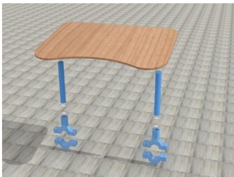
Figura 53 - Vista explodida do modelo - Fonte: o autor.
