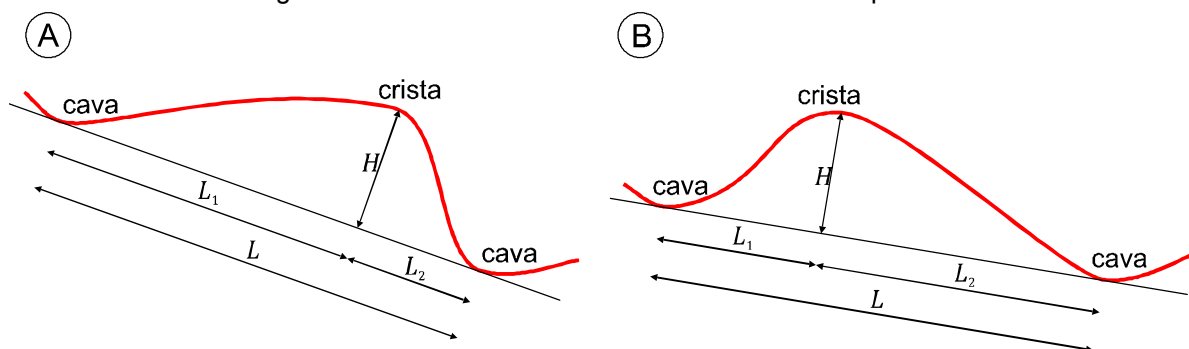
Figura 5: Parâmetros dimensionais das dunas subaquosas.
