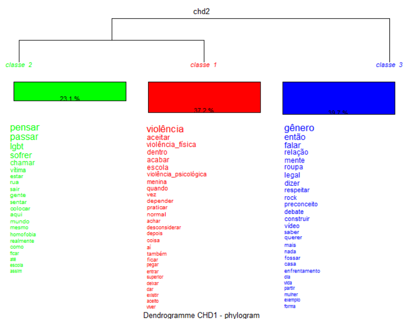
Figura 5 - Dendograma 1 com definição de classes (Recife, 2017)
