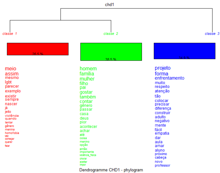
Figura 14 - Dendograma 2 com definição de classes (Recife, 2017)
