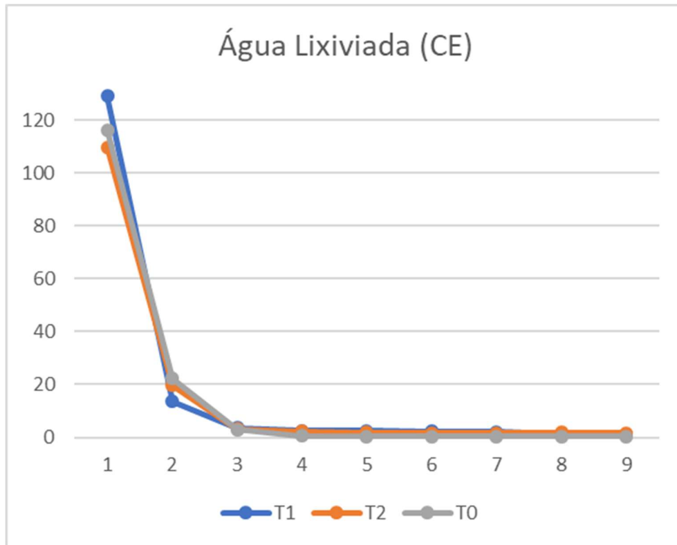
Gráfico 11 - Solo 6 – Condutividade elétrica da água lixiviada
