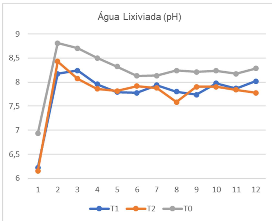
Gráfico 10– pH da água lixiviada do Solo 5
