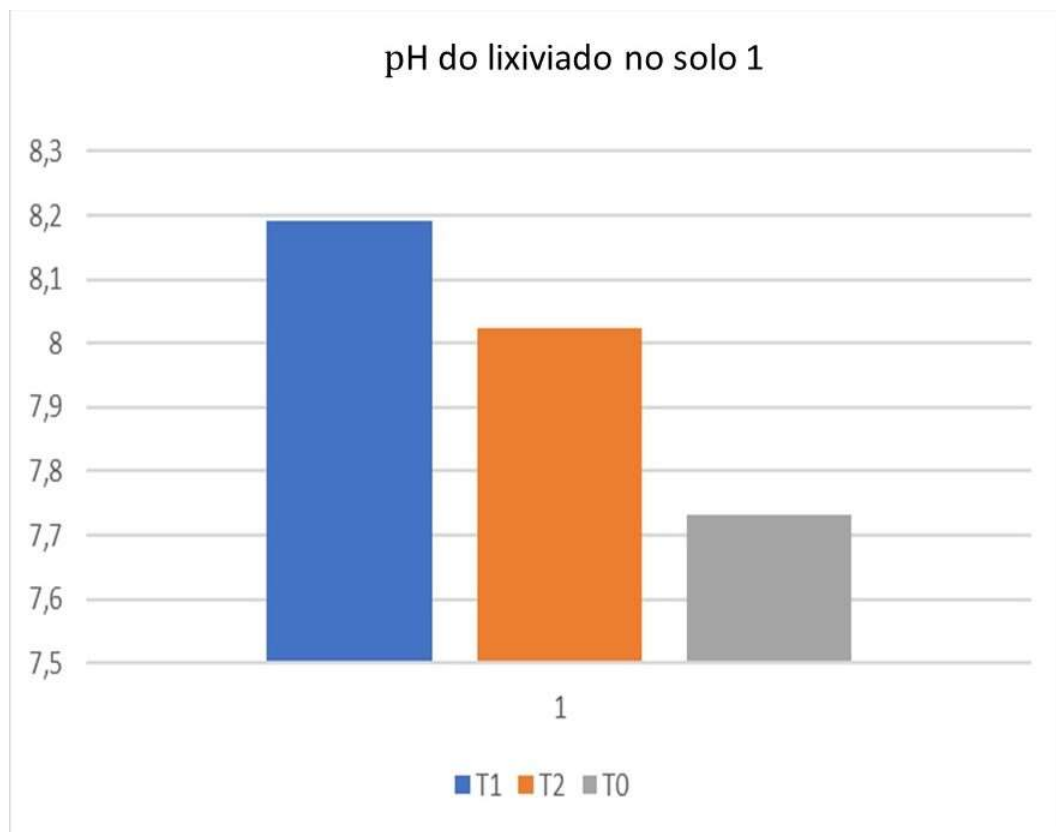
Gráfico 2- pH da água lixiviada no solo 1
