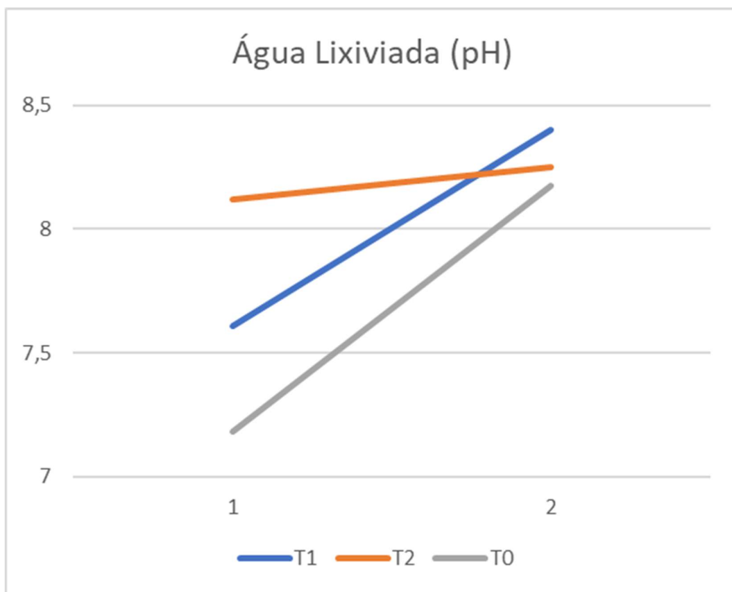
Gráfico 6– pH da água lixiviada Solo 3
