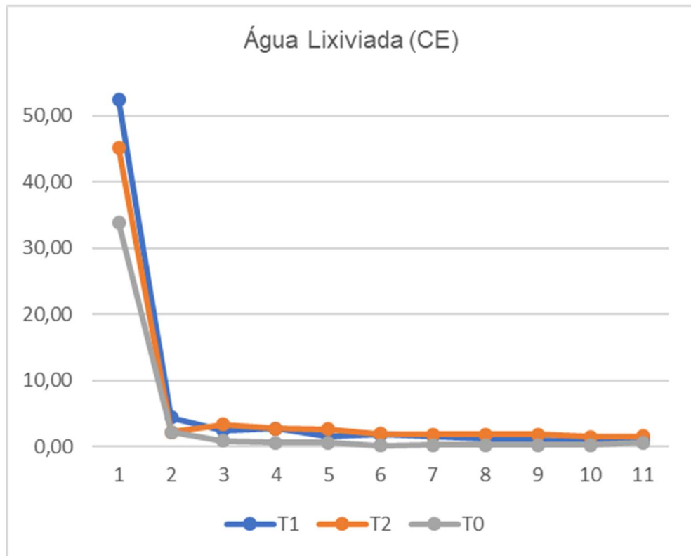
Gráfico 7- Condutividade elétrica da água lixiviada no Solo 4
