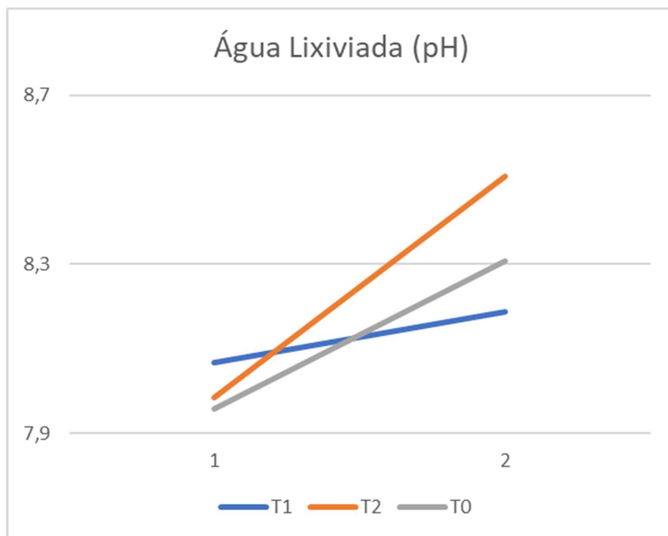
Gráfico 4 – pH da água lixiviada no solo 2
