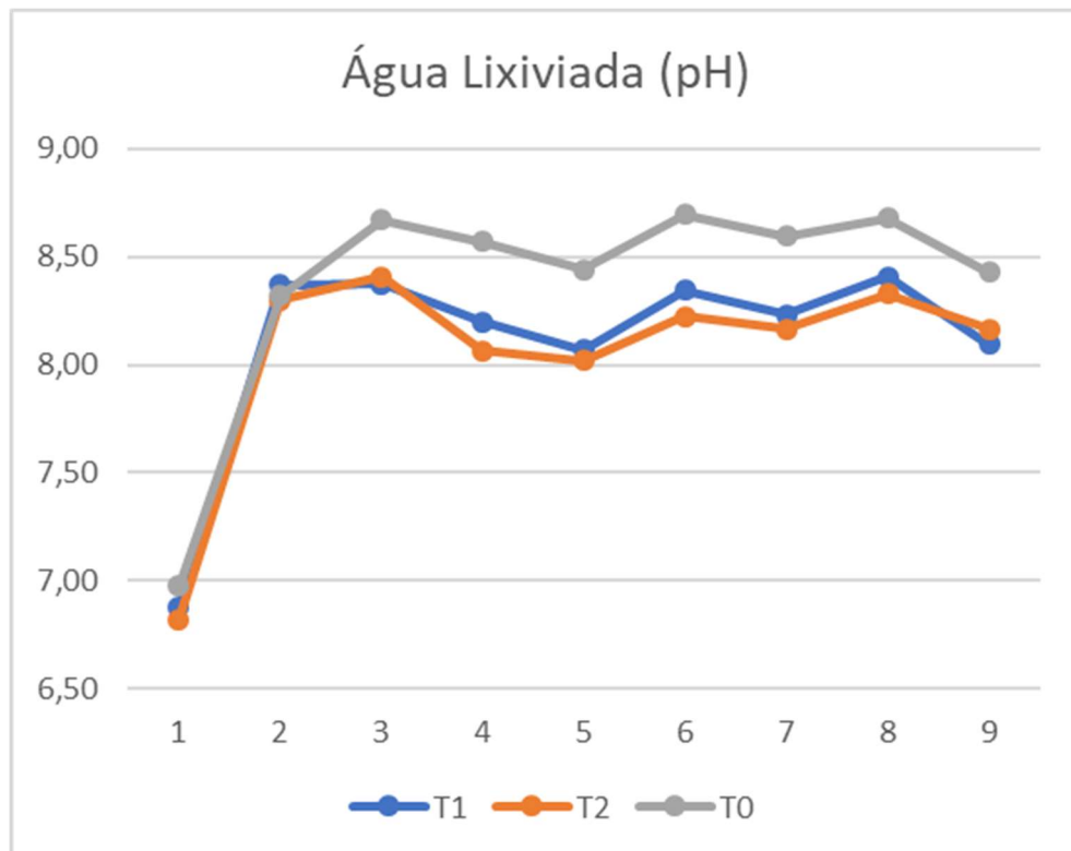
Gráfico 12 - Solo 6 – pH da água lixiviada
