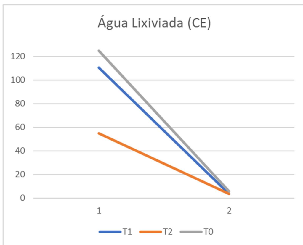
Gráfico 5– Condutividade da água lixiviada do Solo 3
