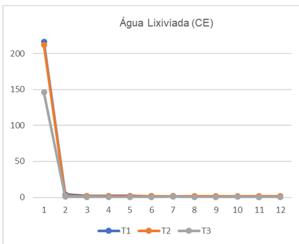
Gráfico 9– Condutividade da água lixiviada do Solo 5
