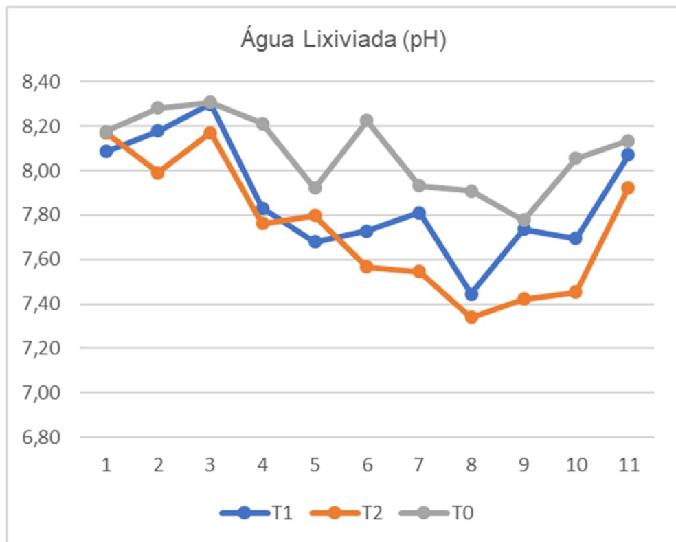
Gráfico 8- pH da água lixiviada no Solo 4
