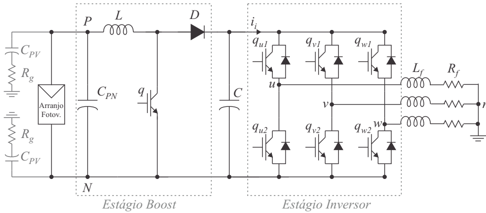
Figura 4 – Conversor de dois estágios para sistemas FV sem transformador.
