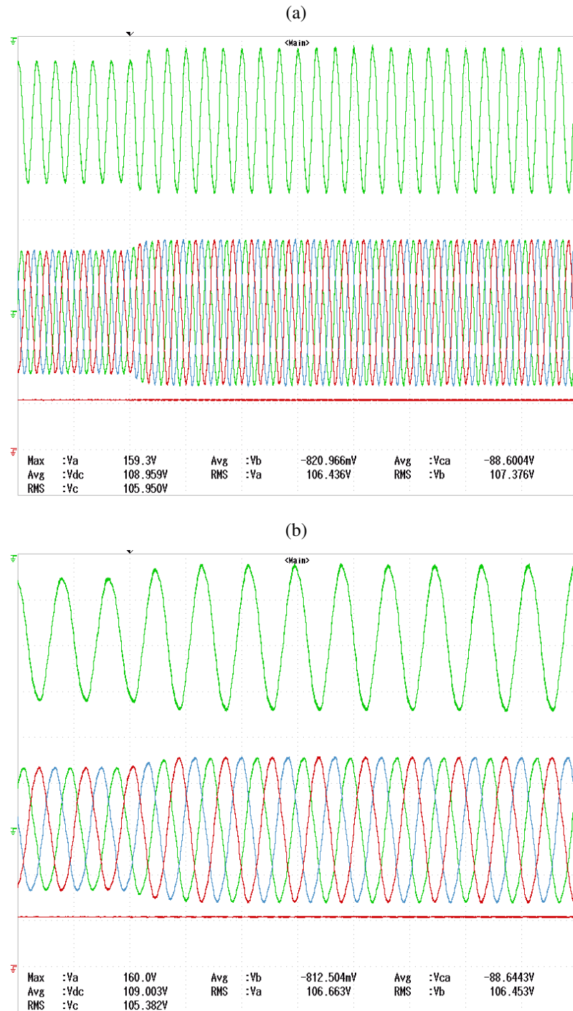
Figura 102 – Inversor buck-boost sete chaves com controle. Degrau de +15% em V_o^{ref} (de 132 V para 155,4 V): (Verde) V_{cA} (50 V/div); (Colorido) v_{oABC} (100 V/div); (Vermelho) V_{in} (200 V/div). (a) 50 ms/div (b) 20 ms/div
