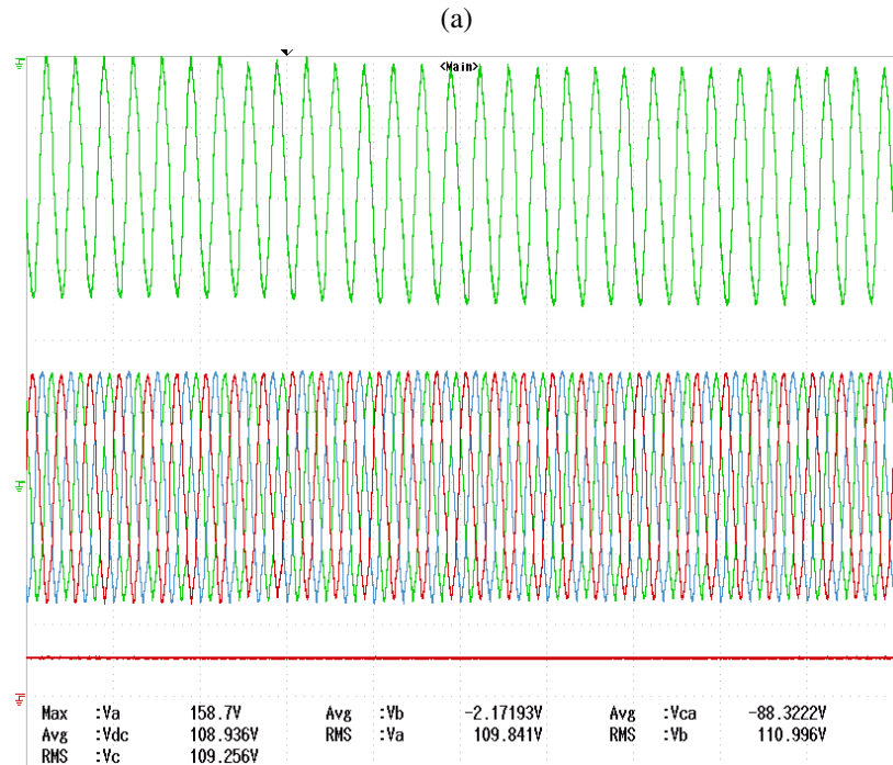
Figura 99 – Inversor buck-boost nove chaves com controle. (a) Degrau de +5% em V_{bb}^{ref} (de -168,1 V para -177 V) (b) Degrau de -5% em V_{bb}^{ref} (de -177 V para -168,1 V): (Verde) V_{cA} (50 V/div); (Colorido) v_{oABC} (100 V/div); (Vermelho) V_{in} (200 V/div). 50 ms/div
