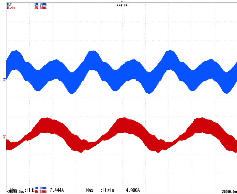
Figura 93 – Inversor buck-boost com nove chaves com carga resistiva e sem controle - Correntes nos indutores, valores máximos, ( i_L=4,9\text{ A} e i_{Lf}=7,44\text{ A} ). Escala de 5\text{ A/div} .
