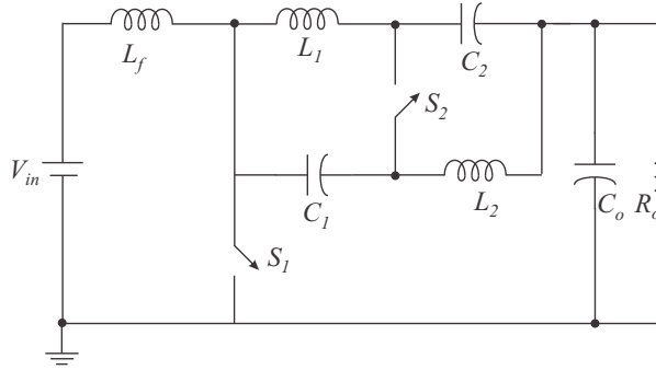
Figura 13 – Topologia proposta em (BERKOVICH et al., 2007) com característica bidirecional de quatro quadrantes.
