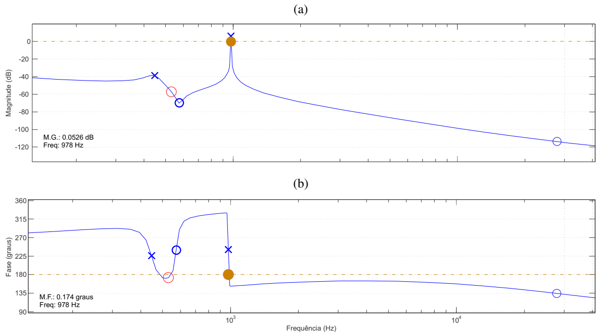
Figura 56 – Digrama de Bode de \hat{v}_{bb}/\hat{d}_1 em malha aberta ( V_o=220 V_{rms} ) - (a) Magnitude (b) Fase.
