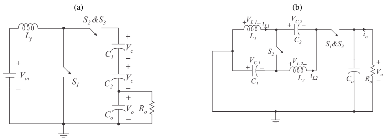
Figura 22 – Representação esquemática da topologia da Figura 21 em: (a) estágio boost e (b) estágio semi-ZSI .
