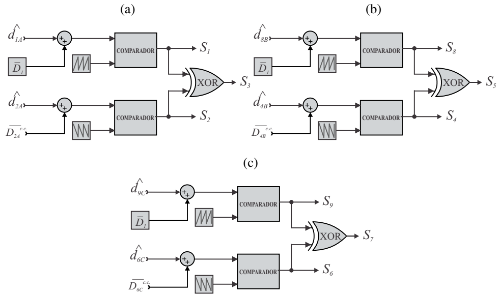
Figura 72 – Diagrama de blocos para obtenção dos sinais de gatilho das chaves S_1 a S_9 , considerando a compensação da componente c.c. de v_o .
