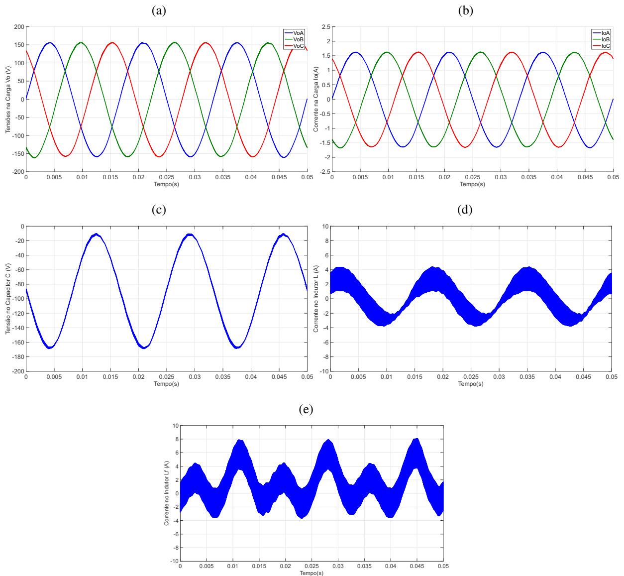
Figura 73 – Inversor buck-boost com nove chaves e controle: (a,b) tensões e correntes na carga; (c) tensão no capacitor C ; (d,e) correntes nos indutores L e L_f .
