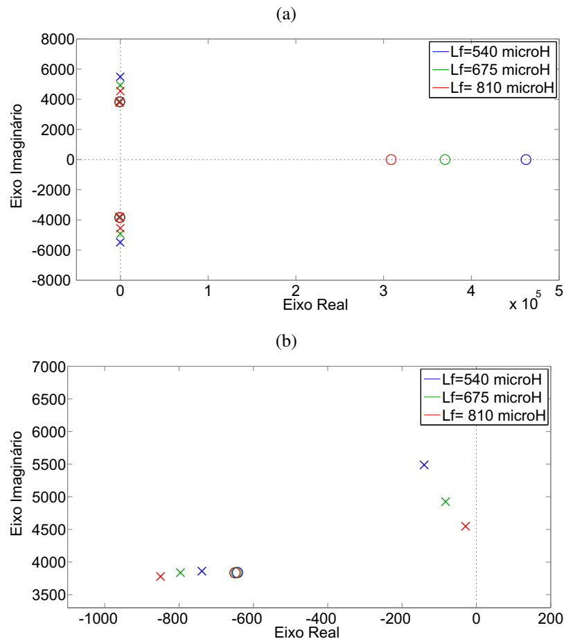
Figura 50 – (a) Lugar das raízes com variação de L_f ; (b) Ampliação para visualização dos polos.
