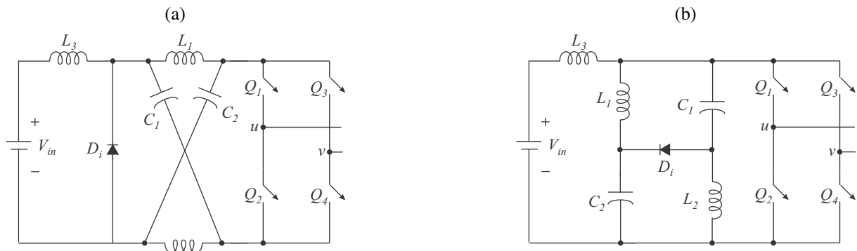
Figura 9 – Exemplos de topologias quasi-ZSI (qZSI).
