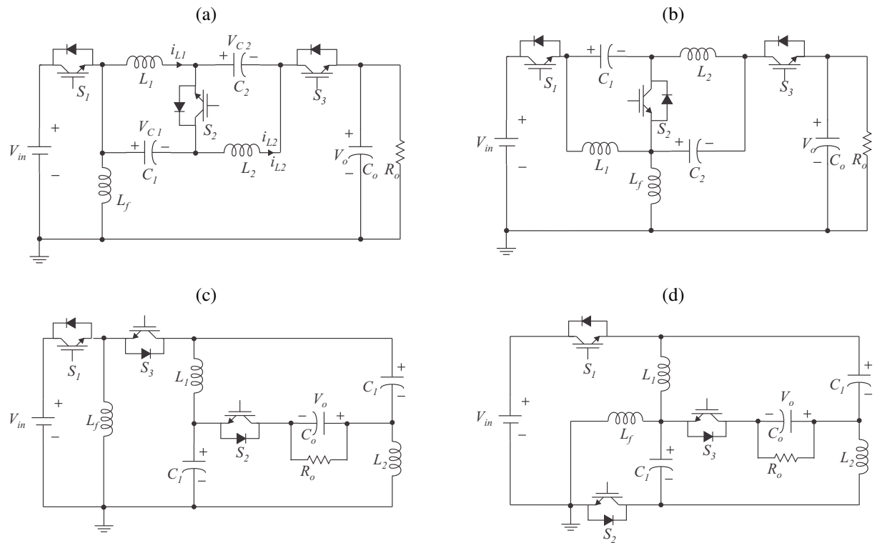
Figura 7 – Família TSTS-ZSIs com entrada do tipo buck-boost propostas em (HUANG et al., 2013).
