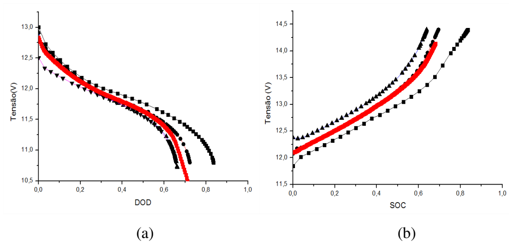
Figura 16 – Tensão em baterias de 12V: Tensão x SOC (a) e Tensão x DOD (b).
