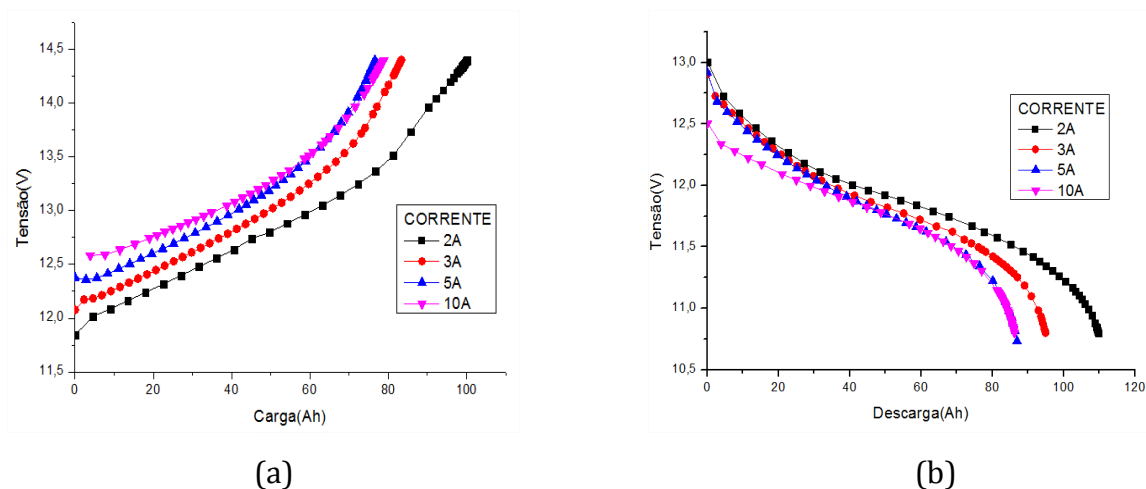
Figura 15 – Ensaio em baterias de 12V de 120Ah para carregamento (a) e descarregamento (b).
